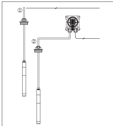
插图 5: 将 VEGAWELL S 51 与供电装置相连接
