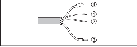
插图. 6: 悬挂电缆接线说明
