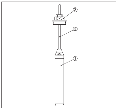
插图. 1: 示例：一个采用螺纹连接的 VEGAWELL S 51
