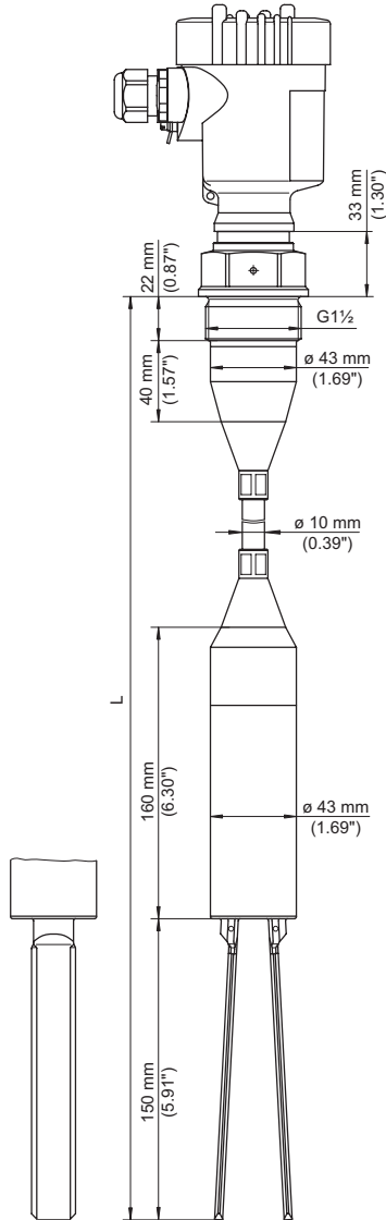
插图. 19: VEGAWAVE 62 带有 FEP 悬挂缆，螺纹型 G1½ (DIN ISO 228/1)
