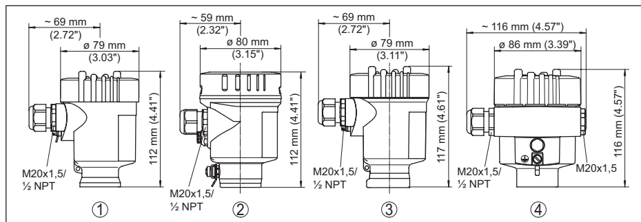
插图. 16: 外壳型的保护等级为 IP66/IP67 和 IP66/IP68; 0.2 bar
