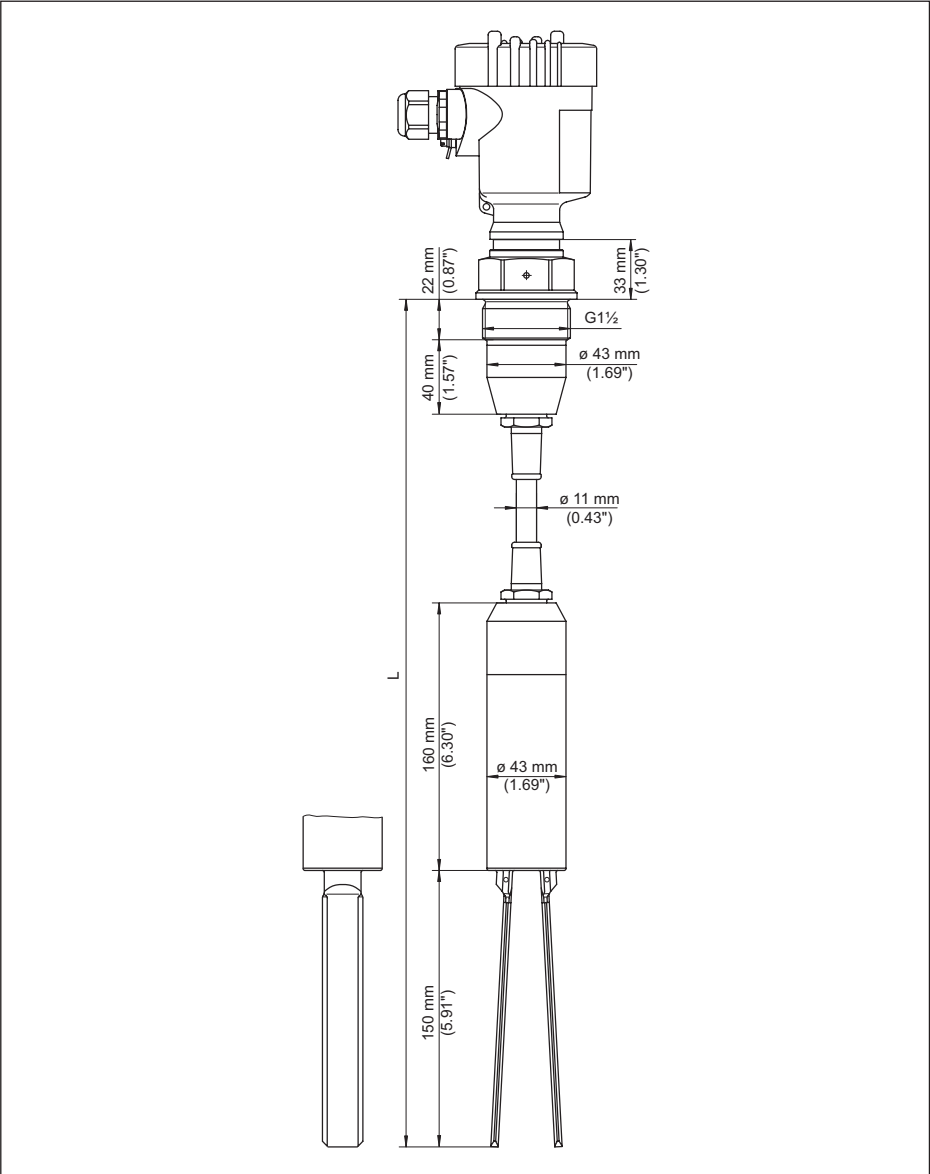
插图. 18: VEGAWAVE 62 带有 PUR 悬挂缆, 螺纹型 G1½ (DIN ISO 228/1)
