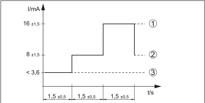
插图. 13: 功能测试的过程图 (运行模式 "最大")
