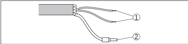
插图. 11: 连接电缆的芯线分布
