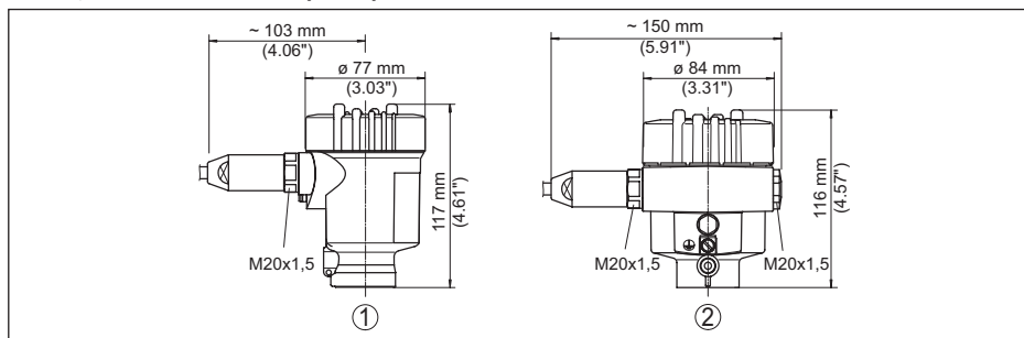
插图. 16: 外壳型的保护等级为 IP66/IP68 (1 bar)
