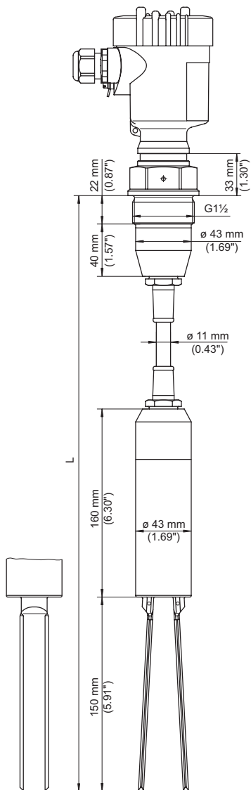
插图. 17: VEGAWAVE 62 带有 PUR 悬挂缆, 螺纹型 G1½ (DIN ISO 228/1)
