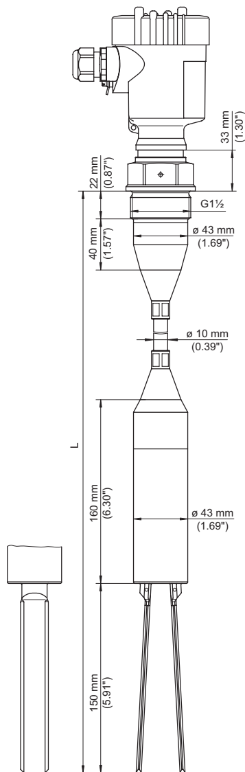
插图. 18: VEGAWAVE 62 带有 FEP 悬挂缆，螺纹型 G1½ (DIN ISO 228/1)
