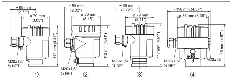
插图. 15: 外壳型的保护等级为 IP66/IP67 和 IP66/IP68; 0.2 bar
