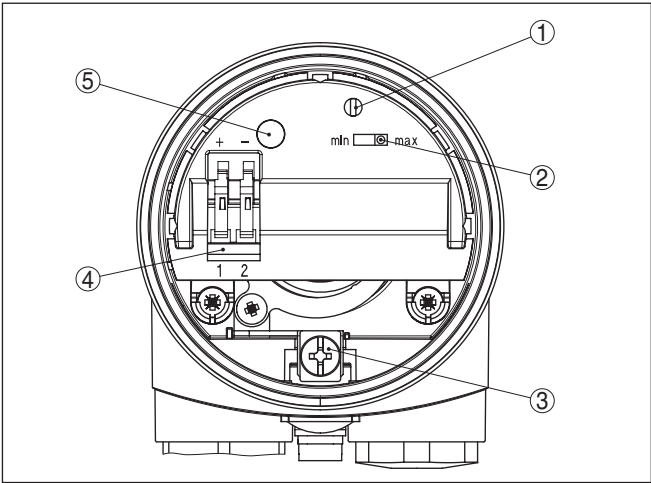
插图. 12: 电子部件腔和接线腔 - 两线制输出口
