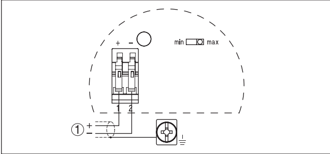
插图. 10: 接线图
