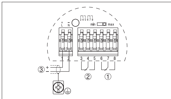
插图. 10: 接线图
