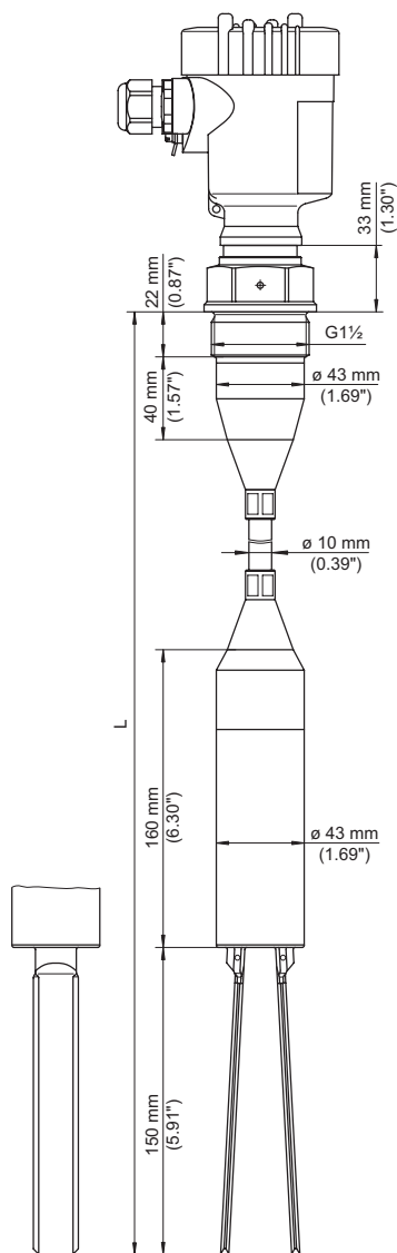
插图. 15: VEGAWAVE 62 带有 FEP 悬挂缆，螺纹型 G1½ (DIN ISO 228/1)
