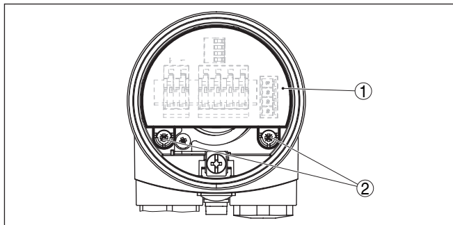
插图. 12: 拧松支撑螺钉
