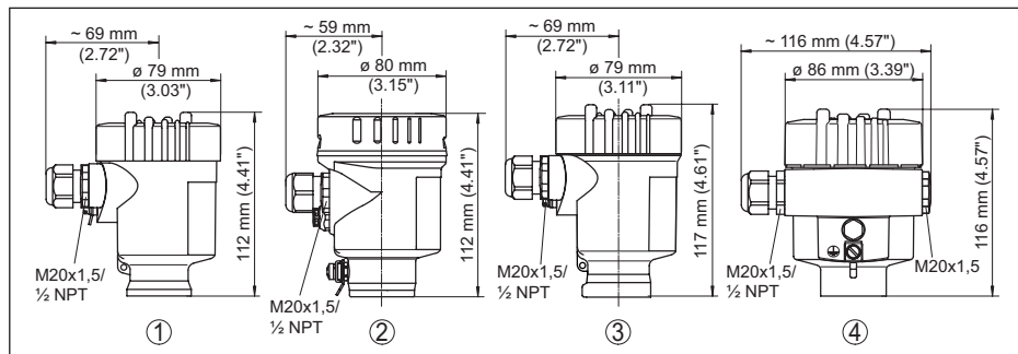
插图. 15: 外壳选型
