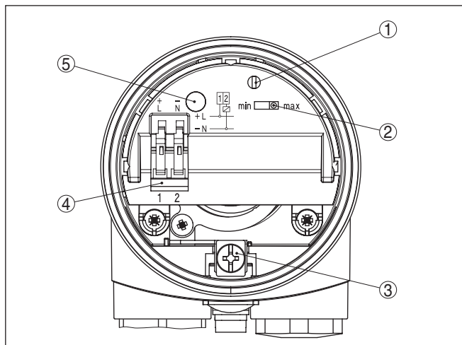
插图. 11: 电子部件腔和接线腔 - 无接触式开关
