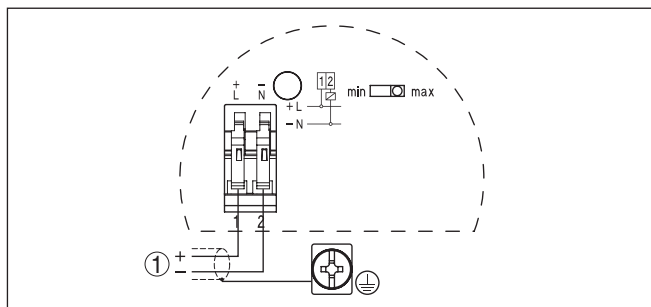
插图. 10: 接线图
