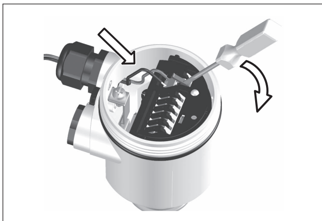
插图. 7: 接线步骤5和6
