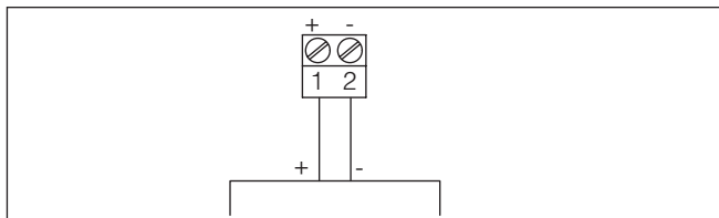
插图. 9: 单腔式外壳的接线图
