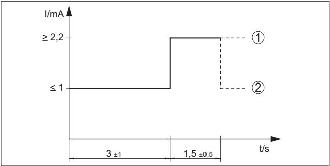
插图. 13: 功能测试的过程图 - 开关功能符合覆盖状态 and 所选的特性曲线 (参见功能表) 1 High Current 2 Low Current
