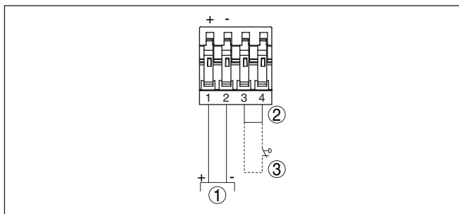
插图. 10: 接线图 - 外部模拟按钮
