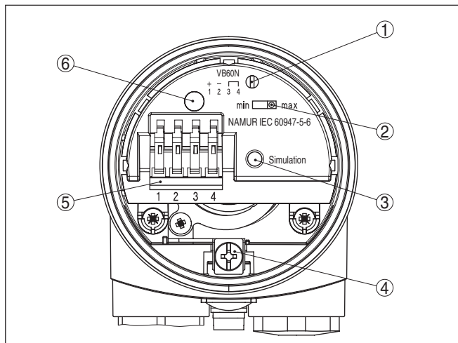
插图. 12: 电子部件腔和接线腔 - NAMUR 输出口
