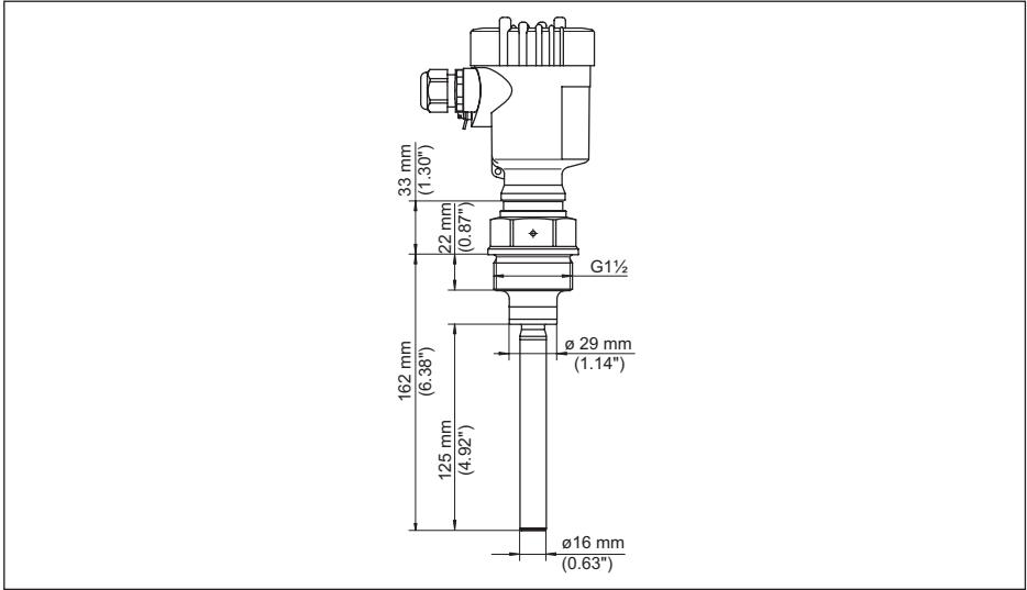
插图. 21: VEGAVIB 61，螺纹型 G1½ (DIN ISO 228/1)
