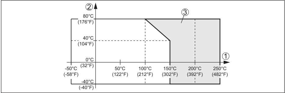
插图. 17: 环境温度 - 过程温度
