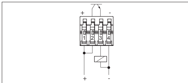
插图. 12: PNP 工作方式
