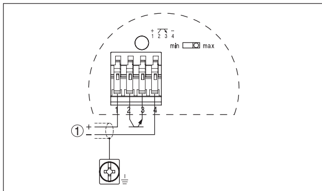
插图. 10: 接线图
