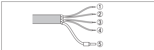
插图. 13: 连接电缆的芯线分布情况。芯线的编号对应于仪表的接线端子。
