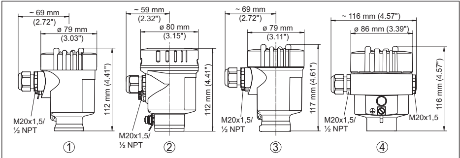
插图. 18: 外壳型的保护等级为 IP66/IP67 和 IP66/IP68; 0.2 bar
