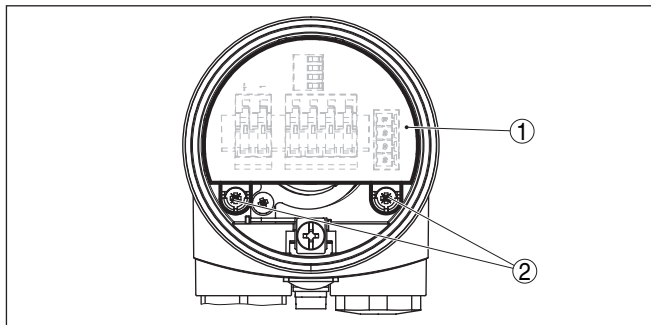
插图. 15: 拧松支撑螺钉
