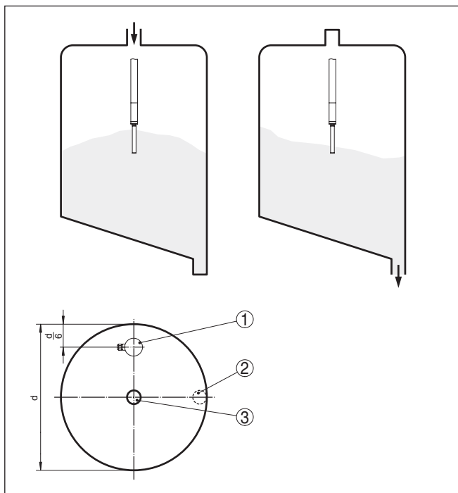
插图. 5: 在中央充填，在侧面排空
