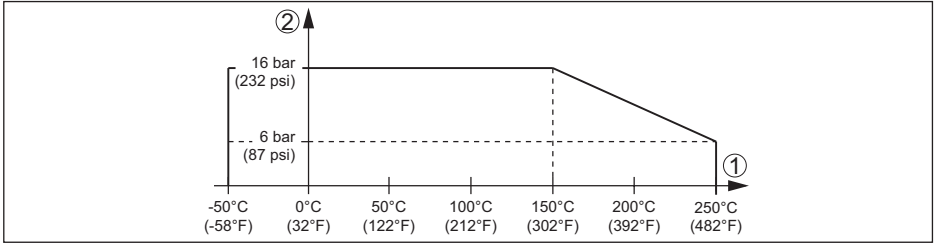
插图. 16: 过程压力 - 过程温度
