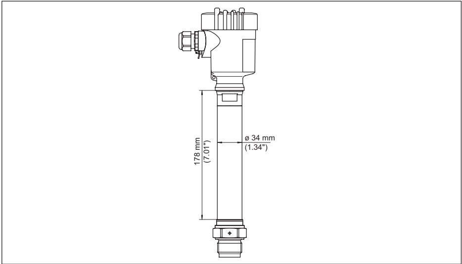
插图. 22: 温度连接元件
