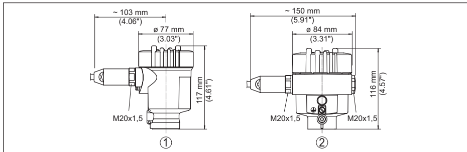
插图. 19: 外壳型的保护等级为 IP66/IP68 (1 bar)
