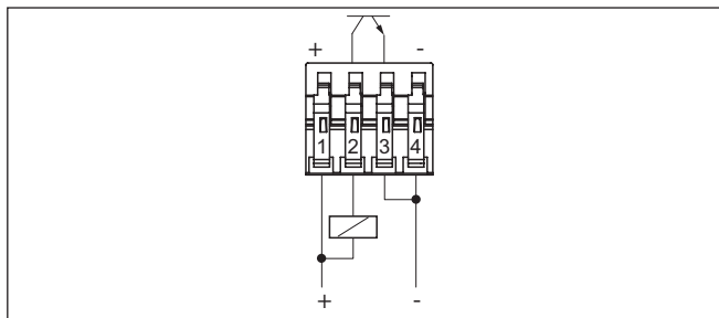
插图. 11: NPN 工作方式
