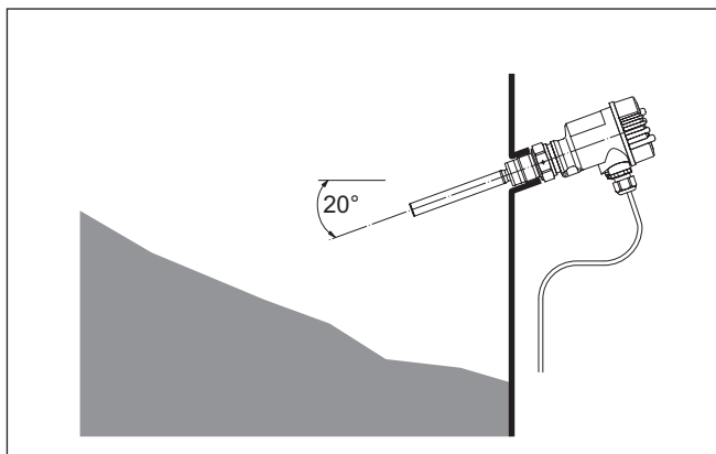
插图. 6: 水平式安装
