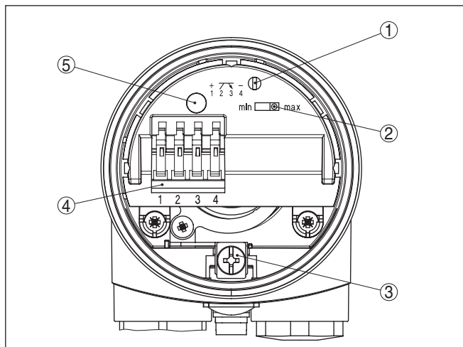
插图. 14: 电子部件腔和接线腔 - 晶体管输出口
