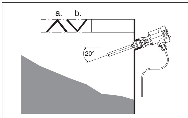
插图. 3: 水平安装
