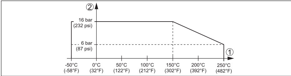
插图. 13: 过程压力 - 过程温度
