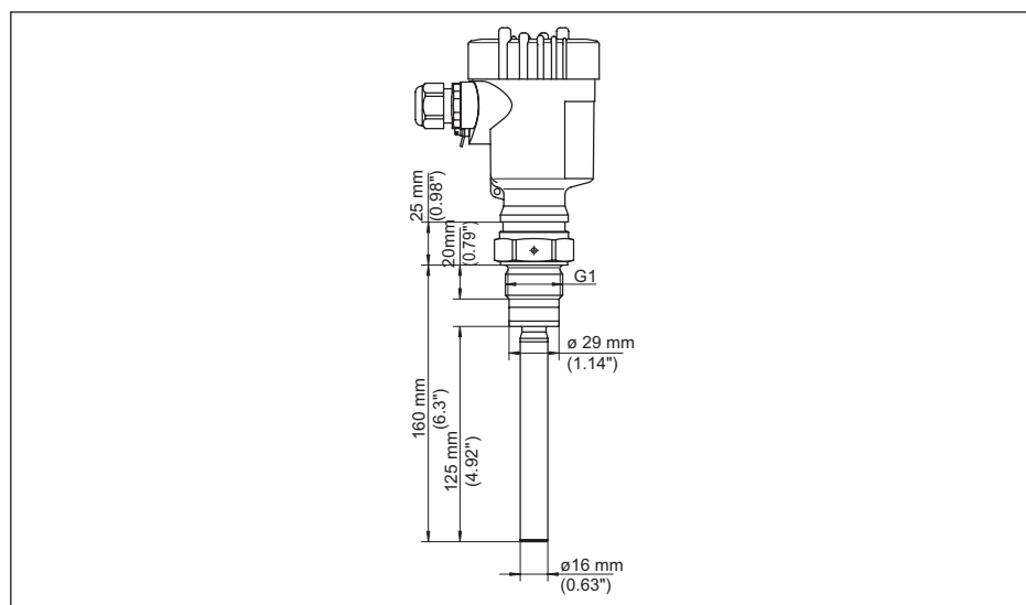
插图. 16: VEGAIB 61，螺纹型 G1 (DIN ISO 228/1)
