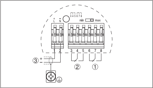
插图. 10: 接线图
