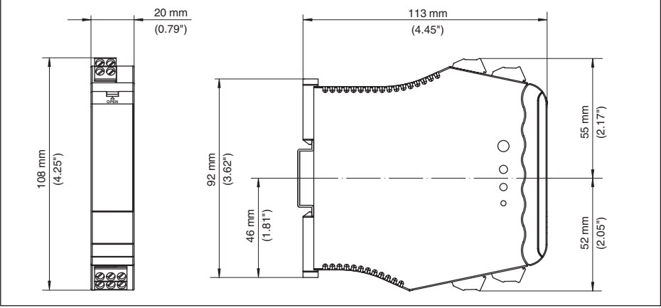
插图 2: VEGATRENN 152 的尺寸
