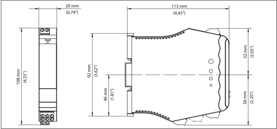
插图. 4: VEGATOR 111 的尺寸
