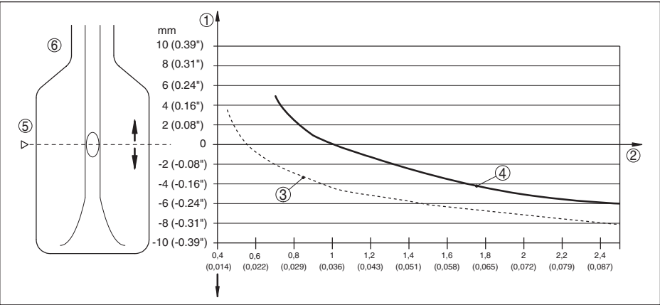
插图. 14: 介质密度对开关点的影响
