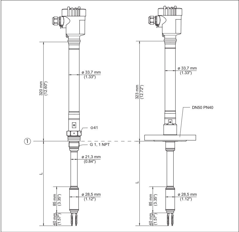
插图. 22: VEGASWING 66, 管型
