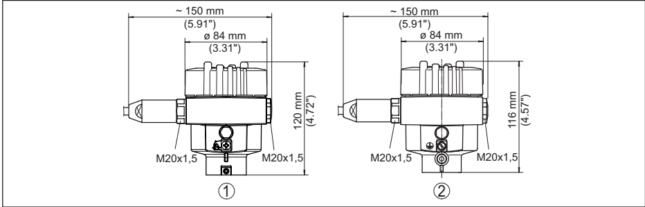
插图. 20: 外壳型的保护等级为 IP66/IP68 (1 bar)
