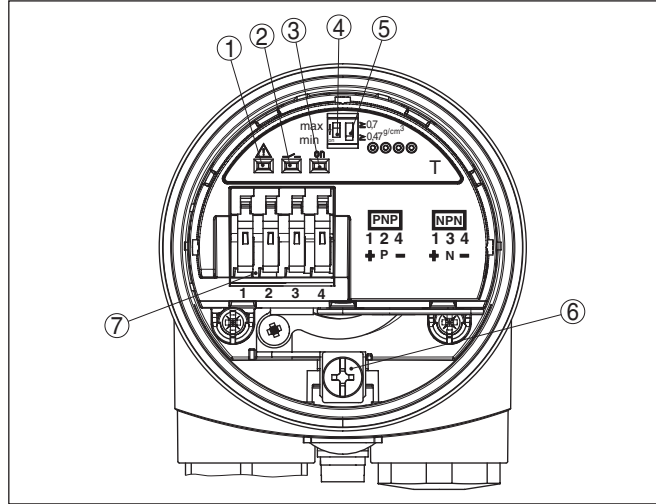
插图. 11: 电子部件和接线腔 单腔式壳体
