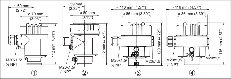
插图. 19: 外壳型的保护等级为 IP66/IP67 和 IP66/IP68 (0.2 bar)
