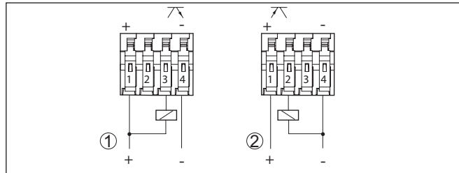
插图. 12: 接线图
