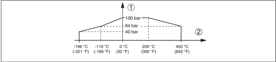
插图. 16: 过程温度 - 过程压力 - 至 100 bar (1450 psig) 的类型
