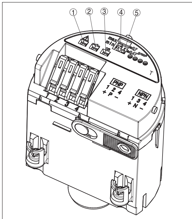
插图. 13: 电子部件 - 晶体管输出口
