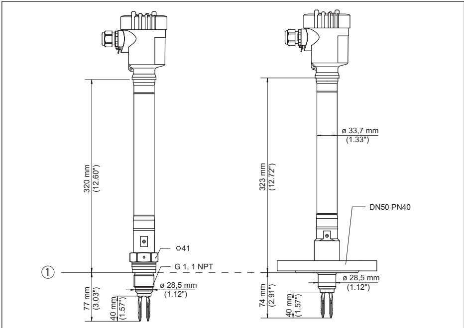
插图. 21: VEGASWING 66, 紧凑型
