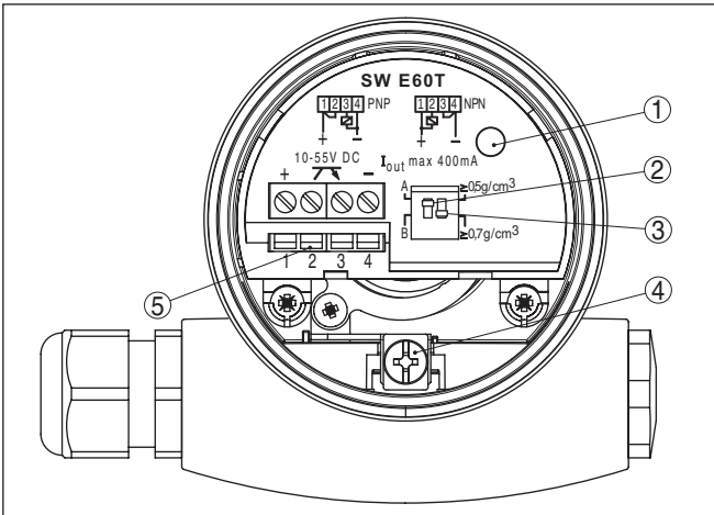
插图. 10: 电子部件和接线腔 单腔式壳体
