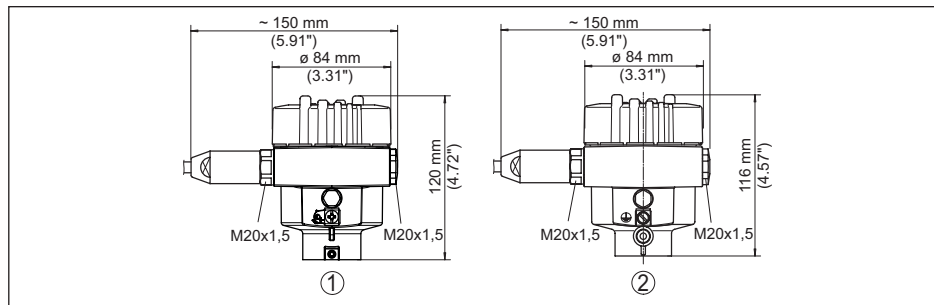
插图. 22: 外壳型的保护等级为 IP66/IP68 (1 bar)
