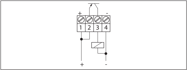
插图. 12: PNP 工作方式
