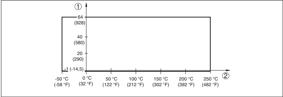
插图. 19: 过程温度 - 开关位置 \geq 0.7 \text{ g/cm}^3 时的过程压力 (灵敏度转换开关)
