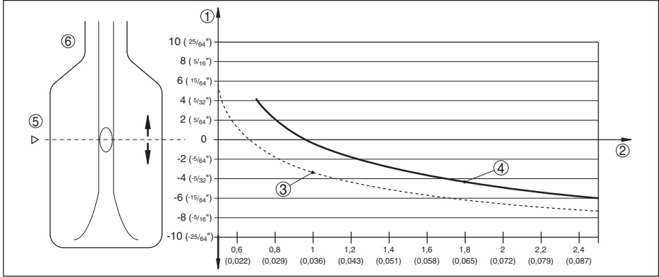
插图. 16: 介质密度对开关点的影响
