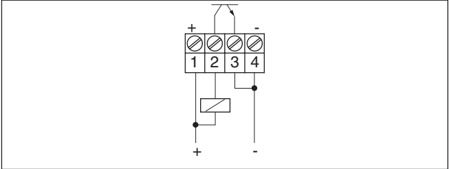
插图. 11: NPN 工作方式
