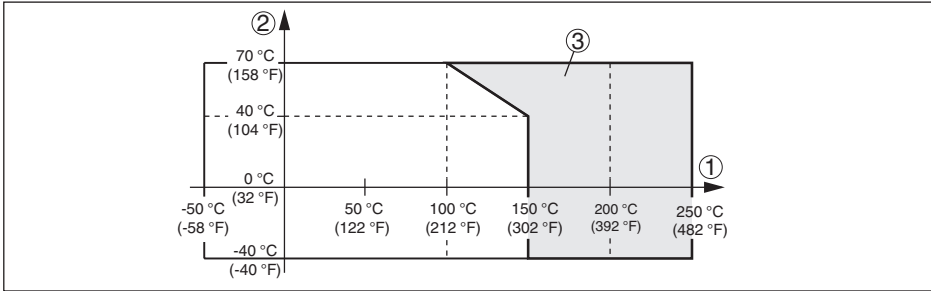
插图. 18: 环境温度 - 过程温度
