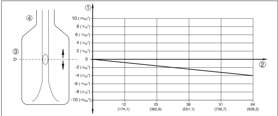
插图. 17: 过程压力对开关点的影响
