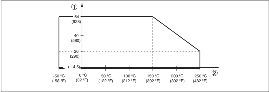
插图. 20: 过程温度 - 开关位置 \geq 0.5 \text{ g/cm}^3 时的过程压力 (灵敏度转换开关)
