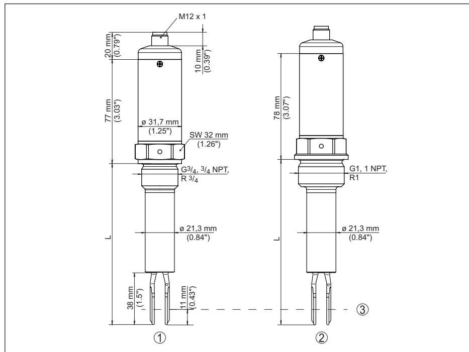
插图. 14: VEGASWING 53, 高温型, 螺纹接头
