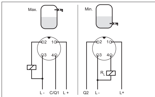
插图. 9: 接线图 (壳体), IO-Link 输出的端子占用情况, 带 M12 x 1 插头
