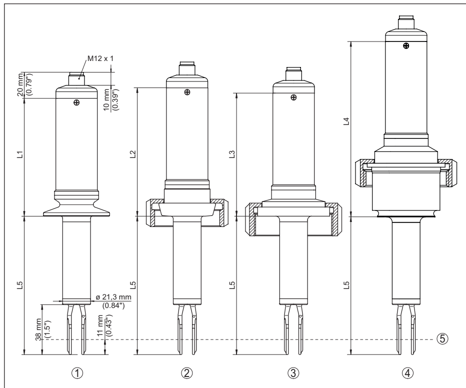
插图. 15: VEGASWING 53, 食品型, 卫生型接头
