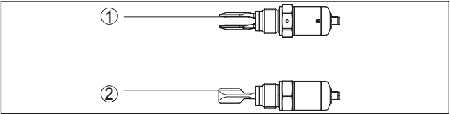
插图. 3: 水平安装 1 开关打开位置 2 开关点 (推荐的安装位置, 主要针对附着性介质)
