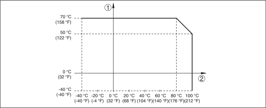
插图. 11: 环境温度与过程温度的相关性
