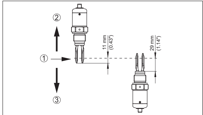
插图. 2: 垂直安装
