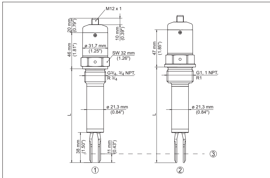
插图. 13: VEGASWING 53, 标准型, 螺纹接头
