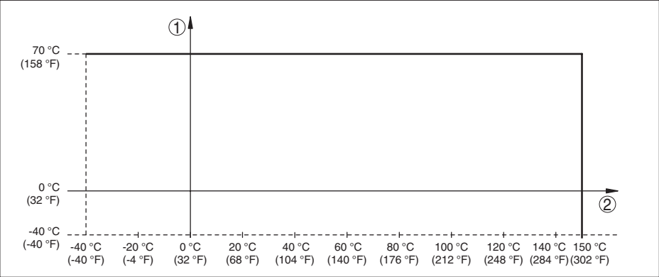
插图. 12: 环境温度与过程温度的相关性
