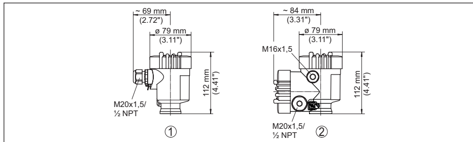
插图 35: 采用防护等级为 IP66/IP67 的外壳版本 (内装显示和调整模块后，外壳高度增加了 9 mm/0.35 in)
