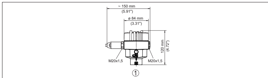
插图. 39: 采用防护等级达 IP66/IP68 (1 bar) 的壳体版本 (内装显示和调整模块后, 壳体高度增加了18 mm/0.71 in)
