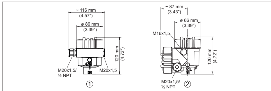
插图 36: 采用防护等级达 IP66/IP68 (0.2 bar) 的壳体版本，(内装显示和调整模块后，壳体高度增加了18 mm/0.71 in)
