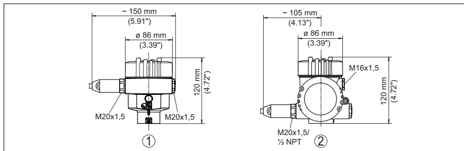
插图. 37: 采用防护等级达 IP66/IP68 (1 bar) 的壳体版本 (内装显示和调整模块后, 壳体高度增加了18 mm/0.71 in)
