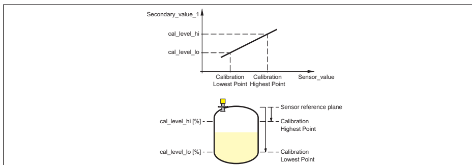
插图. 36: VEGASON 62 的调整
