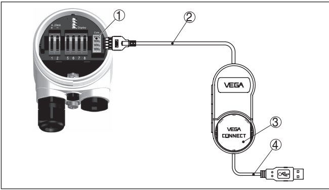
插图. 31: 通过接口适配器 VEGACONNECT 与外部相连
