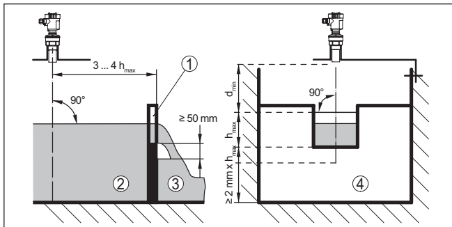
插图. 16: 利用矩形水道来测量流量: d_{\text{最小}} = 传感器的盲区 (参见“技术参数”一章); h_{\text{最大}} = 矩形水道的最大充填量
