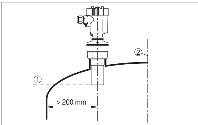
插图. 6: 安装在圆形容器盖上
