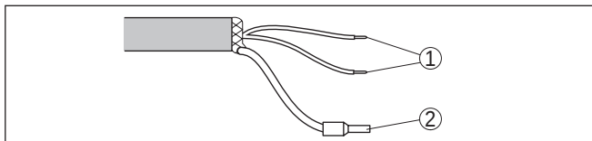
插图. 26: 连接电缆的芯线分布
