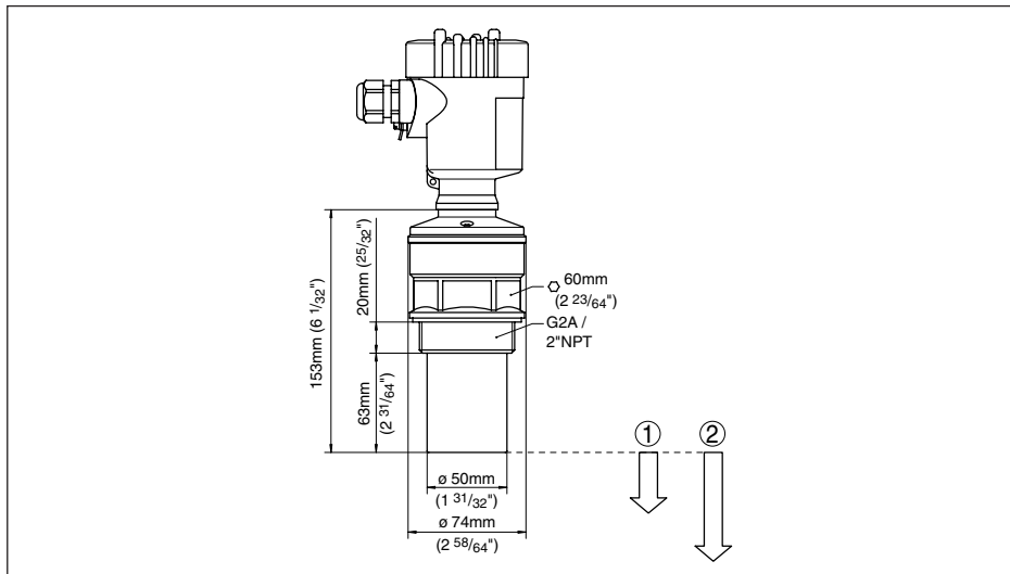
插图. 42: VEGASON 62
