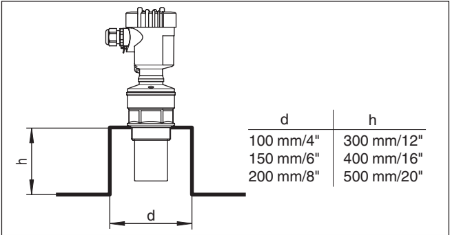
插图. 9: 管接头尺寸有偏差
