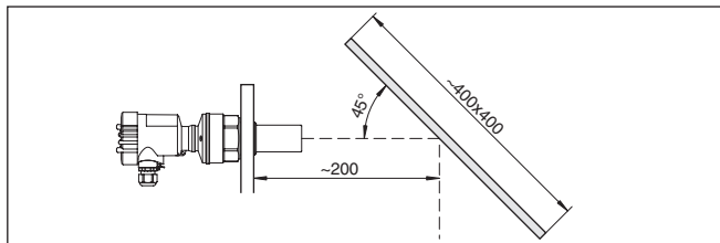
插图. 11: 转向镜
