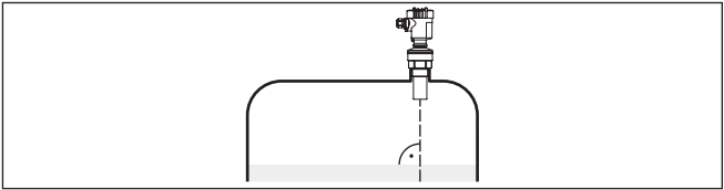
插图. 10: 在液体中校准
