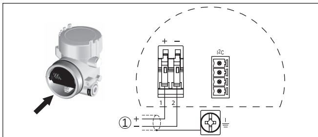
插图. 25: 双腔式外壳的接线图
