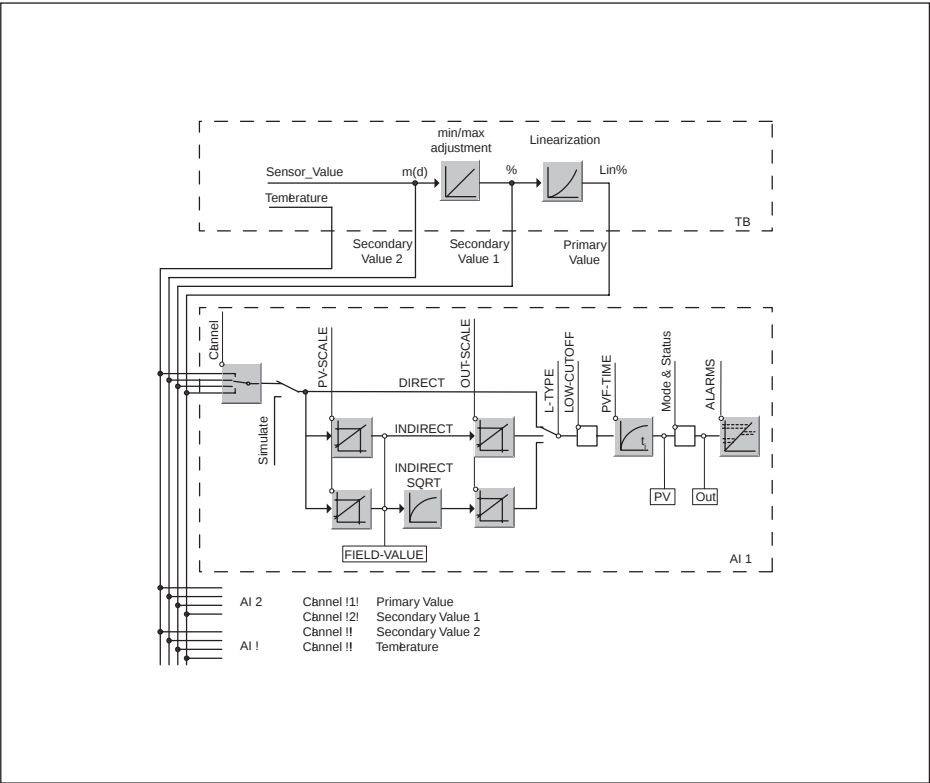
插图. 35: VEGASON 62 的测量值处理
