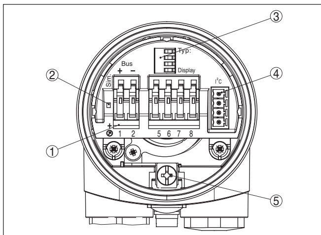
插图. 20: 单腔式外壳的电子部件和接线腔
