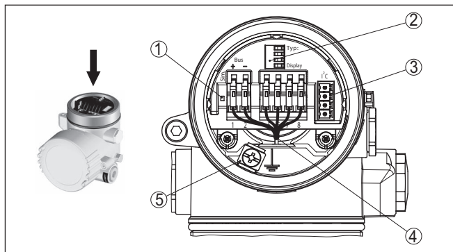
插图. 23: 双腔式外壳的电子部件腔
