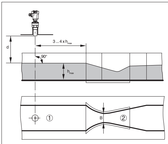
插图. 17: 利用 Khafagi-Venturi 水槽测量流量: d = 传感器的盲区; h_{\text{最大}} = 水槽的最大充填量; B = 水槽的最大面缩率
