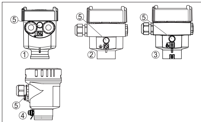
插图. 19: 单腔式外壳所用的各种材料
