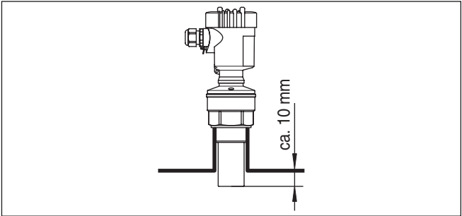
插图. 8: 值得推荐的管接头安装方法
