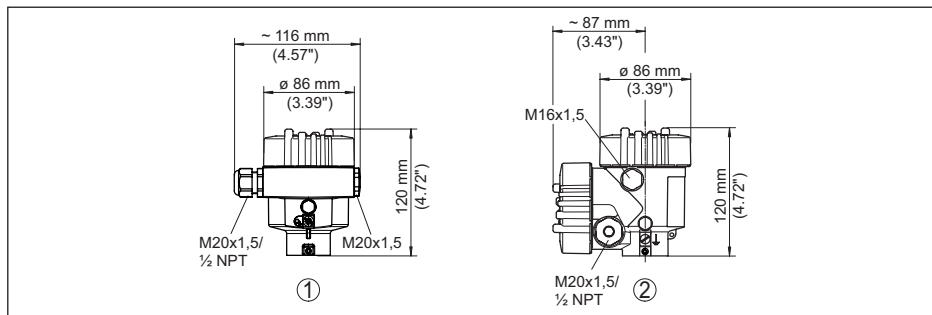
插图. 40: 采用防护等级达 IP66/IP68 (0.2 bar) 的壳体版本, (内装显示和调整模块后, 壳体高度增加了18 mm/0.71 in)
