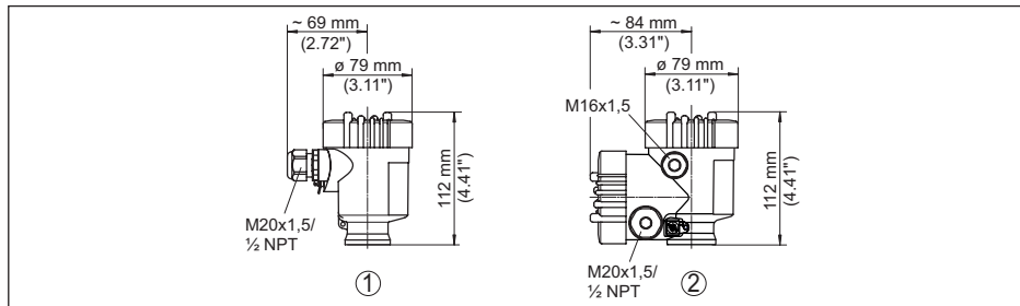
插图. 39: 采用防护等级为 IP66/IP67 的外壳版本 (内装显示和调整模块后, 外壳高度增加了 9 mm/0.35 in)
