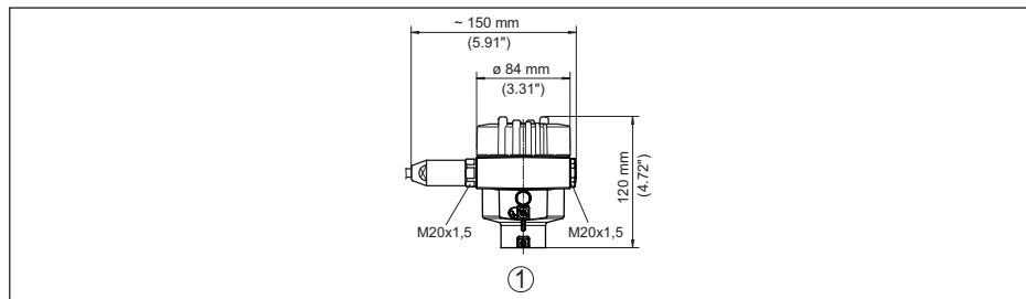
插图. 43: 采用防护等级达 IP66/IP68 (1 bar) 的壳体版本 (内装显示和调整模块后, 壳体高度增加了18 mm/0.71 in)
