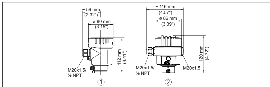
插图. 42: 采用防护等级达 IP66/IP68 (0.2 bar) 的壳体版本, (内装显示和调整模块后, 壳体高度增加了18 mm/0.71 in)
