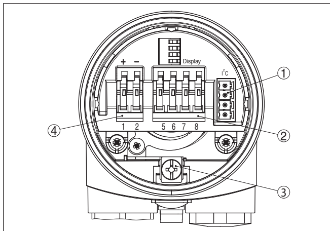
插图. 20: 单腔式外壳的电子部件和接线腔
