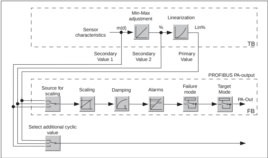
插图 36: VEGASON 61: 带有 AI (PA-OUT) 值和额外的周期值的方块图
