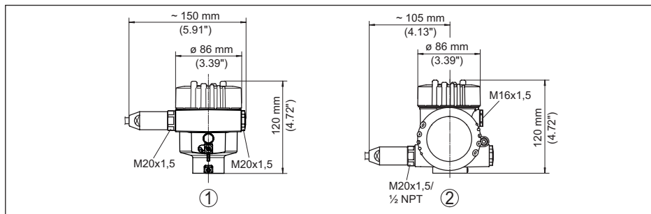
插图. 41: 采用防护等级达 IP66/IP68 (1 bar) 的壳体版本 (内装显示和调整模块后, 壳体高度增加了18 mm/0.71 in)
