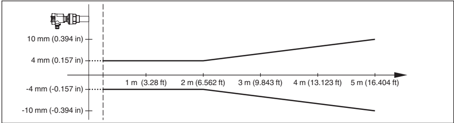
插图. 34: VEGASON 61 的测量偏差
