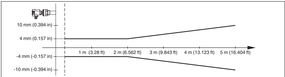
插图. 35: VEGASON 61 的测量偏差
