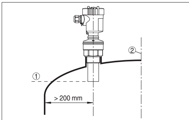
插图. 8: 安装在圆形容器盖上
