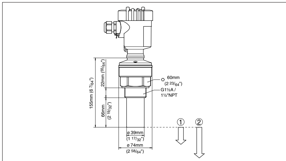
插图. 42: VEGASON 61
