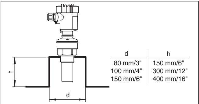
插图. 11: 管接头尺寸有偏差
