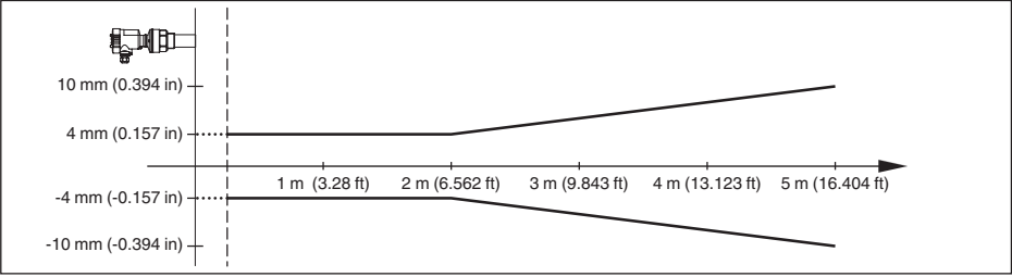
插图. 36: VEGASON 61 的测量偏差
