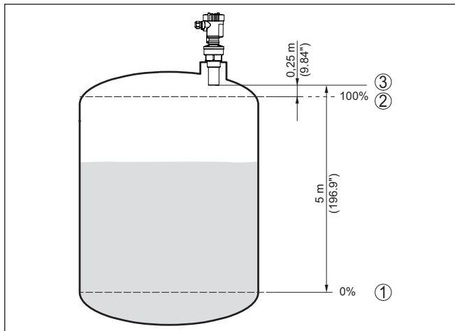
插图. 31: 以最小/最大调整为例说明参数更改情况
