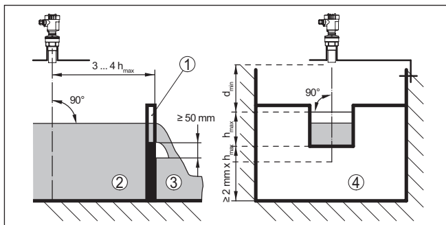
插图. 18: 利用矩形水道来测量流量: d_{\text{最小}} = 传感器的盲区 (参见“技术参数”一章); h_{\text{最大}} = 矩形水道的最大充填量
