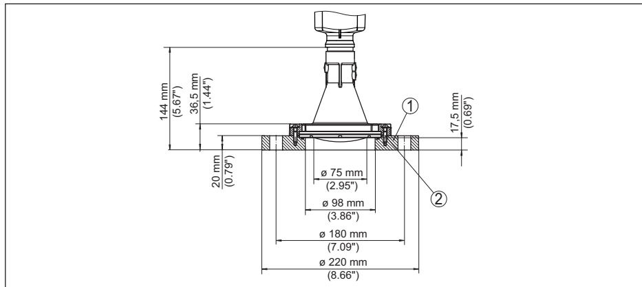
插图 97: VEGAPULS 6X, 带适配法兰 DN 100 PN 6
