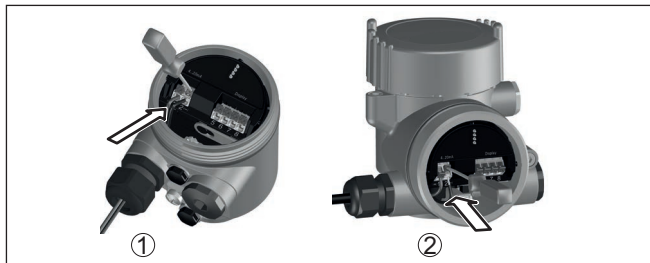
插图. 50: 接线步骤5和6
