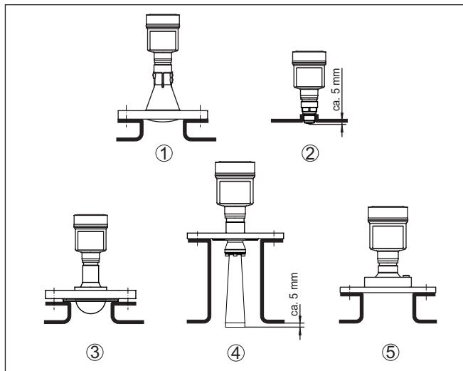
插图. 26: 视型式，安装管接头时的推荐值
