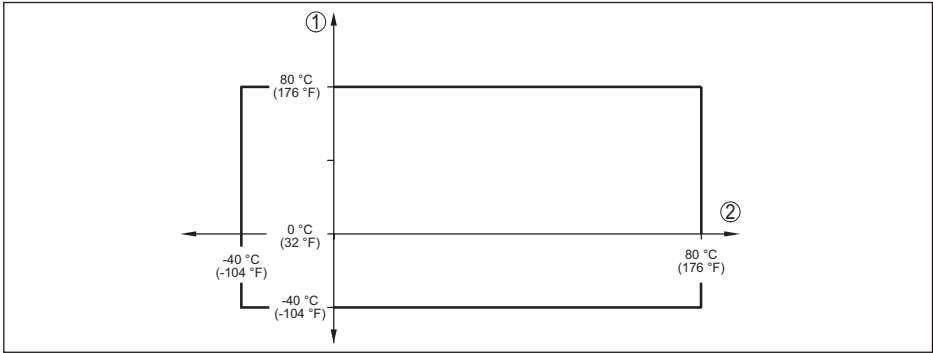
插图. 73: 环境温度降额, 塑料制喇叭口天线
