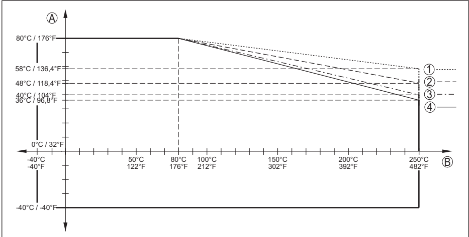
插图. 76: 环境温度降额, 带内置天线系统的螺纹, 至 +250 °C (+482 °F)
