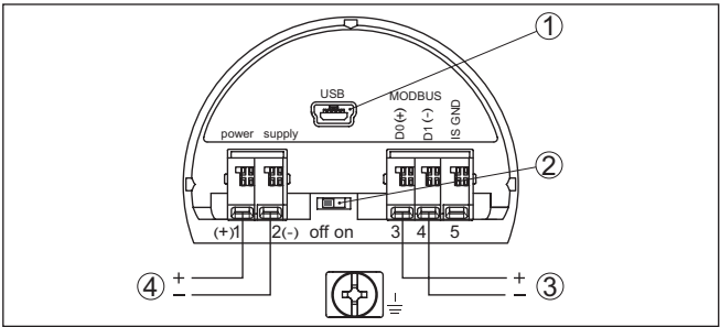
插图. 52: 接线腔
