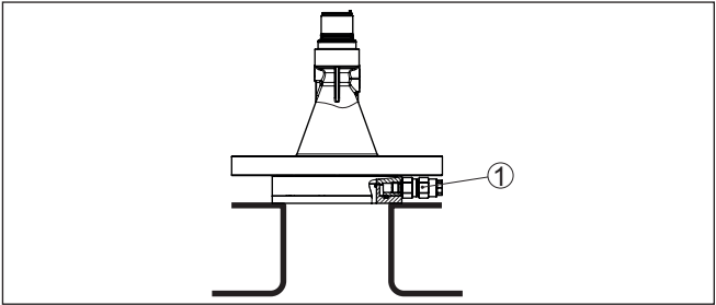
插图. 41: 塑料制喇叭口天线，带锁紧法兰
