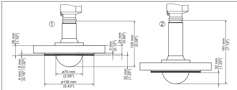
插图. 107: VEGAPULS 6X, 封装天线系统 DN 80 PN 40
