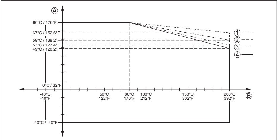
插图. 75: 环境温度降额, 带内置天线系统的螺纹, 至 +200 °C (+392 °F)
