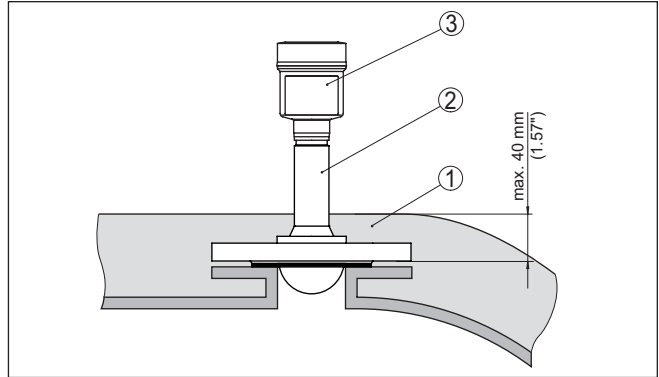
插图. 31: 将仪表安装在绝缘容器上
