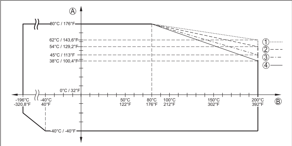
插图. 80: 环境温度降额, 带塑料天线系统的法兰 -196 ... +200 °C (-320.8 ... +392 °F)
