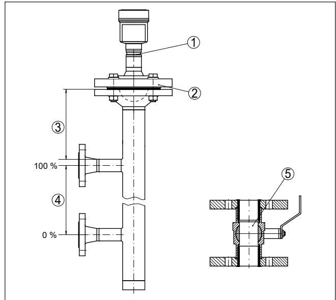
插图. 45: 的构造 - 旁路
