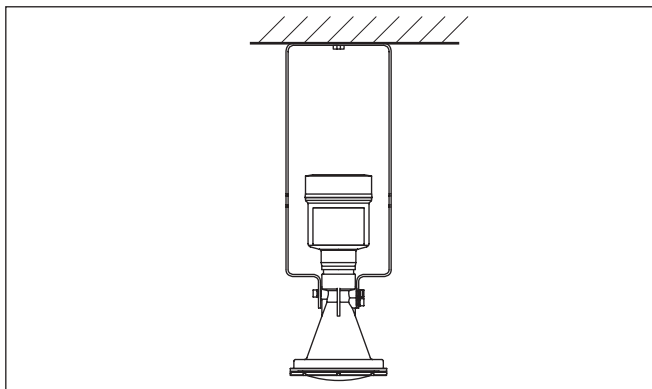
插图. 13: 用长度为 300 毫米的龙门框将仪表安装到天花板上
