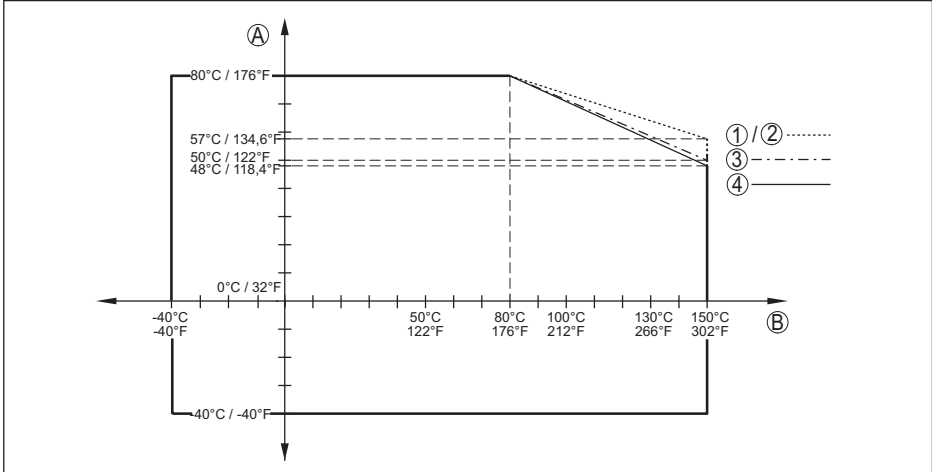
插图. 77: 环境温度降额, 带塑封天线系统的法兰, 至 +150 °C (+302 °F)
