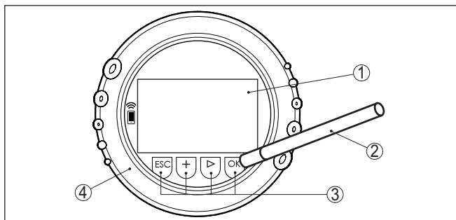
插图. 55: 显示和调整元件 - 拥有磁笔操作功能
