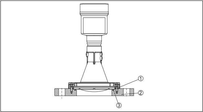
插图. 17: 适配法兰
