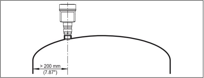
插图. 19: 将雷达仪表安装在圆形容器盖上
