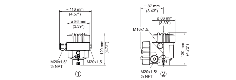
插图 91: 采用防护等级达 IP66/IP68 (0.2 bar) 的壳体版本, (内装显示和调整模块后, 壳体高度增加了18 mm/0.71 in)
