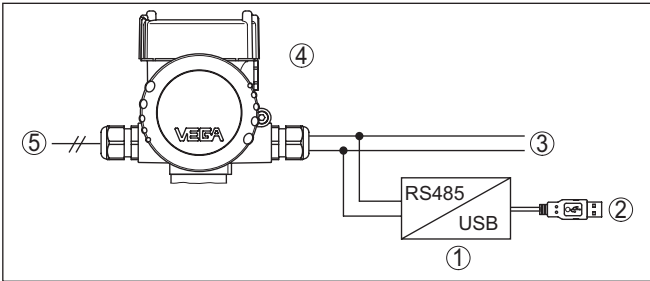
插图. 5: 电脑通过接口适配器与 RS 485 电线相连接
