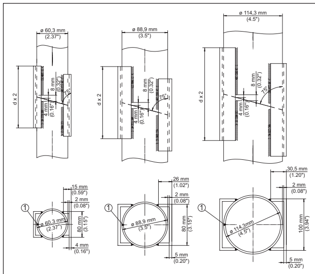
插图. 47: 导波管延长件的焊接连接 (举例)
