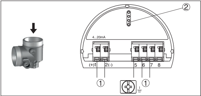
插图. 51: 双腔式外壳的电子部件腔
