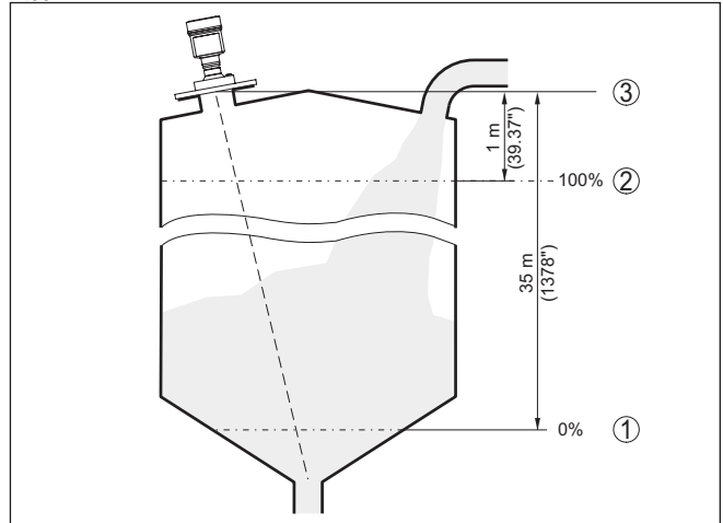
插图. 57: 参数调整举例: 最小/最大调整 - 固料
