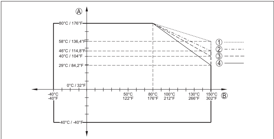
插图. 74: 环境温度降额, 带内置天线系统的螺纹, 至 +150 °C (+302 °F)
