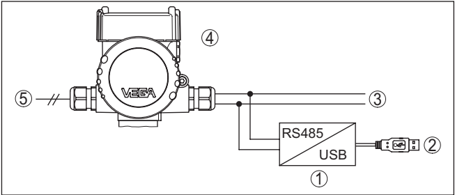
插图. 65: 电脑通过接口适配器与 RS 485 电线相连接
