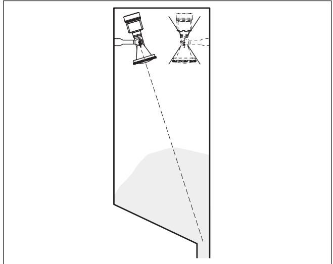
插图. 40: 在多腔式料仓中进行安装和校准
