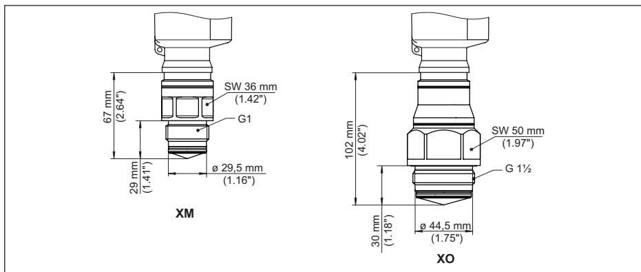
插图. 108: VEGAPULS 6X, 用于卫生型适配器的螺纹
