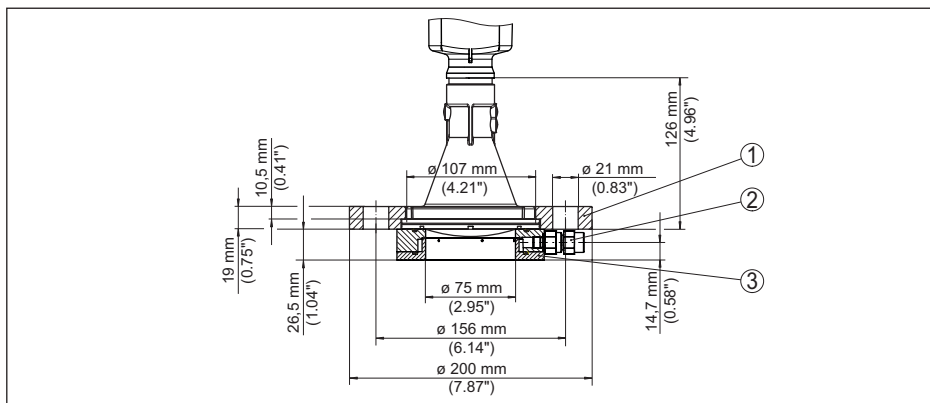
插图. 96: VEGAPULS 6X，带有锁紧法兰和吹气接口，适用于 3" 150 lbs, DN 80 PN 16
