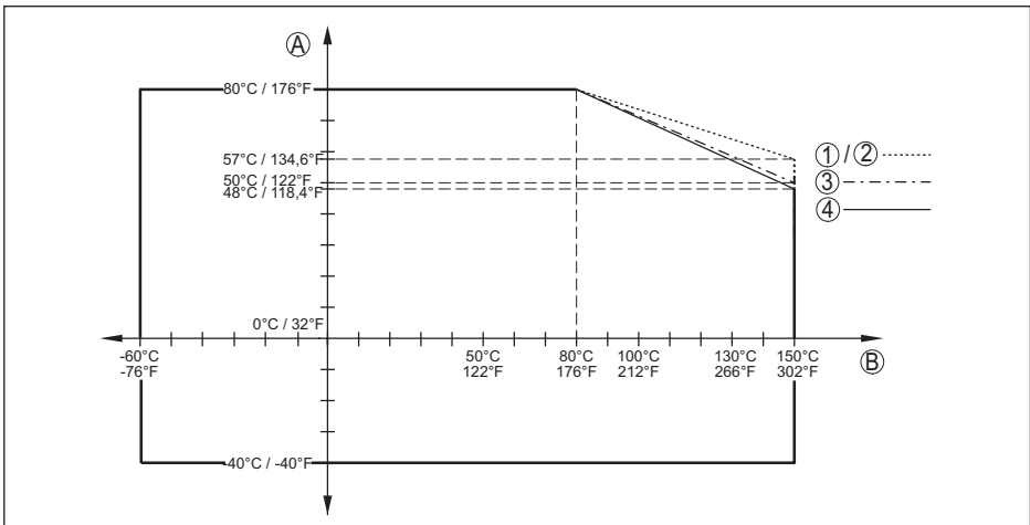
插图. 78: 环境温度降额, 带塑封天线系统的法兰 -60 ... +150 °C (-76 ... +302 °F)
