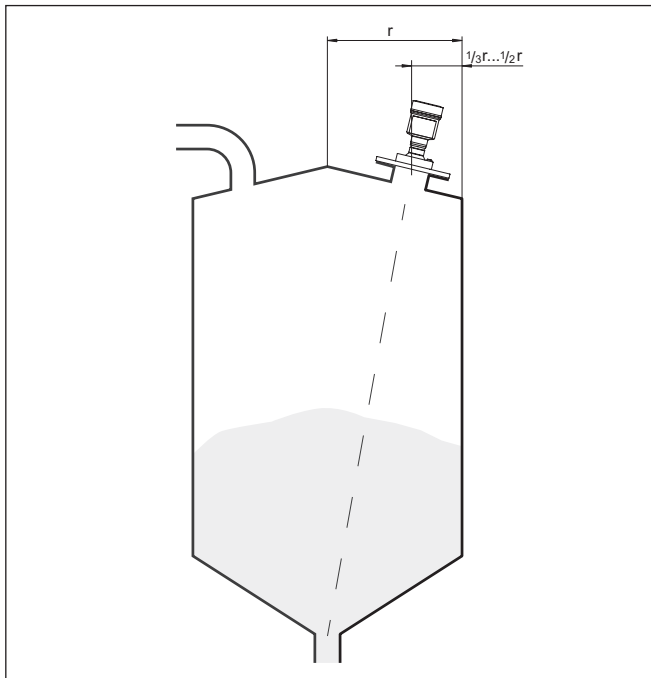
插图. 34: 安装位置和校准
