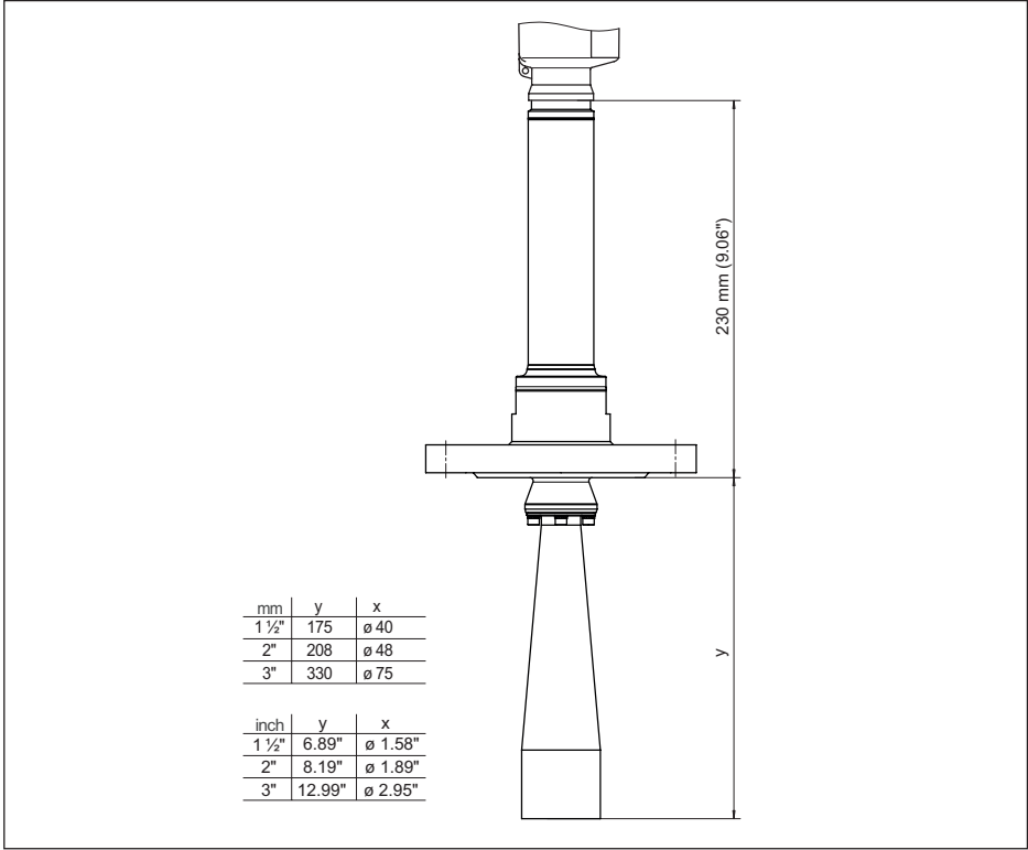
插图. 105: VEGAPULS 6X, 带有喇叭口天线的法兰，+450 °C 型
