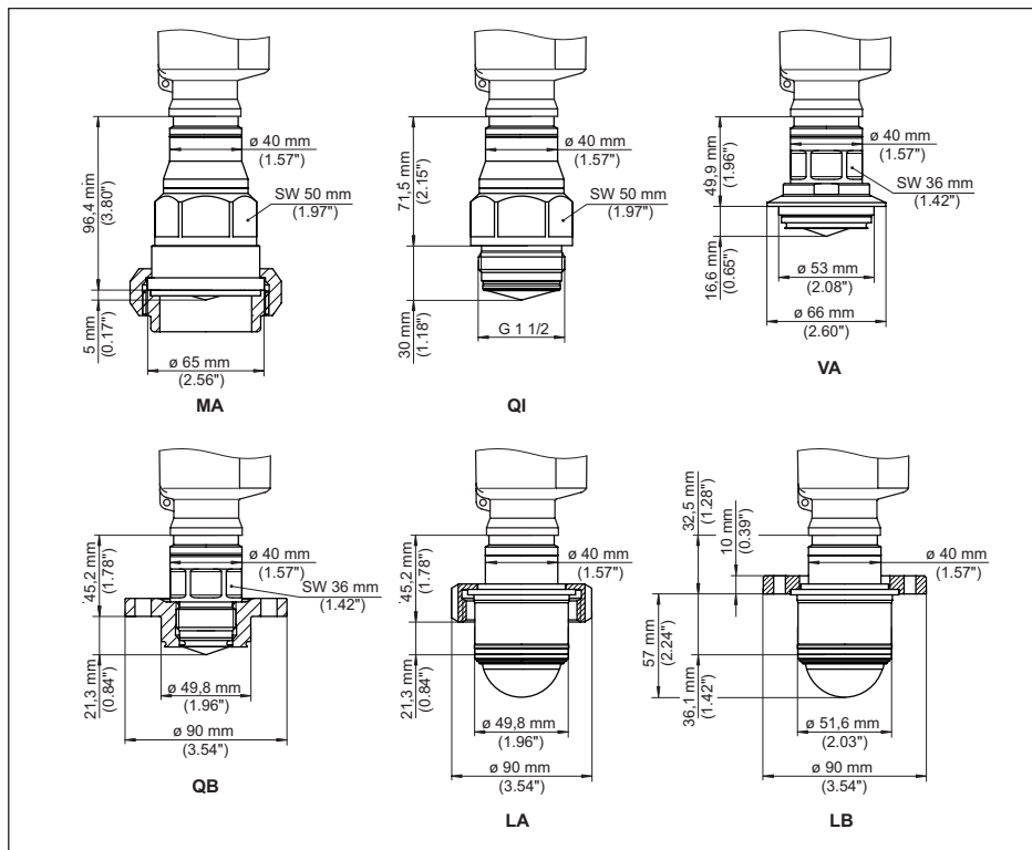
插图. 110: VEGAPULS 6X, 卫生型接口
