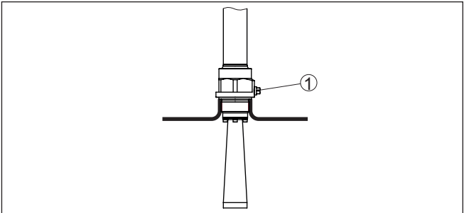
插图. 43: 带有吹气接口的喇叭口天线 +450 °C 版本
