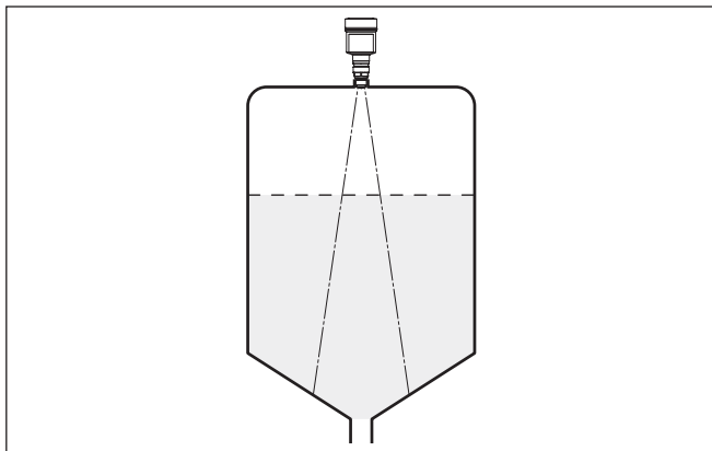
插图. 20: 将雷达仪表安装到带有锥形底部的容器上
