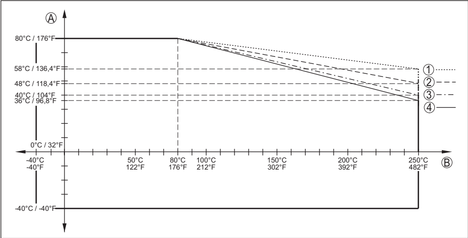
插图 87: 环境温度降额, 带喇叭口天线的法兰, 至 +250 °C (+482 °F)
