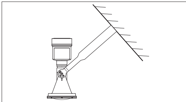
插图. 15: 用长度为 300 毫米的龙门框将仪表安装在倾斜的墙壁上
