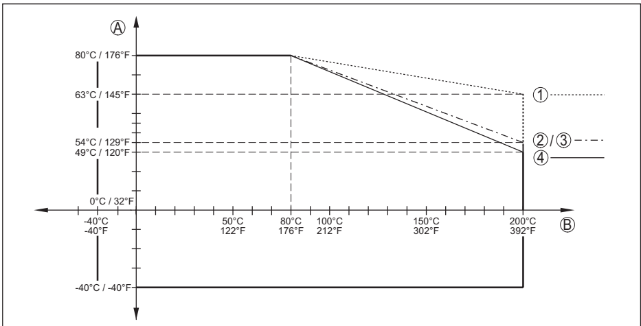
插图. 82: 环境温度降额, 带透镜天线的法兰, 至 +200 °C (+392 °F)
