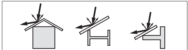
插图. 32: 用散射挡板来覆盖光滑的型材
