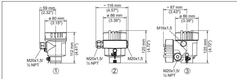
插图. 93: 采用防护等级达 IP66/IP68 (0.2 bar) 的壳体版本, (内装显示和调整模块后, 壳体高度增加了18 mm/0.71 in)
