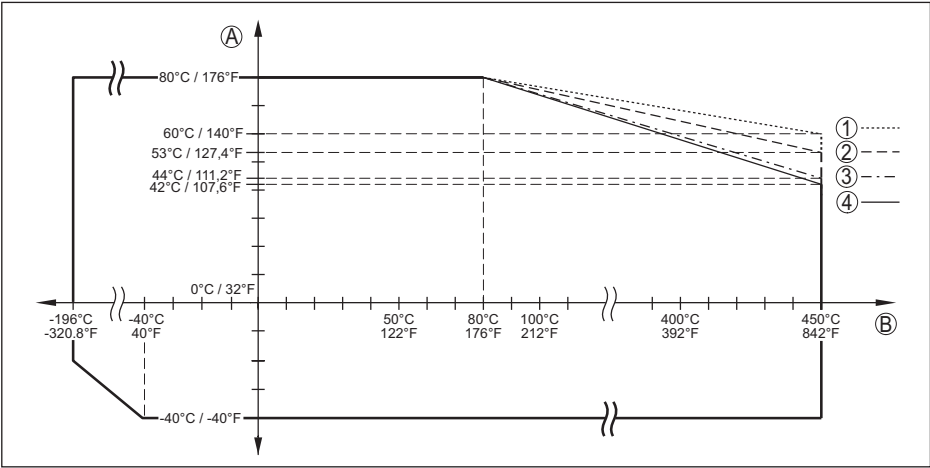
插图 88: 环境温度降额, 号角天线, 至 +450 °C (+842 °F)
