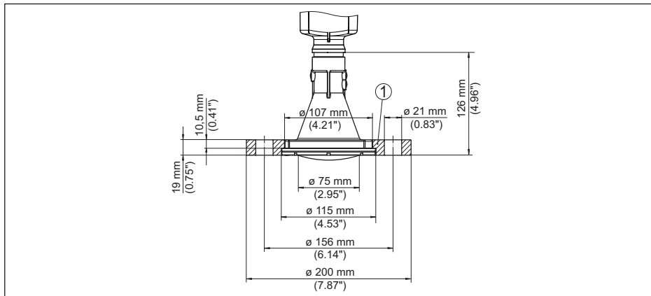
插图. 95: VEGAPULS 6X 带有锁紧法兰，适用于法兰 3" 150 lbs, DN 80 PN 16
