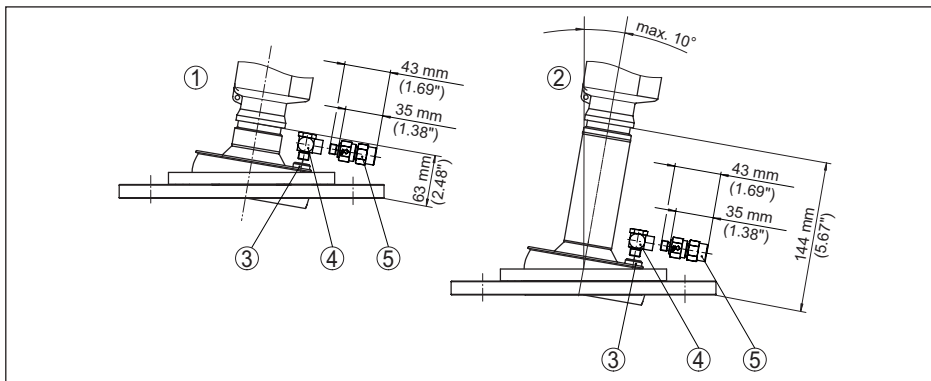
插图. 114: VEGAPULS 6X, 带有透镜天线、万向节和吹气接口的法兰
