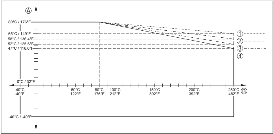
插图: 83: 环境温度降额, 带透镜天线的法兰, 至 +250 °C (+482 °F)
