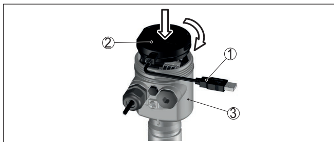
插图. 63: 通过接口适配器将电脑直接与仪表相连
