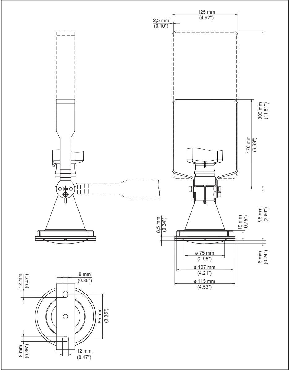
插图. 99: VEGAPULS 6X, 塑料制喇叭口天线, 龙门框, 长度为 170 或 300 mm
