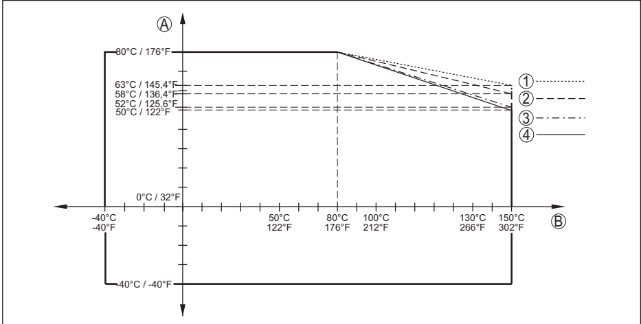
插图. 81: 环境温度降额, 带透镜天线的法兰, 至 +150 °C (+302 °F)
