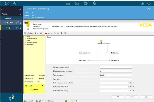
插图. 66: DTM 视图 (举例)
