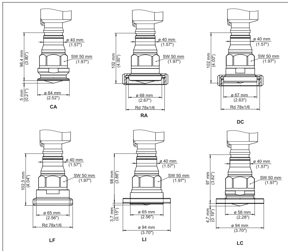
插图. 109: VEGAPULS 6X, 卫生型接口
