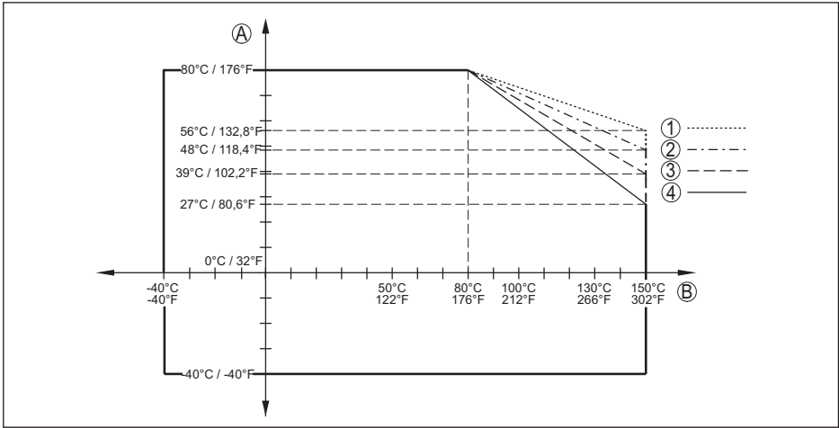
插图: 84: Derating Umgebungstemperatur, Hygieneanschluss bis +150 °C (+302 °F)
