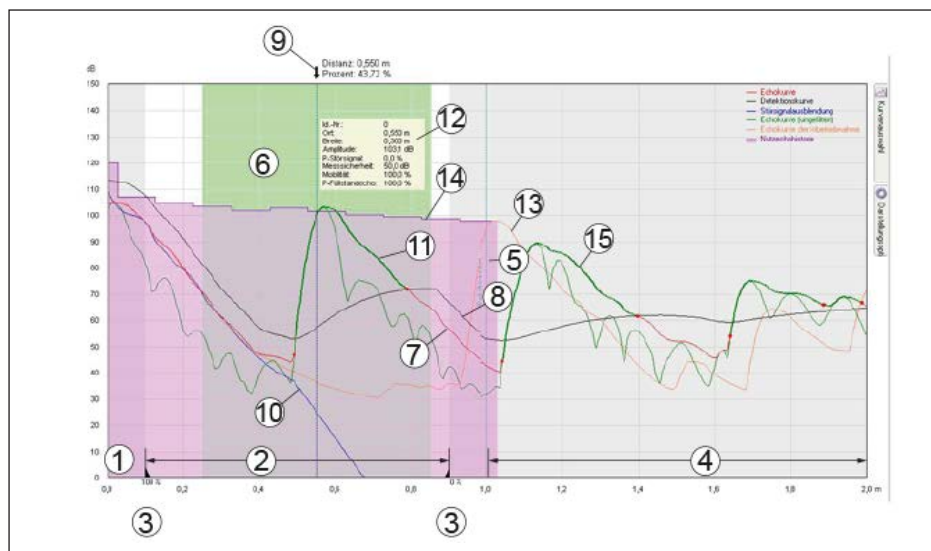
插图. 68: 回波曲线窗口内的范围
