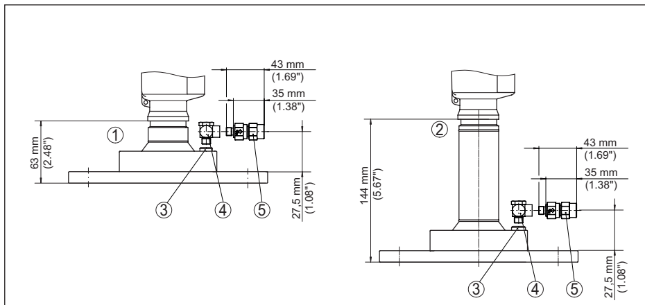
插图. 112: VEGAPULS 6X, 带有透镜天线和吹气接口的法兰
