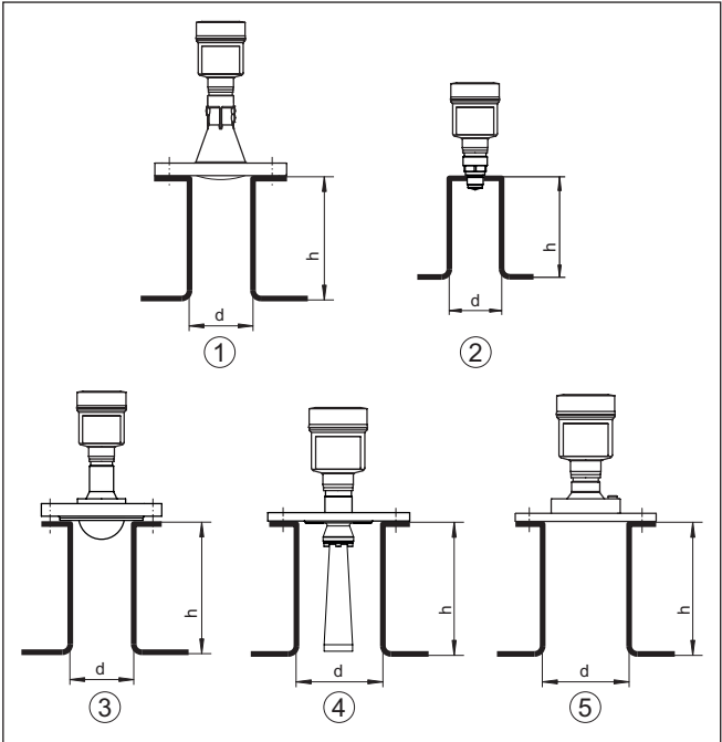
插图. 27: 当管接头的尺寸有别时管接头的安装
