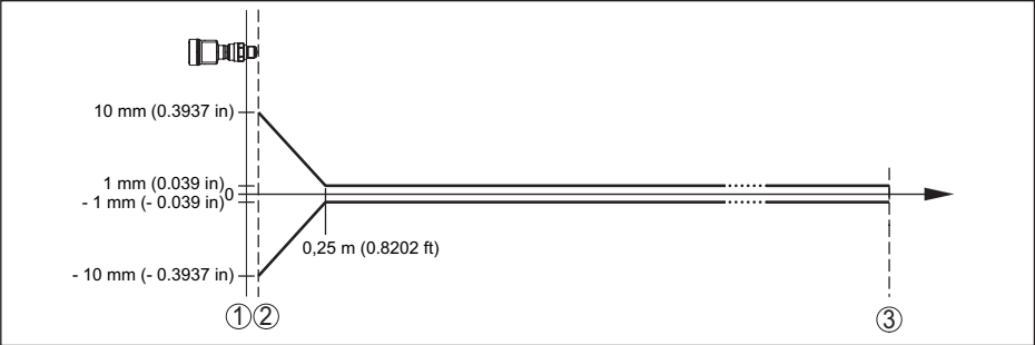
插图 72: 基准条件下的测量误差 (以带有内置天线系统的螺纹为例，相应地适用于所有版本) 18)
