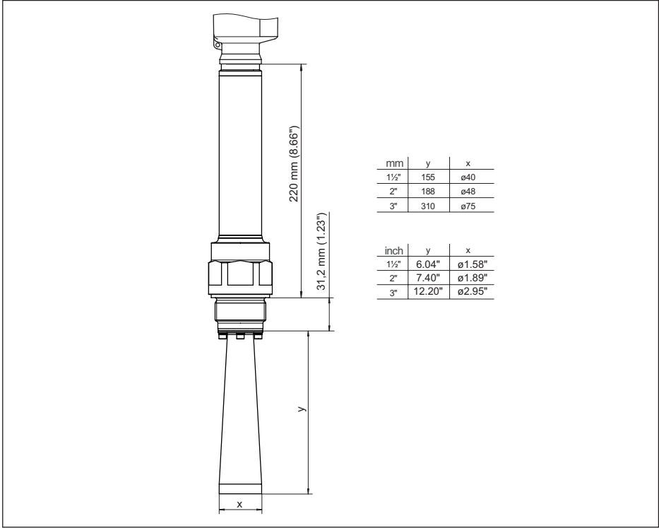
插图. 104: VEGAPULS 6X, 带有喇叭口天线的螺纹， +450 °C 型
