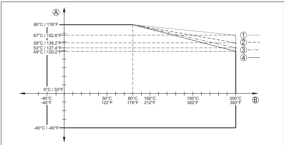
插图: 86: 环境温度降额, 带喇叭口天线的法兰, 至 +200 °C (+392 °F)
