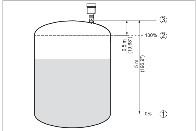
插图. 56: 参数调整举例: 最小/最大调整 - 液体
