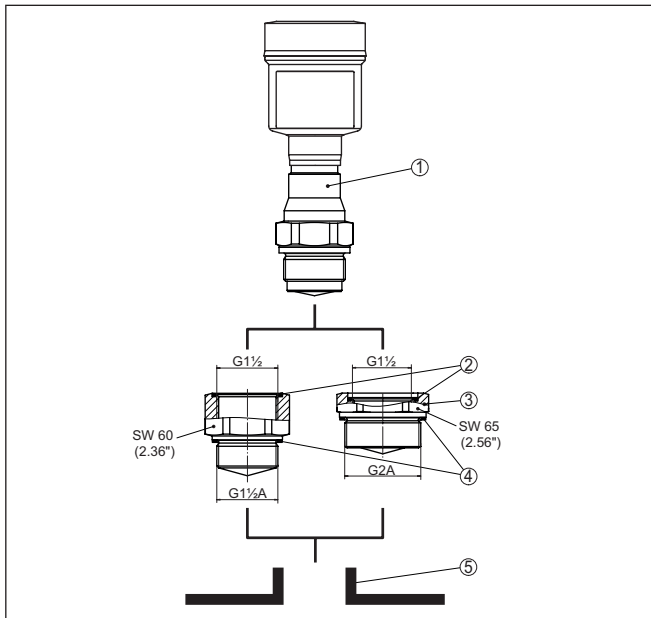
插图. 30: PTFE 螺纹适配器 (举例: 带螺纹 G1½)
