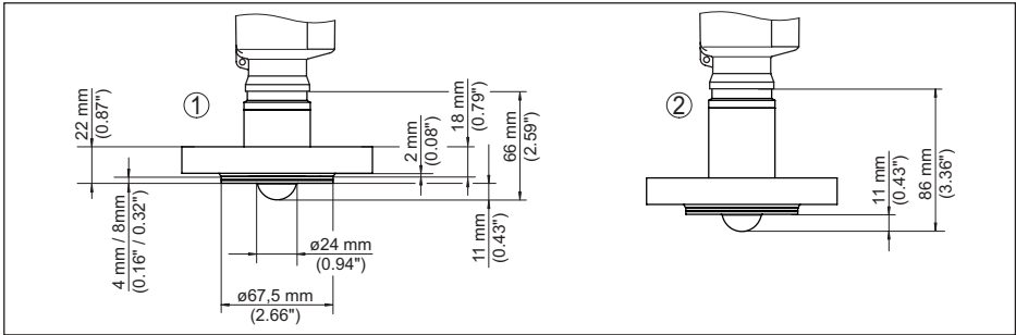
插图. 106: VEGAPULS 6X, 封装天线系统 DN 25 PN 40
