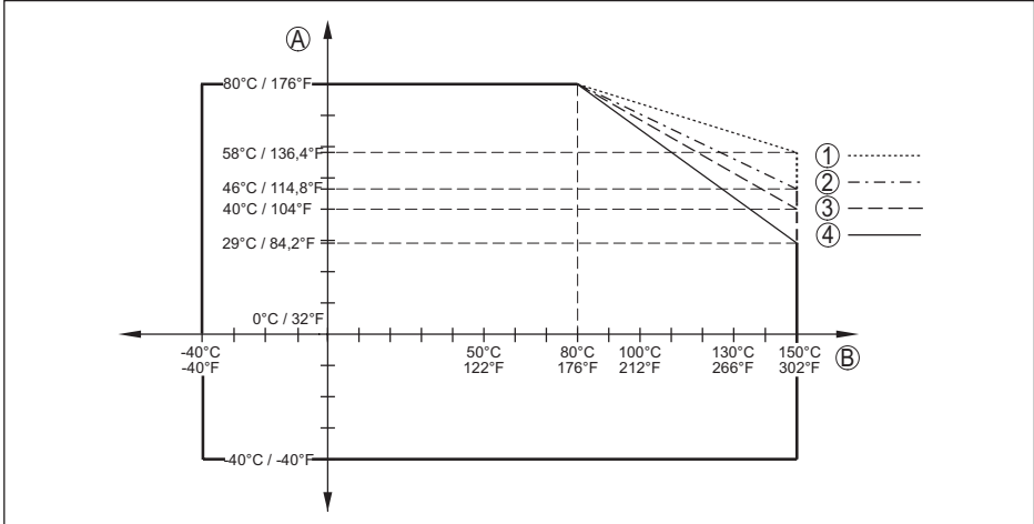
插图: 85: 环境温度降额, 带喇叭口天线的法兰, 至 +150 °C (+302 °F)
