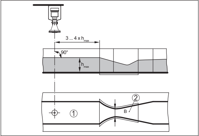
插图. 49: 用卡发基-文丘里槽来测量流量: h_{max} = 水槽的最大灌装量; B = 水槽的最大收缩率
