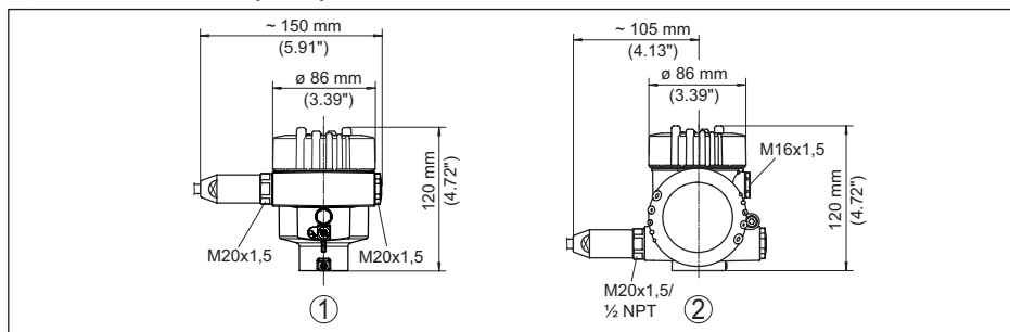
插图 92: 采用防护等级达 IP66/IP68 (1 bar) 的壳体版本 (内装显示和调整模块后, 壳体高度增加了18 mm/0.71 in)
