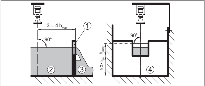
插图. 48: 用矩形槽测量流量: h_{max} = 矩形槽的最大注水高度
