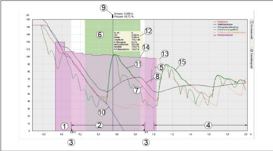
插图. 69: 回波曲线窗口内的范围连同“扩展的显示区域”这一显示选项
