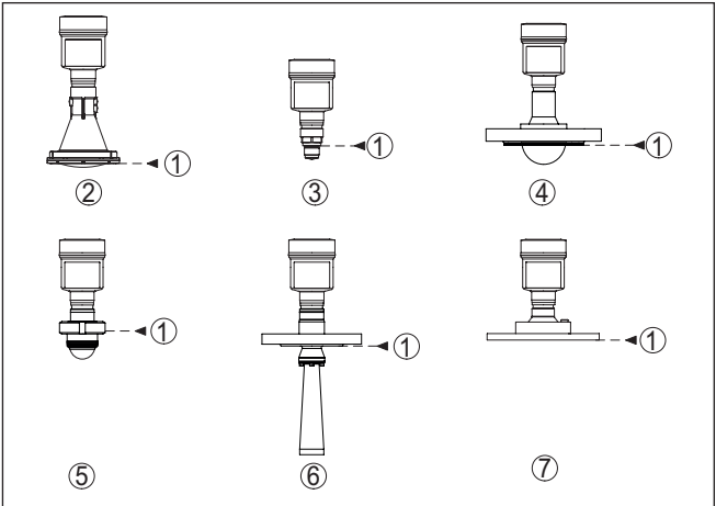
插图. 22: 基准面的位置
