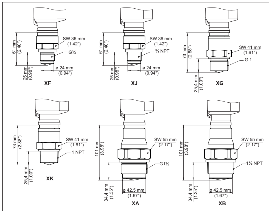
插图. 101: VEGAPULS 6X, 带有内置天线系统的螺纹，至 +150 °C (+302 °F)
