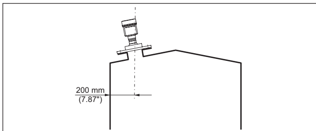
插图. 21: 将雷达仪表安装在容器盖上
