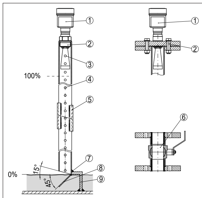
插图. 46: 构造 - 导波管 (举例)
