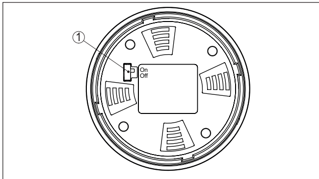
插图. 61: 激活蓝牙
