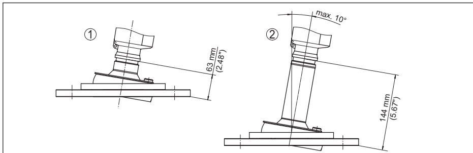
插图. 113: VEGAPULS 6X, 带有透镜天线和万向节的法兰
