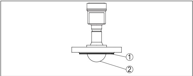
插图. 28: VEGAPULS 6X, 带法兰和塑封天线系统
