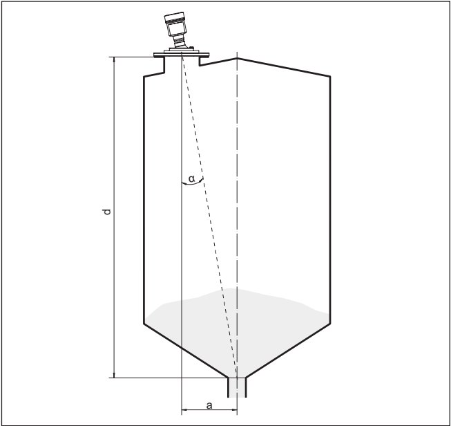
插图. 35: 测定倾斜角度以瞄准 VEGAPULS 6X
