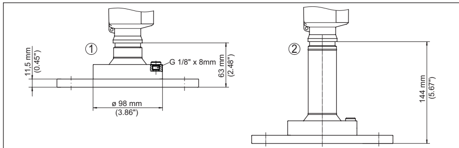
插图. 111: VEGAPULS 6X, 带有透镜天线的法兰 (法兰厚度参见图纸, 法兰尺寸根据 DIN, ASME, JIS)
