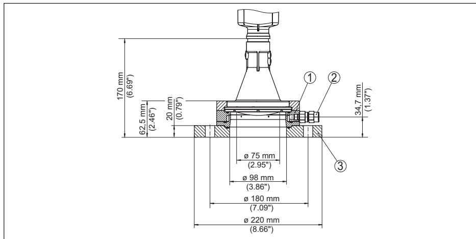
插图 98: VEGAPULS 6X, 适配法兰和吹气接口 DN 100 PN 6
