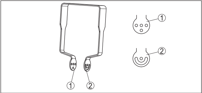
插图. 10: 龙门框 - 用于初步固定螺丝
