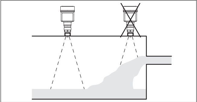
插图. 23: 流入介质时安装雷达仪表
