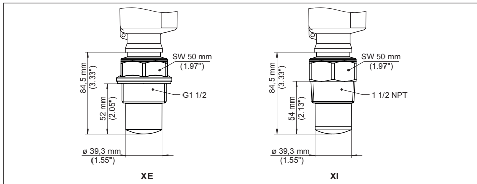
插图. 100: VEGAPULS 6X, 螺纹, 带有内置的用PVDF制成的天线系统的螺纹, 至 +80 °C (+176 °F), 用于无爆炸危险的区域时至 +100 °C (+212 °F)
