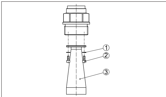
插图. 9: 构造 - 喇叭口天线 (举例)
