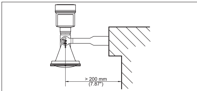
插图. 14: 用长度为 170 毫米的龙门框将仪表水平安装在墙壁上
