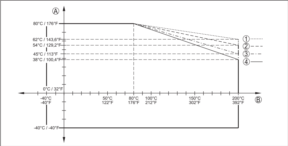
插图. 79: 环境温度降额, 带塑料天线系统的法兰, 至 +200 °C (+392 °F)
