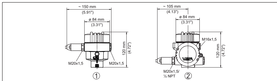
插图. 94: 采用防护等级达 IP66/IP68 (1 bar) 的壳体版本 (内装显示和调整模块后, 壳体高度增加了18 mm/0.71 in)
