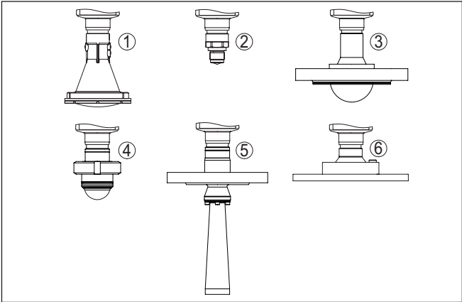
插图. 3: 天线系统 VEGAPULS 6X
