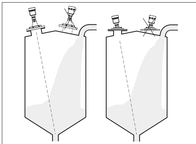
插图. 24: 从上面装料时雷达仪表的安装
