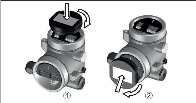
插图. 53: 将显示和调整模块装到双腔式壳体上
