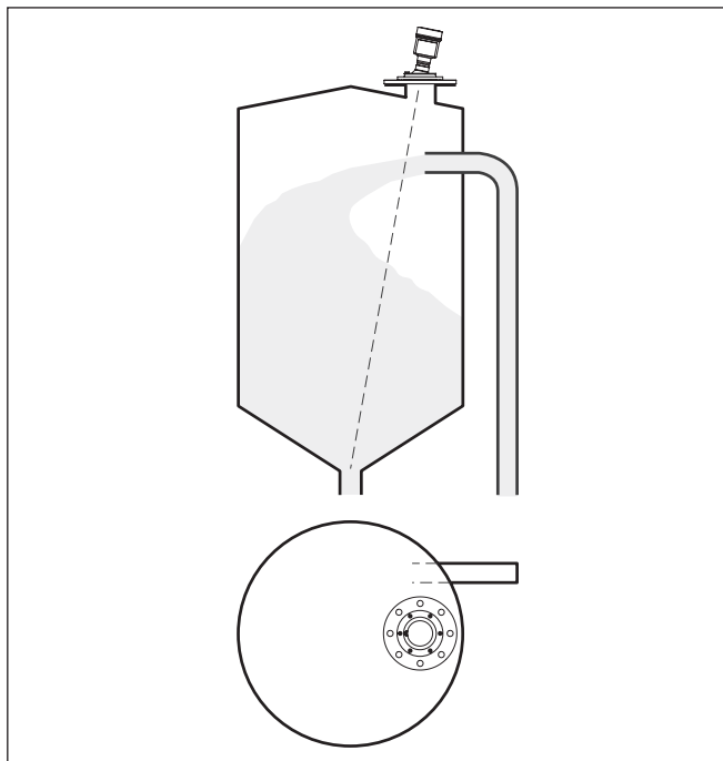
插图. 25: 从侧面装料时雷达仪表的安装
