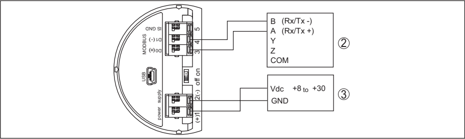
插图. 89: 将 VEGAPULS 6X 与 RTU Fisher ROC 809 相连接
