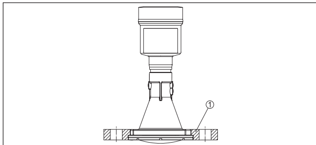
插图. 16: 组合式锁紧法兰
