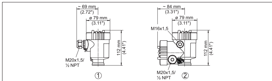
插图 90: 采用防护等级为 IP66/IP67 的外壳版本 (内装显示和调整模块后, 外壳高度增加了 9 mm/0.35 in)
