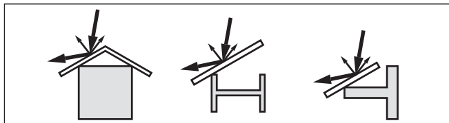
插图. 14: 用散射挡板来覆盖光滑的型材
