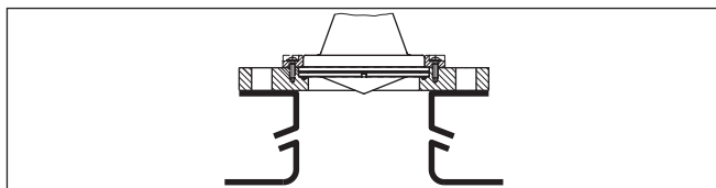
插图. 15: 空气冲洗接头
