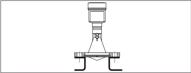
插图. 9: 值得推荐的管接头安装方法
