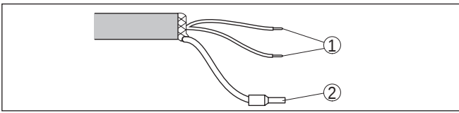
插图. 25: 连接电缆的芯线分布
