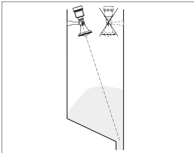
插图. 13: 在多腔式料仓中进行安装和校准
