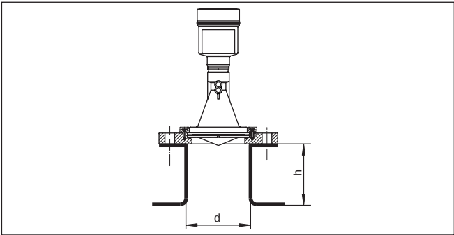
插图. 9: 值得推荐的管接头安装方法
