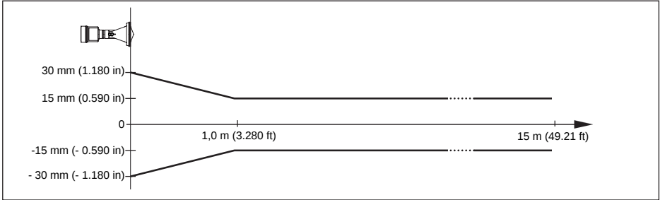
插图. 32: VEGAPULS 67 的测量偏差
