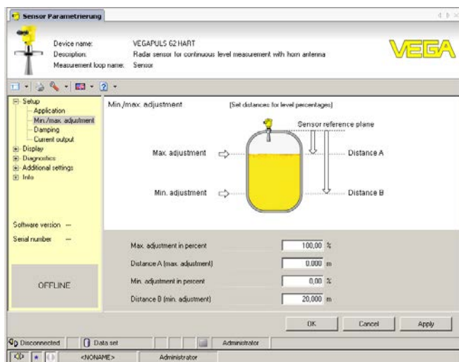
插图. 32: DTM 视图举例
