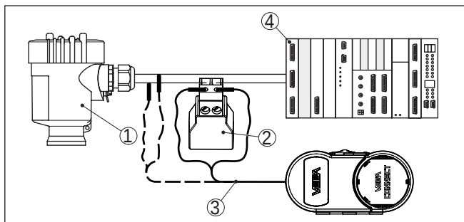
插图. 31: 通过 HART 将电脑与信号线路相连
