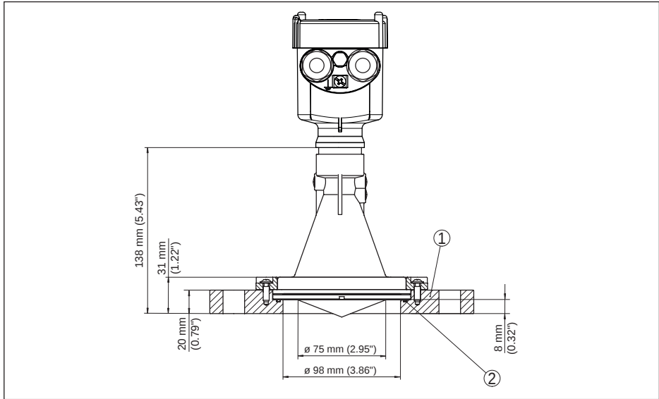
插图. 41: VEGAPULS 67, 适配法兰 DN 100, DN 150
