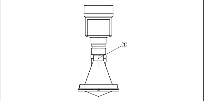
插图. 4: 偏振层在 VEGAPULS 67 上的位置
