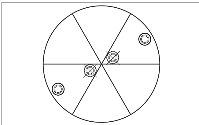
插图. 12: 在多腔式料仓中进行安装和校准
