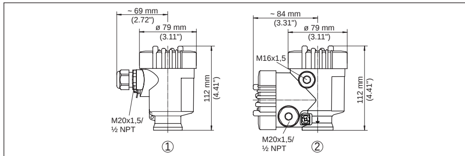
插图. 34: 采用保护方式为 IP 66/IP 67 的外壳型式 (内装显示和调整模块后, 外壳高度增加了 9 mm/0.35 in)
