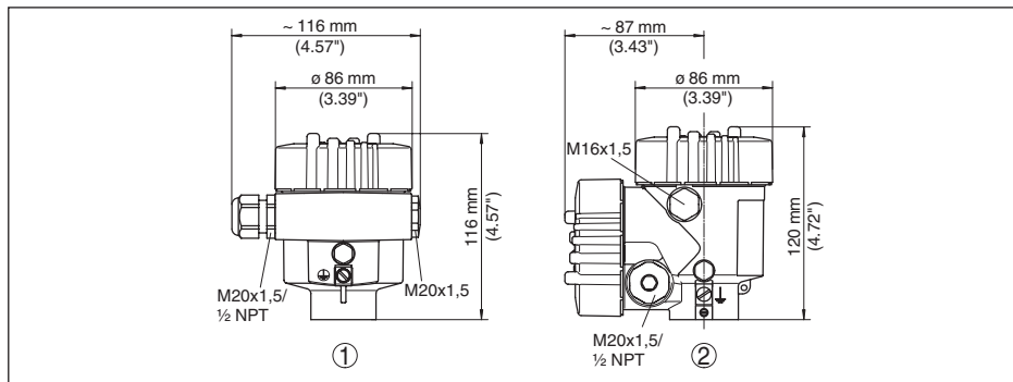
插图. 35: 采用保护等级达 IP 66/IP 68 (0.2 bar) 的壳体型式 (内装显示和调整模块后, 壳体高度增加了18 mm/0.71 in)
