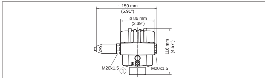
插图. 36: 采用保护等级达 IP 66/IP 68 (1 bar) 的壳体型式 (内装显示和调整模块后, 壳体高度增加了18 mm/0.71 in)
