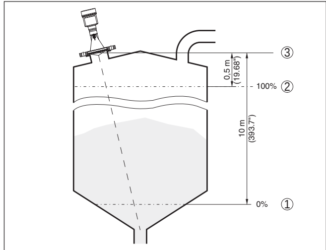
插图. 28: 参数化举例
