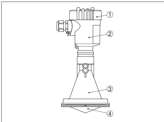
插图. 1: VEGAPULS 67, 带塑料外壳的型式
