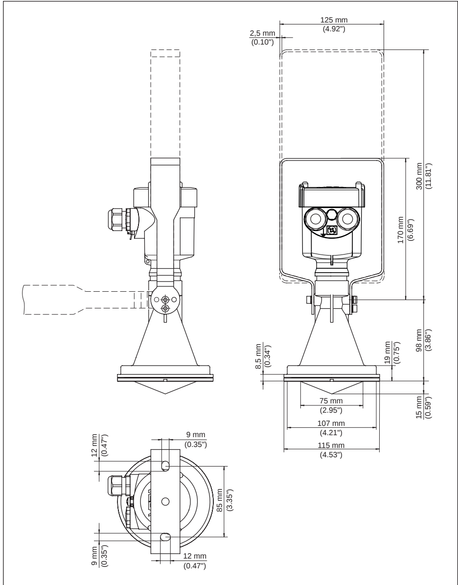
插图. 39: VEGAPULS 67, 带有长度为 170 或 300 毫米的龙门框的型式
