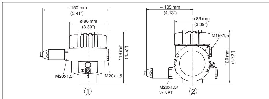
插图. 51: 采用保护等级达 IP 66/IP 68 (1 bar) 的壳体型式 (内装显示和调整模块后，壳体高度增加了18 mm/0.71 in)
