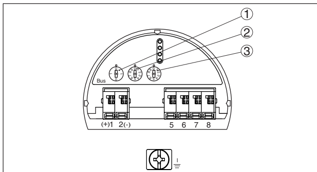
插图. 21: 地址选择开关
