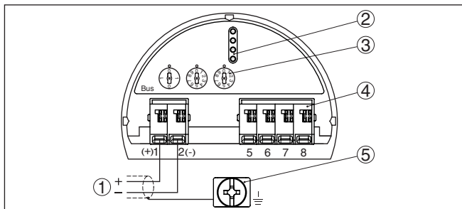
插图. 12: 单腔式壳体的电子部件和接线腔
