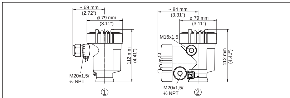
插图. 49: 采用保护方式为 IP 66/IP 67 的外壳型式 (内装显示和调整模块后, 外壳高度增加了 9 mm/0.35 in)
