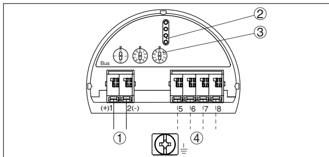
插图. 15: 防爆 (Ex-d-ia) 型双腔式壳体的电子部件腔
