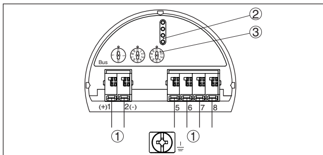
插图. 13: 双腔式壳体的电子部件腔
