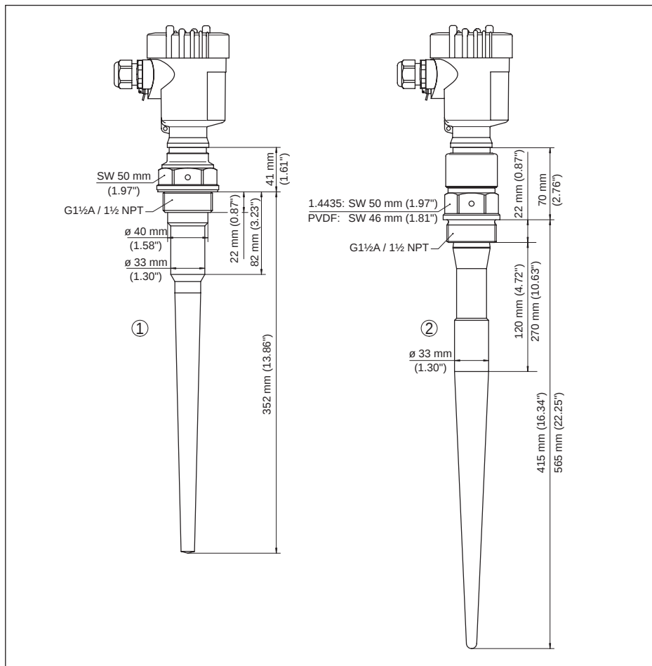
插图. 52: VEGAPULS 65, 螺纹型
