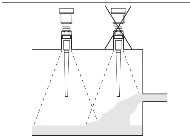
插图. 6: 流入介质时安装雷达传感器
