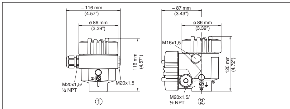
插图. 50: 采用保护等级达 IP 66/IP 68 (0.2 bar) 的壳体型式 (内装显示和调整模块后, 壳体高度增加了18 mm/0.71 in)
