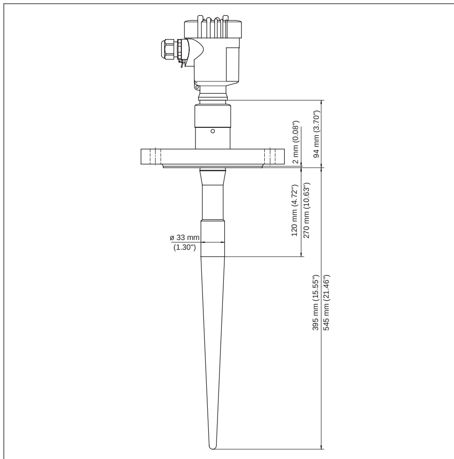
插图. 53: VEGAPULS 65, 法兰型, 用于100 mm 高 (无源长度 120 mm, 4 23/32") 或 250 mm 高 (无源长度 270 mm, 10 5/8") 的接头
