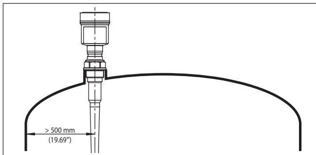
插图. 4: 将雷达传感器安装在圆形容器盖上
