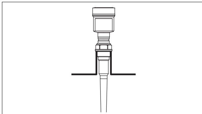
插图. 7: 值得推荐的管接头安装方法
