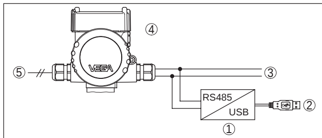
插图. 16: 电脑通过接口适配器与 RS 485 电线相连接
