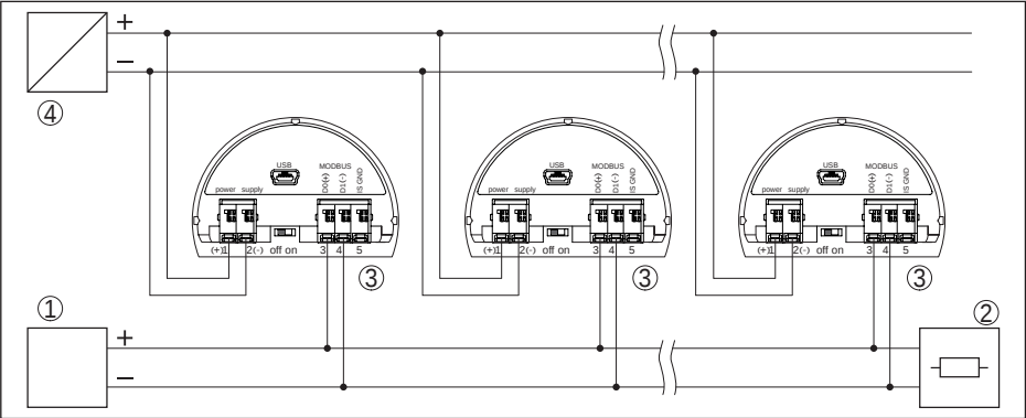
插图. 28: Modbus 总线结构
