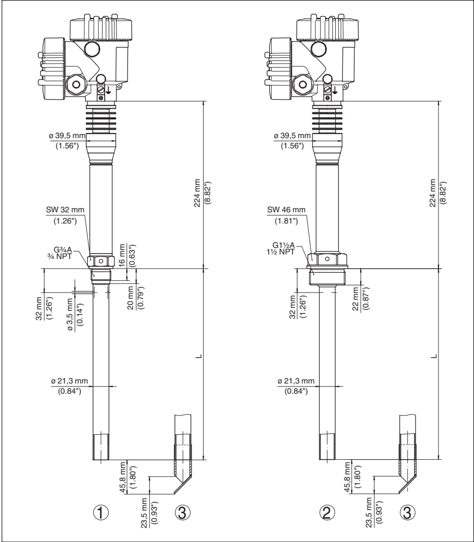
插图. 35: VEGAPULS 62, 带螺纹的立管型 8)
