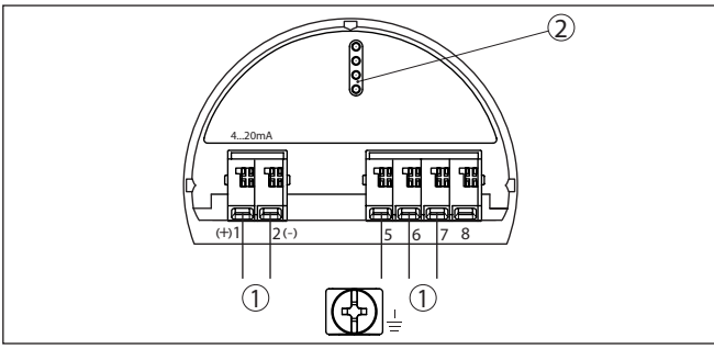
插图. 6: 双腔式壳体的电子部件腔
