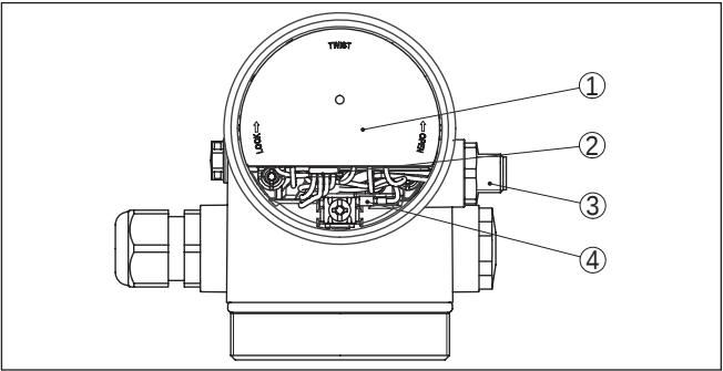
插图. 8: 目检带有与外部显示和调整单元相连接的 VEGADIS-Adapter 的电子部件腔
