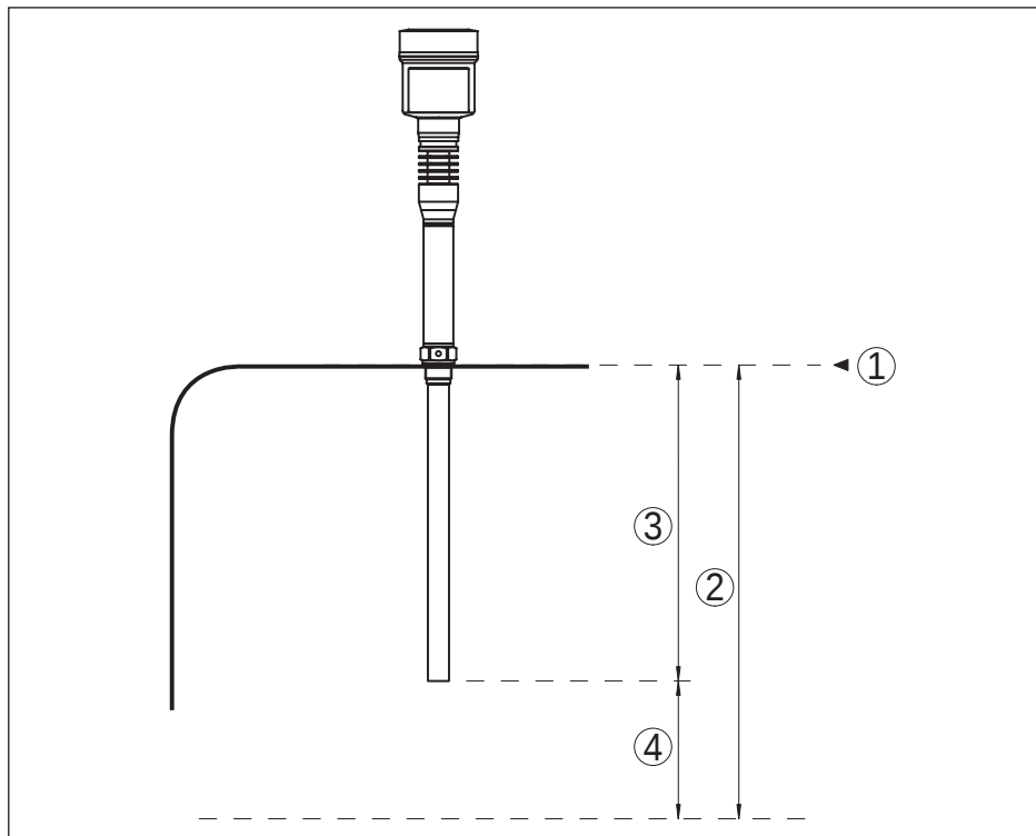
插图. 26: 有关输入值的信息
