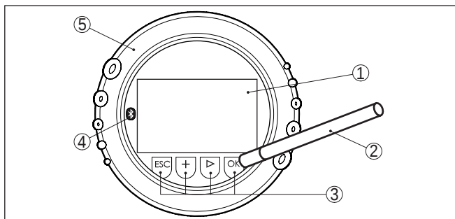
插图. 12: 显示和调整元件 - 拥有磁笔操作功能
