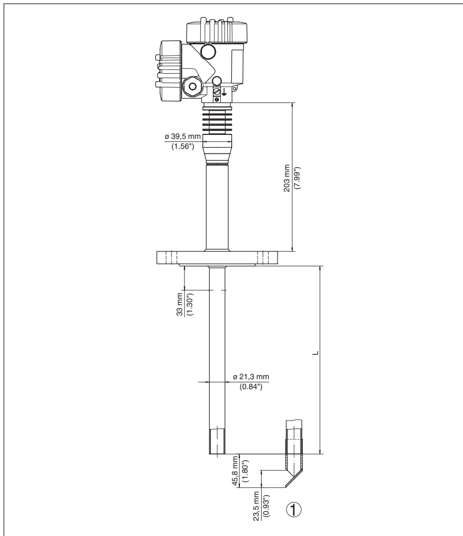
插图. 36: VEGAPULS 62, 带法兰的立管型 9)
