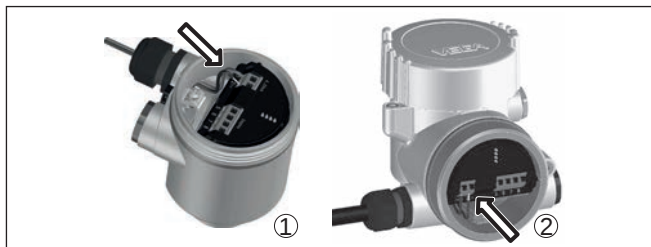
插图. 4: 接线步骤5和6
