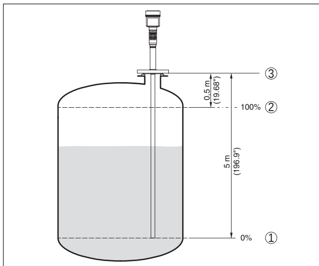
插图. 13: 有关最小/最大调整的参数化举例
