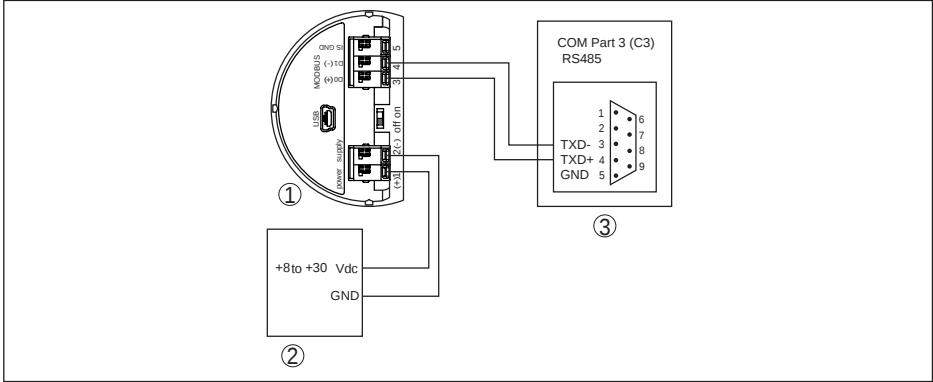
插图. 33: 将 VEGAPULS 62 与 RTU ScadaPack 相连接
