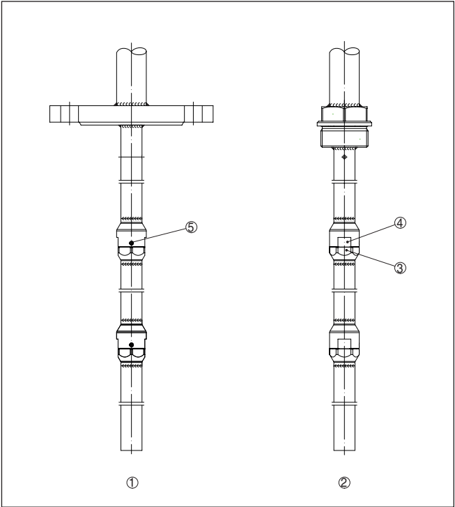
插图. 3: 组装好的多段式立管天线
