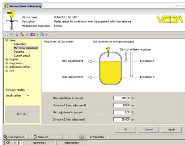
插图. 17: DTM 视图举例
