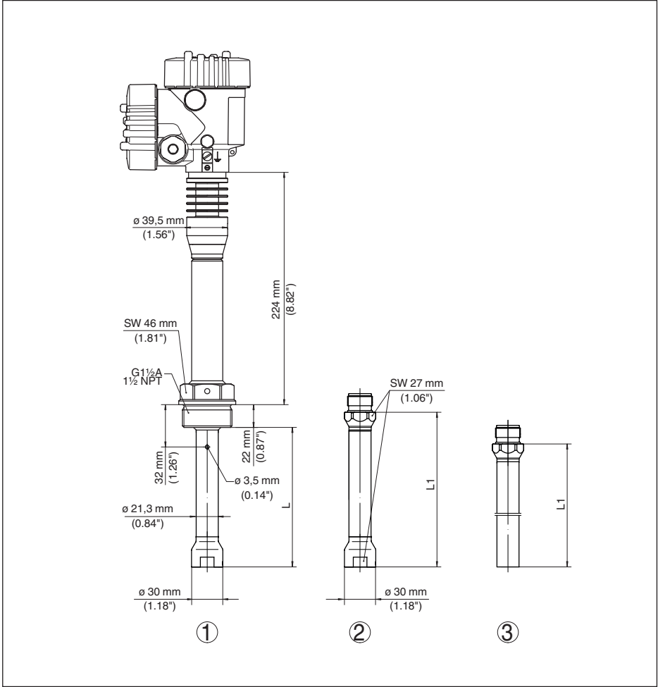
插图. 37: VEGAPULS 62, 用于带螺纹的立管延长件的型式 10)
