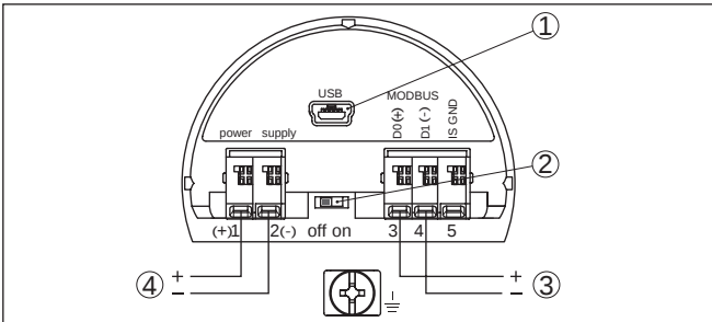
插图. 7: 接线腔
