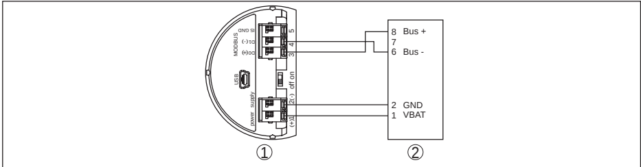
插图. 30: 将 VEGAPULS 62 与 RTU ABB Total Flow 相连接
