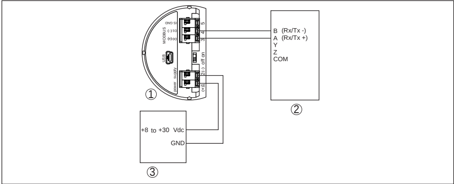
插图. 29: 将 VEGAPULS 62 与 RTU Fisher ROC 809 相连接
