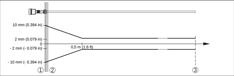
插图. 27: 在基准条件下的测量偏差
