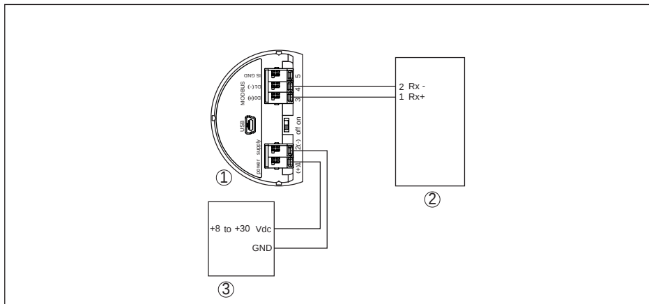
插图. 31: 将 VEGAPULS 62 与 RTU Thermo Electron Autopilot 相连接
