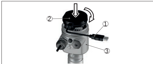
插图. 14: 通过接口适配器将电脑直接与传感器相连
