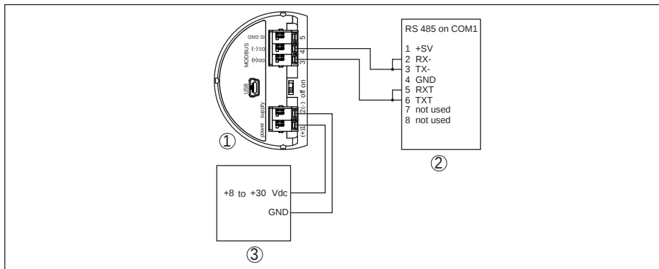
插图. 32: 将 VEGAPULS 62 与 RTU Bristol ControlWave Micro 相连接
