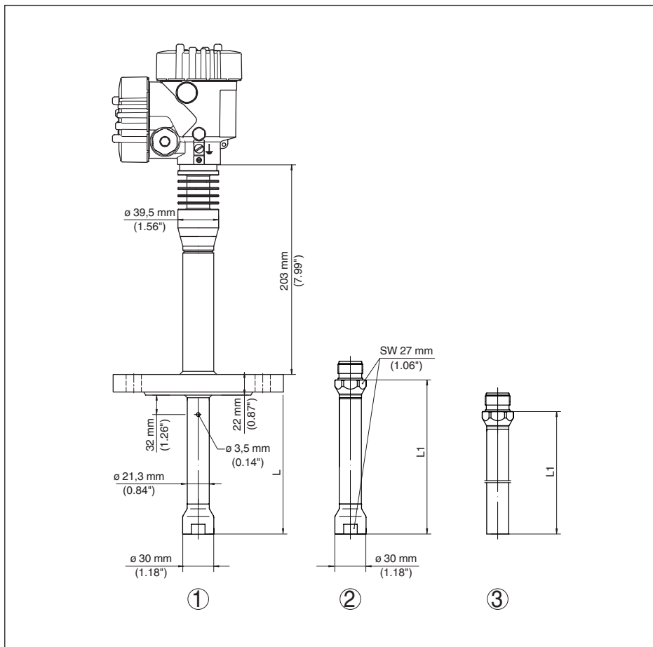
插图. 38: VEGAPULS 62, 用于带法兰的立管延长件的型式 11)
