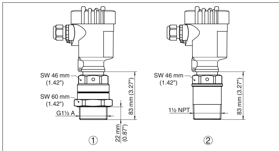
插图. 9: VEGAMIP 61, 内置的号角天线 (螺纹型)
