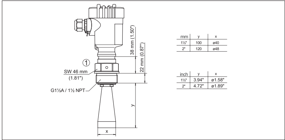
插图. 11: VEGAMIP 61, 号角天线 (316L)
