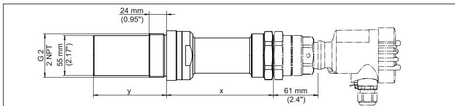
插图. 14: 带筒管的安装适配件 (选购件), 用于正面齐平式安装, 用于带有内置号角天线的 VEGAMIP 61, 螺纹型 G1½ 带 PTFE 盖 (也可以带 1½ NPT 螺纹)
