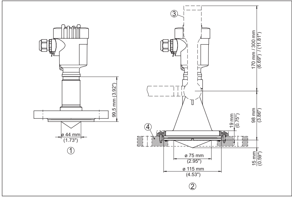
插图. 10: VEGAMIP 61，封装天线
