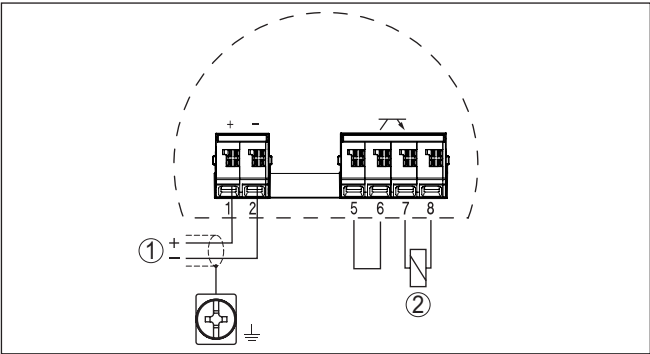
插图. 21: 接收单元的接线图 - VEGAMIP 61 (Receiver) - PNP 表现
