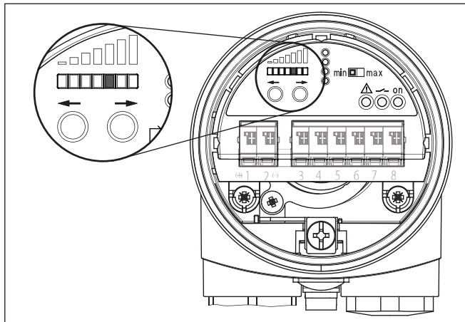
插图. 27: LED 显示条 - 为信号阻尼较低的介质进行设置
