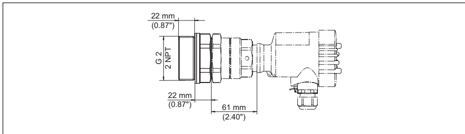
插图. 33: 带有陶瓷盖的安装适配件 (选购件), 用于带有内置号角天线的 VEGAMIP 61, 螺纹型 G1½, 带 PTFE 盖 (也可带 1½ NPT 螺纹)
