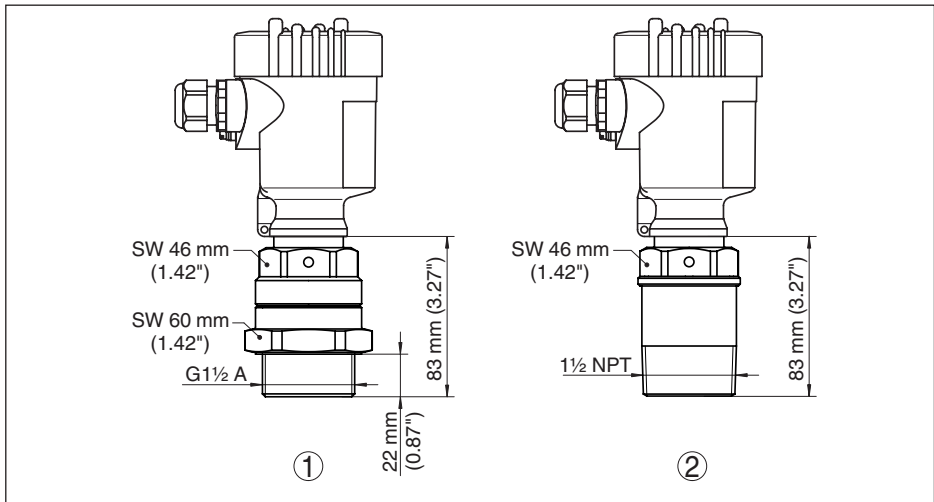
插图: 30: VEGAMIP 61, 内置的号角天线 (螺纹型)
