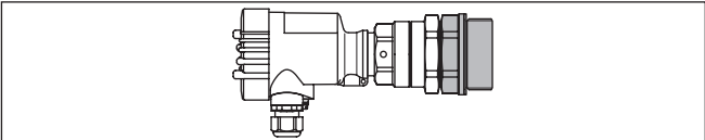
插图. 3: VEGAMIP 61 带有防磨损的陶瓷安装适配件 -40 ... +80 °C (-40 ... +176 °C)
