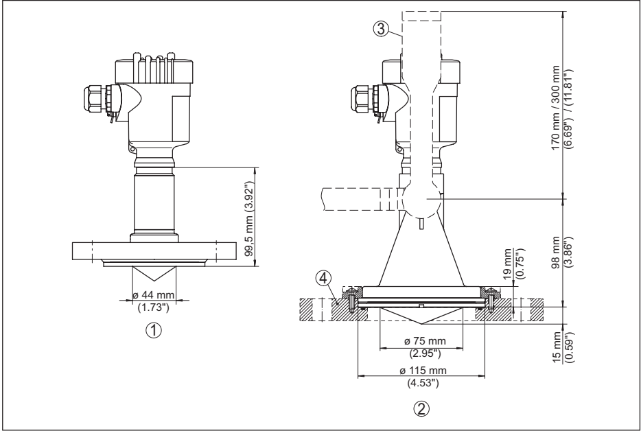
插图. 31: VEGAMIP 61，封装天线
