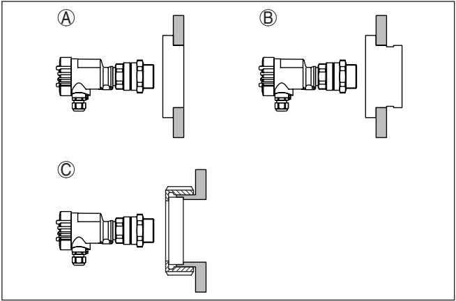
插图. 8: 安装在一个容器视窗前
