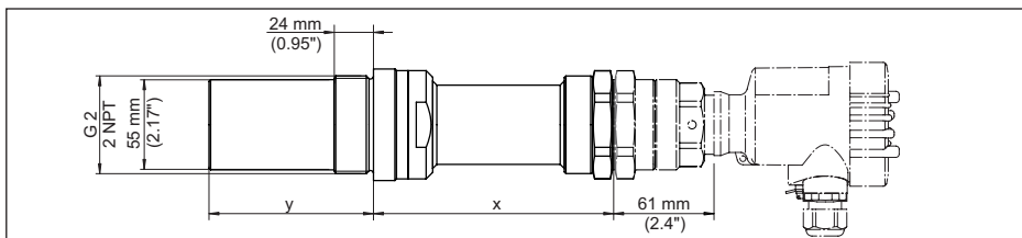
插图. 35: 带筒管的安装适配件 (选购件), 用于正面齐平式安装, 用于带有内置号角天线的 VEGAMIP 61, 螺纹型 G1½ 带 PTFE 盖 (也可以带 1½ NPT 螺纹)
