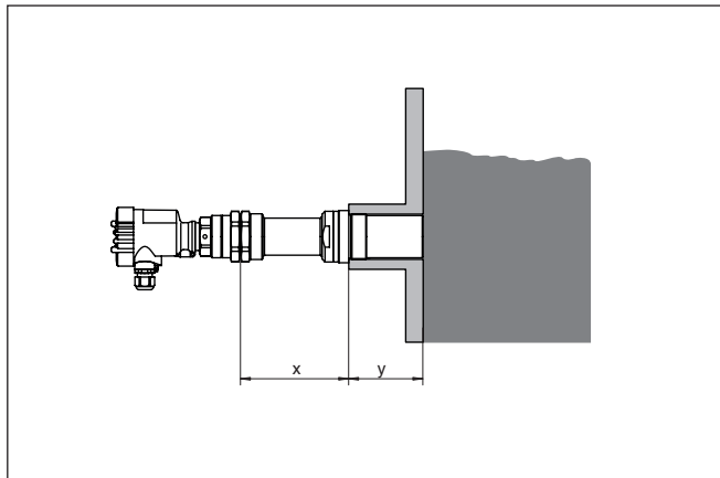
插图. 15: “带简管的高温型”安装适配件 -40 ... +450 °C (-40 ... +842 °F)，用于正面齐平式安装
