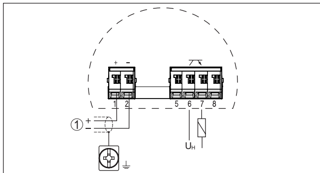
插图. 23: 接收单元的接线图 - VEGAMIP 61 (Receiver - 接收器) - 无电位
