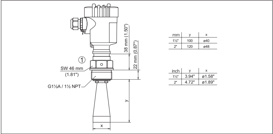
插图. 32: VEGAMIP 61, 号角天线 (316L)
