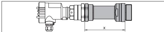
插图. 14: VEGAMIP 61 带安装适配件“高温型”-40 ... +450 °C (-40 ... +842 °F)
