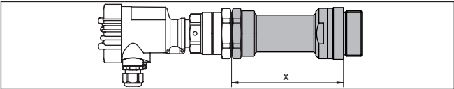
插图. 4: VEGAMIP 61 带安装适配件 "高温型" -40 ... +450 °C (-40 ... +842 °F) x 长度： "高温型" 安装适配件
