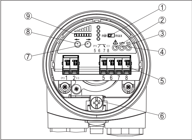
插图. 24: 电子插件 MP6X S (接收单元) - 晶体管输出口
