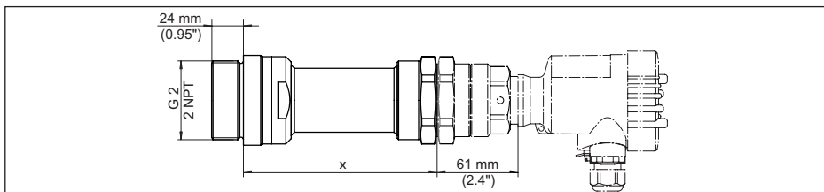
插图. 34: 带有陶瓷盖的安装适配件 (选购件), 用于带有内置号角天线的 VEGAMIP 61, 螺纹型 G1½, 带 PTFE 盖 (也可带 1½ NPT 螺纹)
