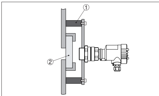
插图. 16: 容器振动时的安装
