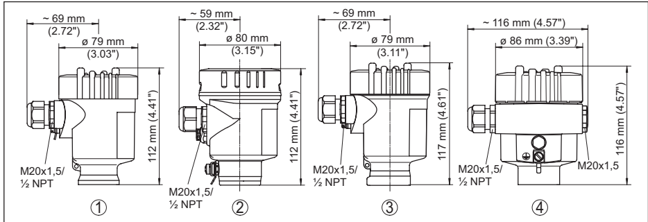
插图: 29: 外壳选型
