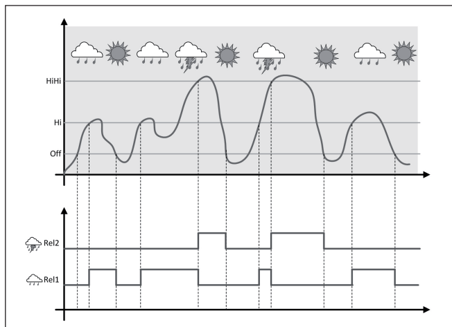
插图. 20: 用选项 "好天气运行" 来举例说明泵的控制
