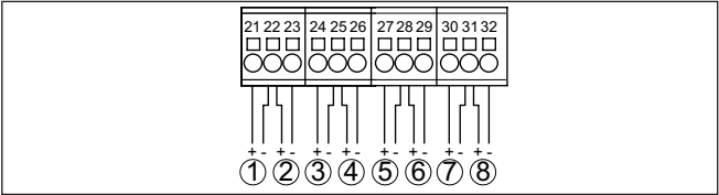
插图. 9: 数字输入端连接
