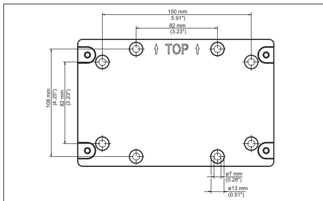
插图. 3: 用于壁挂式安装的安装板 VEGAMET 862
