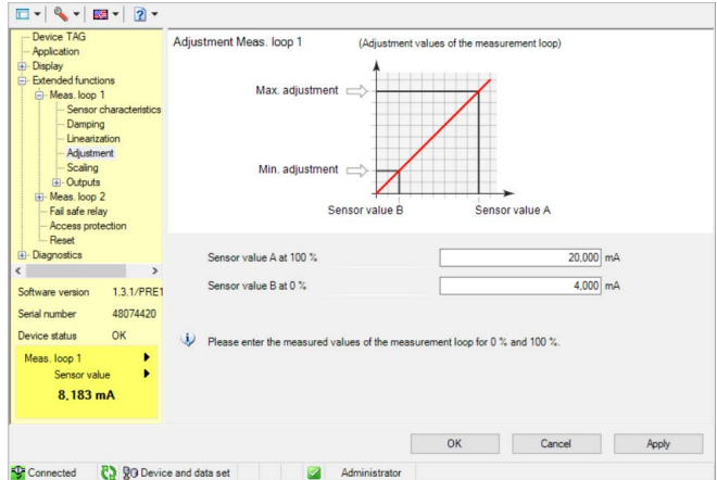
插图. 15: 一个 DTM 视图举例 - 调整
