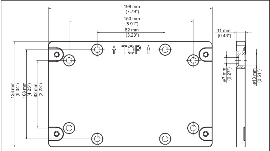
插图. 27: 安装板的尺寸
