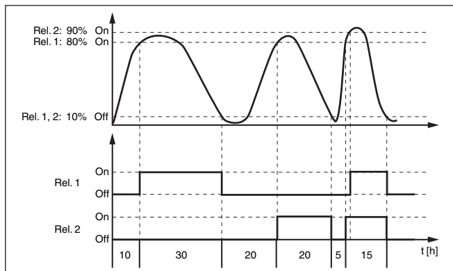
插图. 19: 示例: 泵控制器 2
