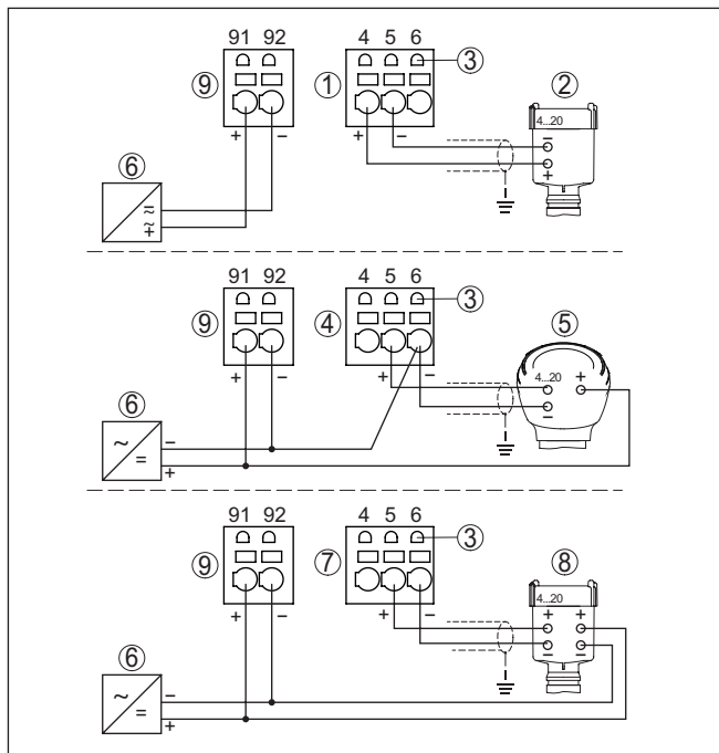
插图. 8: 两线制-/三线制-/四线制仪表的连接 (有源/无源)
