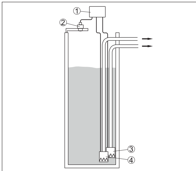
插图. 17: 泵站举例：在流入沟口控制泵
