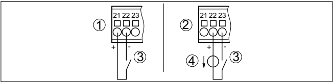
插图. 10: 数字输入端 (有源/无源) 的接口分布
