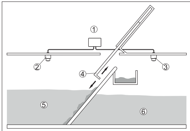
插图. 23: 格栅控制举例
