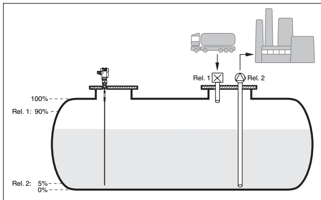
插图. 16: 举例说明对卧式圆形槽罐的物位测量
