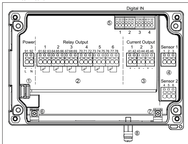
插图. 6: VEGAMET 862 的接线图
