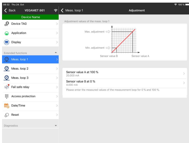
插图. 14: App 应用程序视图举例 - 调试 调整
