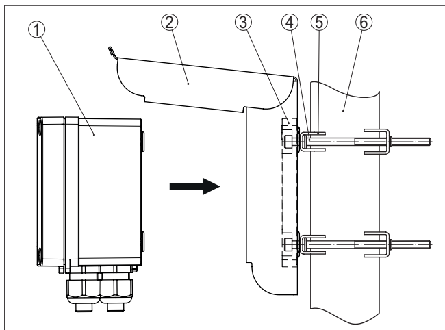
插图. 5: 将遮阳罩安装在管件上
