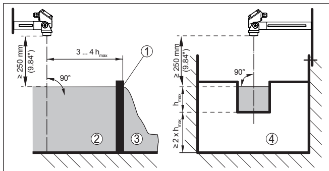
插图. 24: 用矩形槽测量流量: h_{\max} = 矩形槽的最大注水高度
