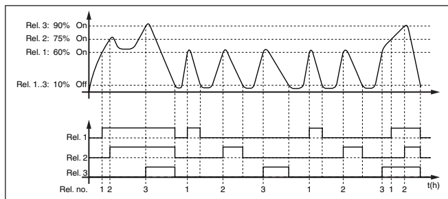
插图. 21: 泵控制器 4 的接通表现
