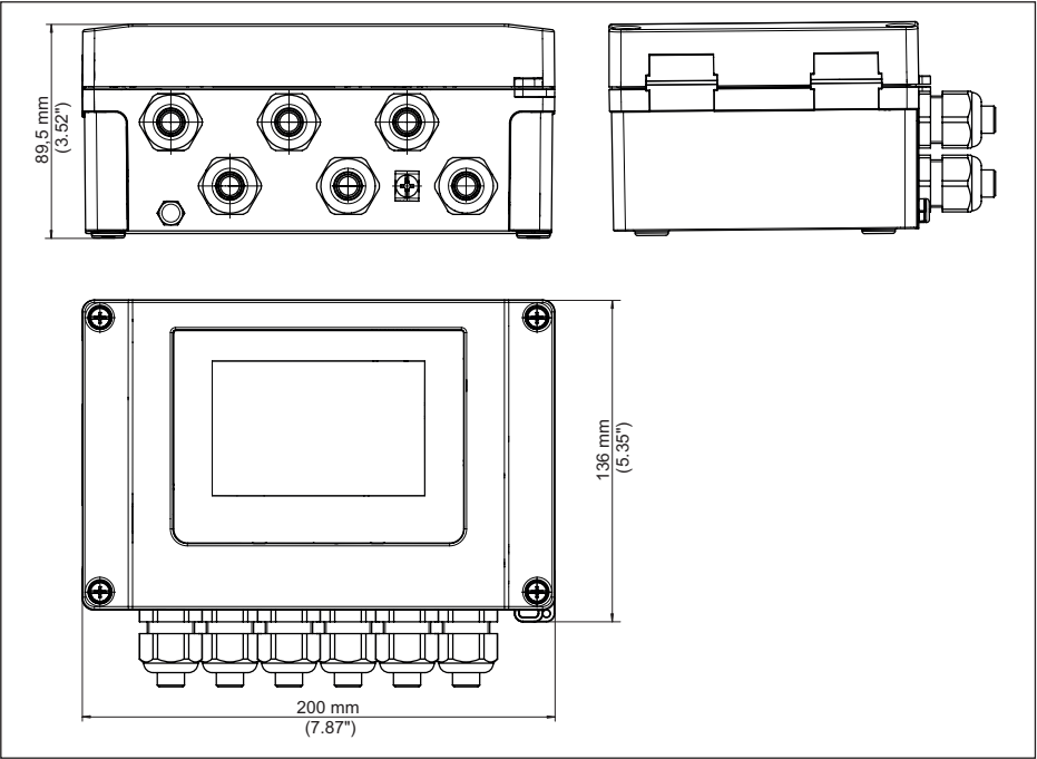
插图. 26: VEGAMET 862 的尺寸
