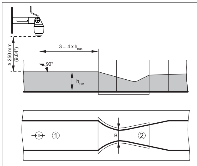
插图. 25: 用卡发基-文丘里槽来测量流量: h_{\max} = 水槽的最大灌装量; B = 水槽的最大收缩率
