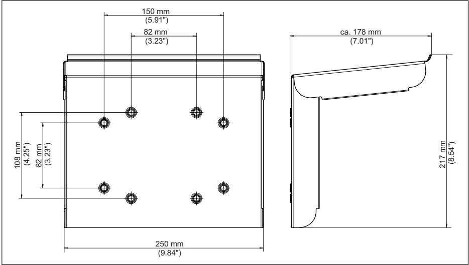
插图. 28: 遮阳罩的尺寸
