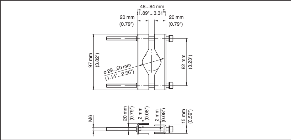
插图. 29: 用于安装在管件上用的夹子尺寸
