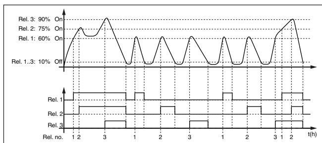
插图. 17: 泵控制器 4 的接通表现
