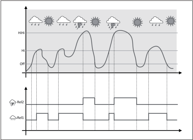
插图. 19: 用选项 "好天气运行" 来举例说明泵的控制
