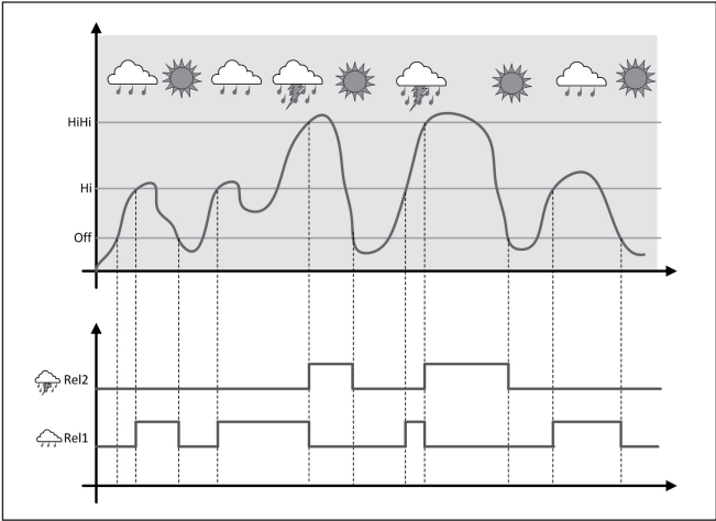
插图. 16: 用选项 "好天气运行" 来举例说明泵的控制
