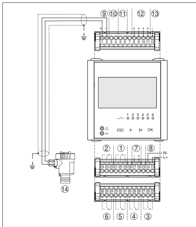
插图. 5: 带两线制传感器的接线图
