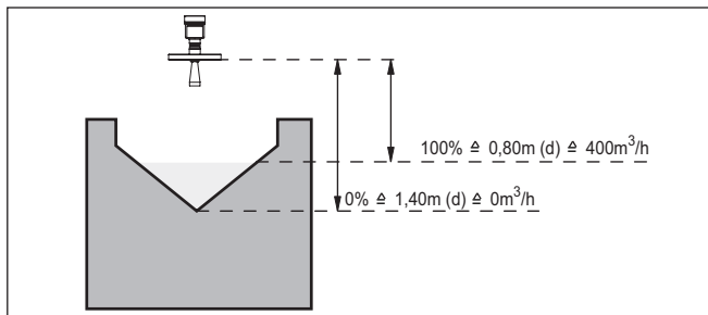
插图. 21: 用三角形水道调整流量的测量
