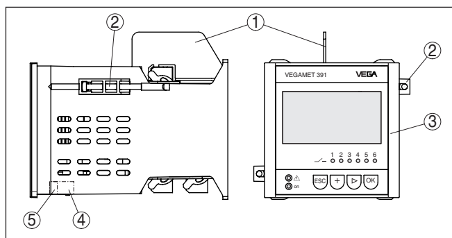
插图. 1: VEGAMET 391
