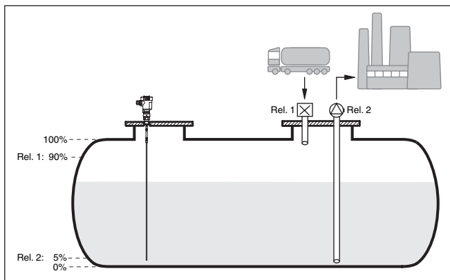
插图. 12: 举例说明对卧式圆形槽罐的物位测量
