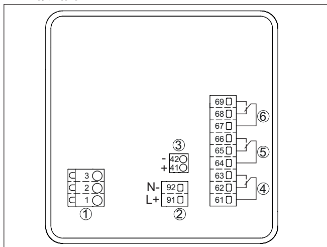
插图 4: VEGAMET 341 的接线图
