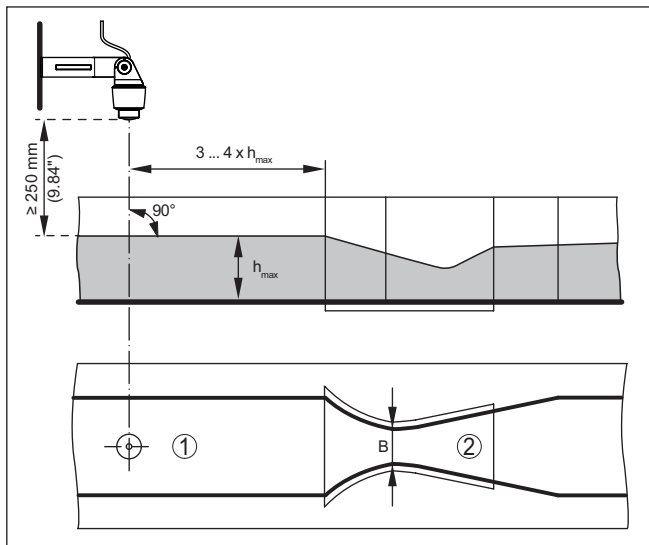
插图. 20: 用卡发基-文丘里槽来测量流量: h_{\max} = 水槽的最大灌装量; B = 水槽的最大收缩率
