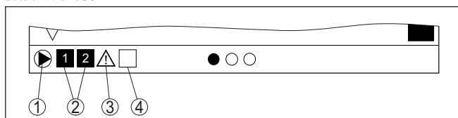
插图. 14: 泵控制激活情况下的显示器状态条距举例
