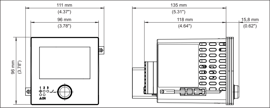
插图. 21: VEGAMET 341 的尺寸
