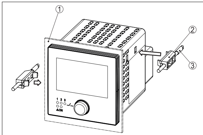
插图. 3: 安装在控制板内
