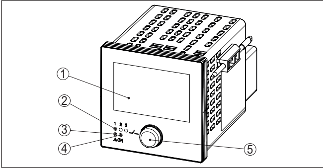
插图. 7: 显示和调整元件 1 液晶显示器 2 继电器状态显示 3 故障报告状态显示 4 运行就绪状态显示 5 用于操作菜单的旋钮/按钮
