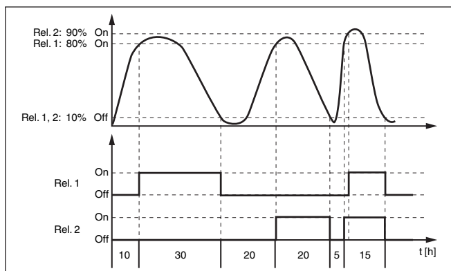
插图. 15: 示例: 泵控制器 2
