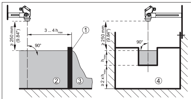
插图. 19: 用矩形槽测量流量: h_{\max} = 矩形槽的最大注水高度
