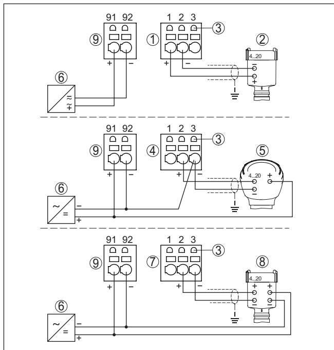
插图. 5: 两线制-/三线制-/四线制仪表的连接 (有源/无源)
