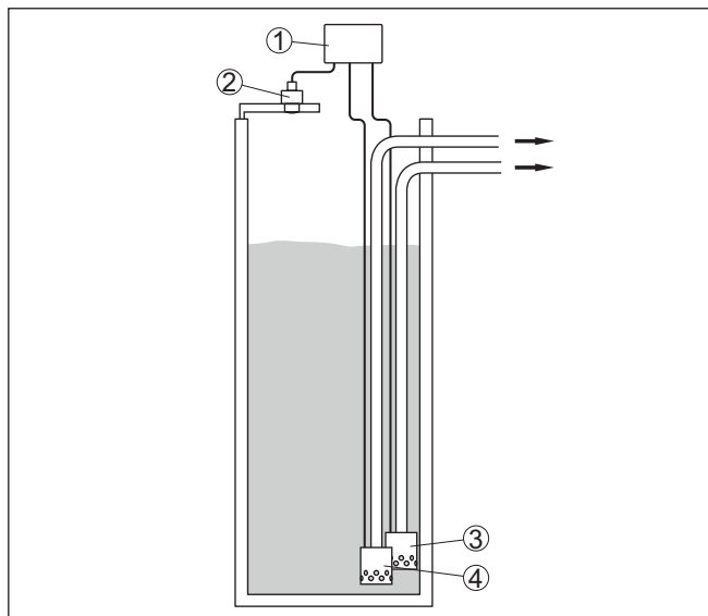
插图. 13: 泵站举例：在流入沟口控制泵
