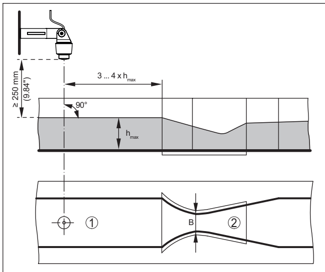
插图. 20: 用卡发基-文丘里槽来测量流量: h_{\max} = 水槽的最大灌装量; B = 水槽的最大收缩率
