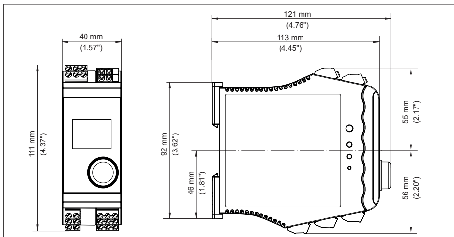
插图. 21: VEGAMET 142 的尺寸
