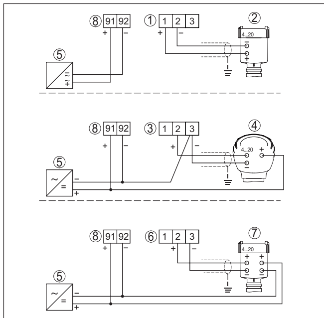
插图 4: 两线制-/三线制-/四线制仪表的连接 (有源/无源)
