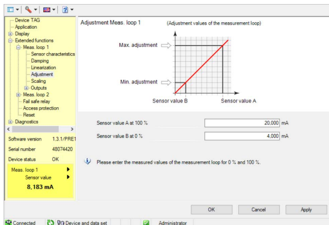
插图. 10: 一个 DTM 视图举例 - 调整
