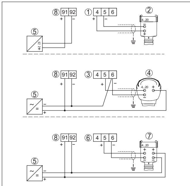
插图. 5: 两线制-/三线制-/四线制仪表的连接 (有源/无源)
