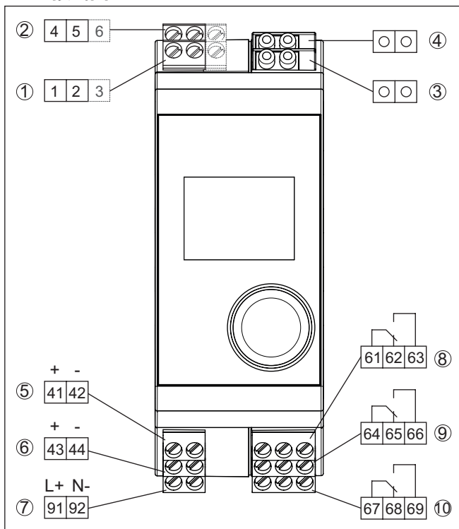
插图. 3: VEGAMET 142 的接线图
