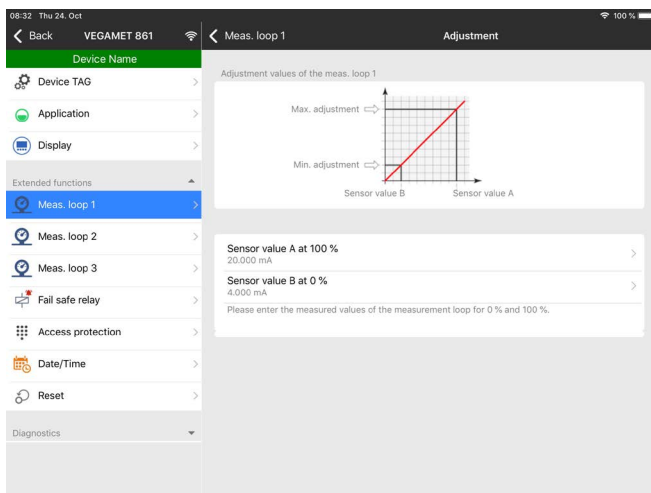
插图. 9: App 应用程序视图图举例 - 调试 调整
