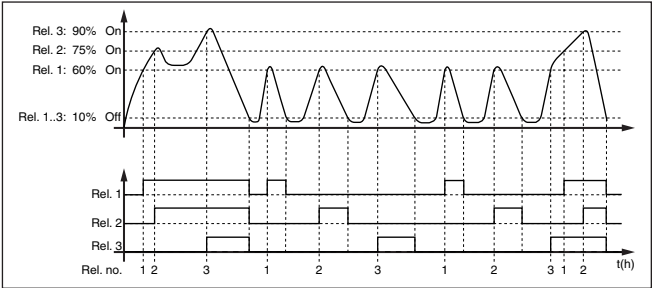
插图. 16: 泵控制器 4 的接通表现
