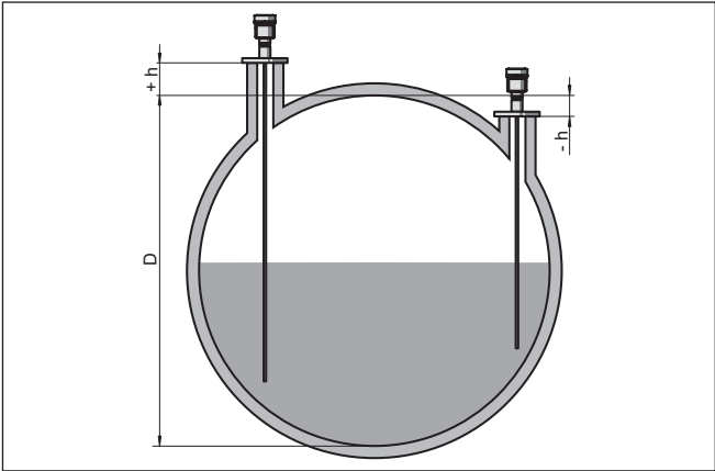
插图. 20: 容器高度和管接头修正值
