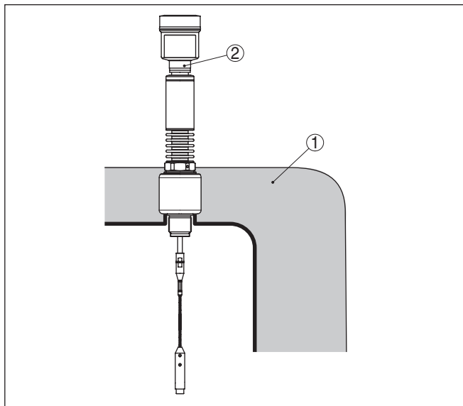
插图. 10: 将仪表安装在绝缘容器上。
