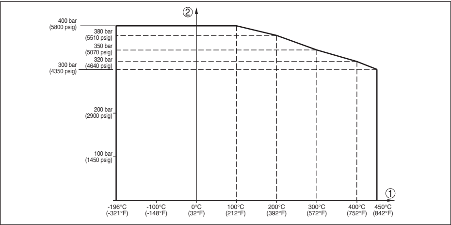
插图. 40: 过程压力 - 过程温度 ( -196 ... +450 °C/-321 ... +842 °F 型)
