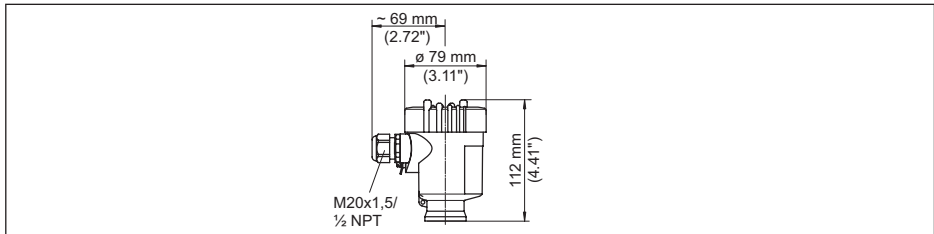
插图. 41: 采用防护等级为 IP66/IP67 的外壳版本 (内装显示和调整模块后, 外壳高度增加了 9 mm/0.35 in)
