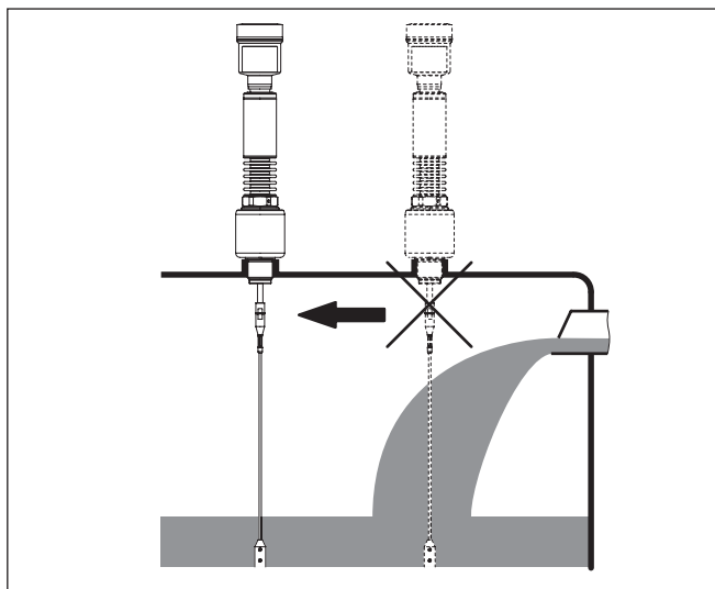
插图. 7: 流入介质时安装传感器
