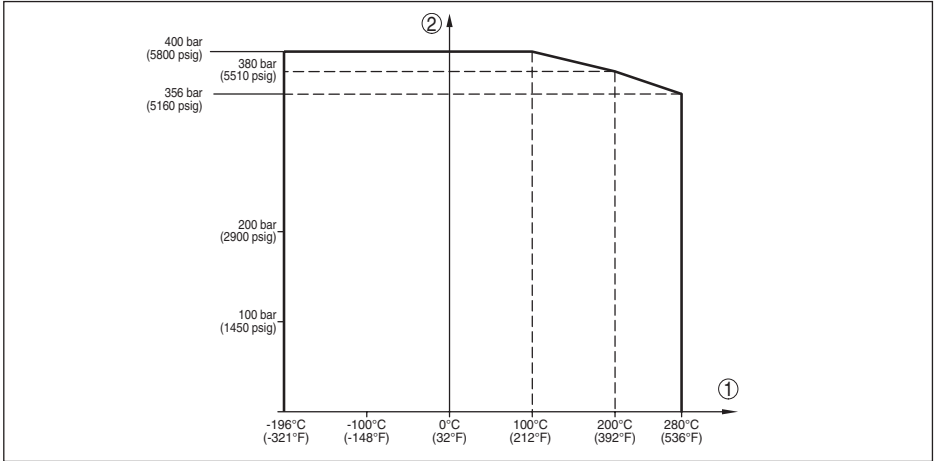
插图. 39: 过程压力 - 过程温度 ( -196 ... +280 °C/-321 ... +536 °F 型)
