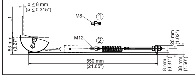
插图. 12: 绳型仪表的系紧装置
