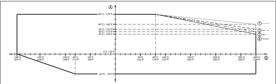
插图. 37: 环境温度 - 过程温度，标准型
