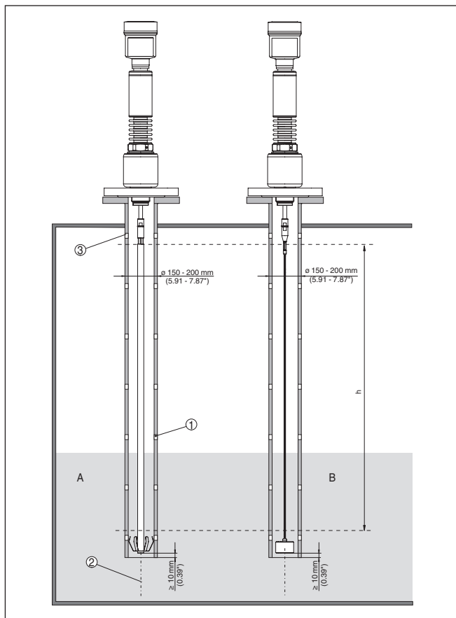
插图. 9: 安装在一根立管中
