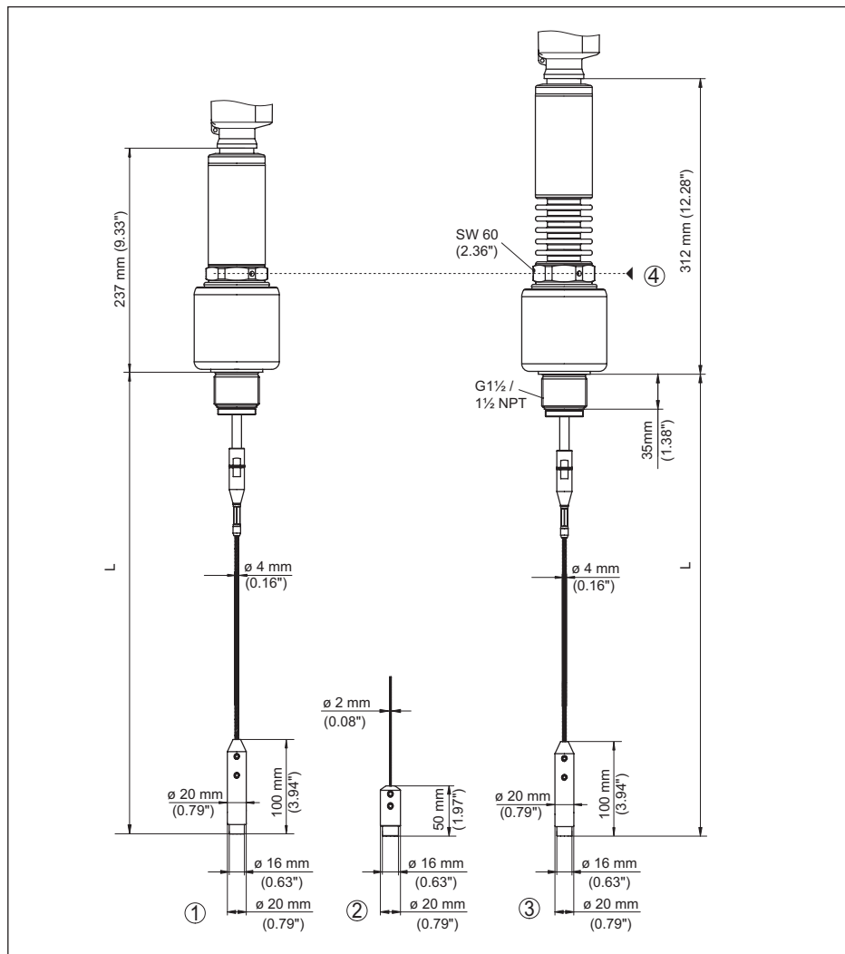
插图. 46: VEGAFLEX 86, 带重锤的绳型 (所有重锤都带有用于环首螺钉的螺纹孔, M8)
