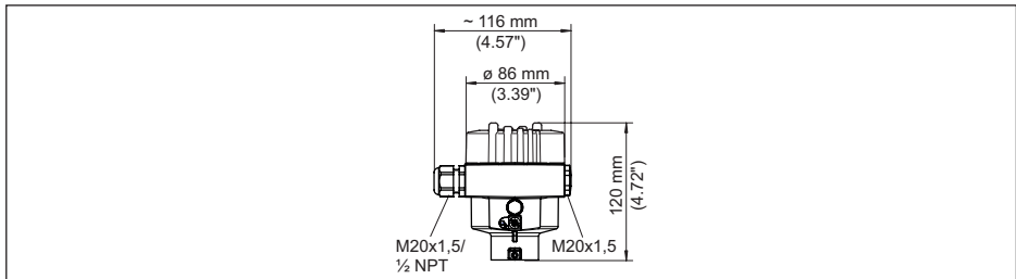
插图. 42: 防护等级达 IP66/IP68 (0.2 bar) 的壳体版本, (内装显示和调整模块后, 壳体高度增加了18 mm/0.71 in)
