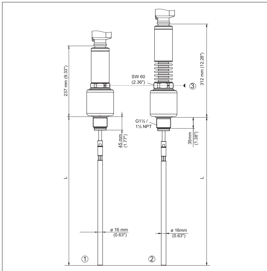
插图. 48: VEGAFLEX 86, 螺纹型
