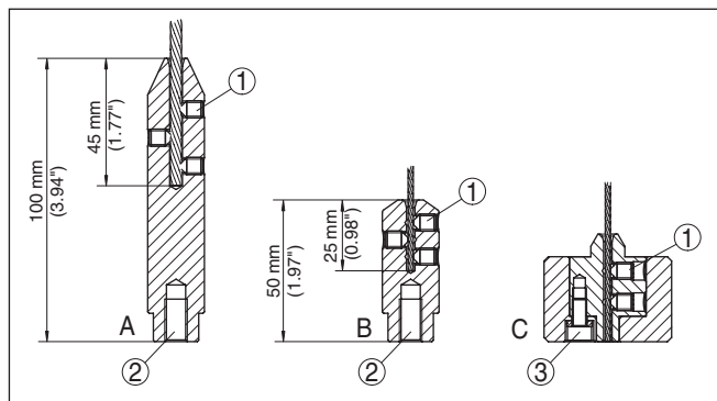
插图. 30: 裁短绳型测量探头
