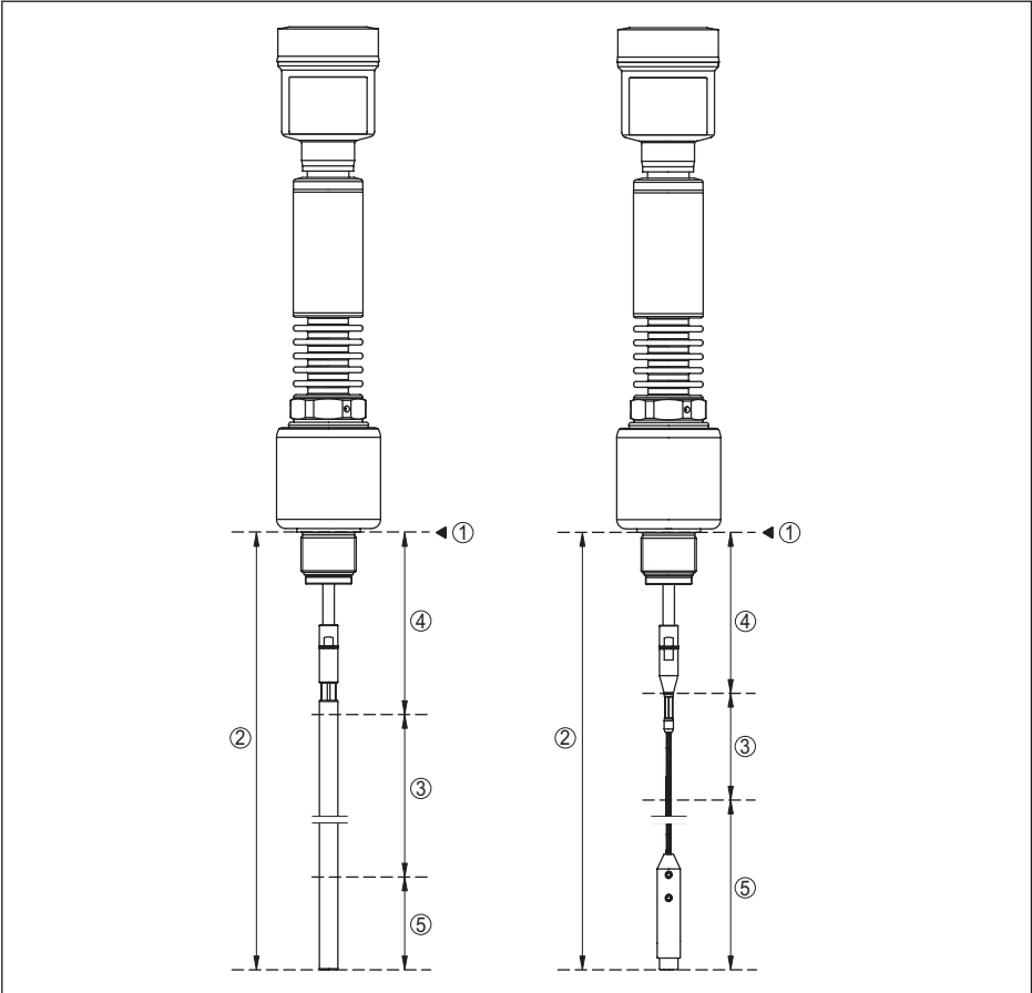
插图. 31: VEGAFLEX 86 的量程
