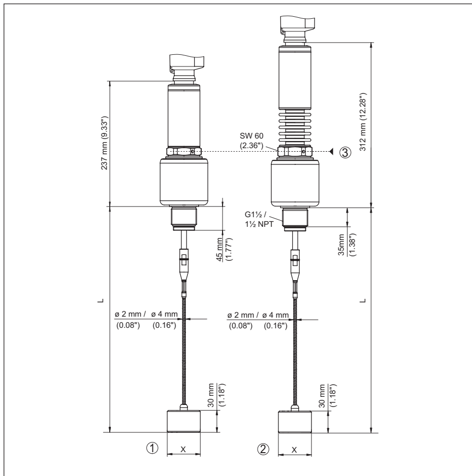
插图. 47: VEGAFLEX 86, 带对中重量的螺纹型
