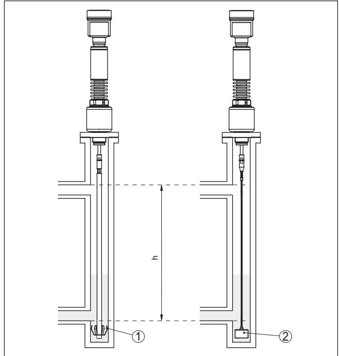
插图. 8: 星状对中垫片或定心锤的位置
