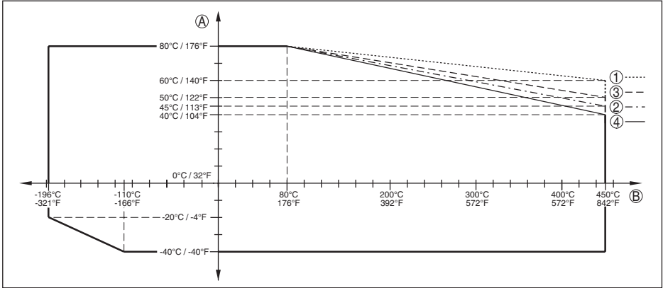
插图. 38: 环境温度 - 过程温度, 标准型
