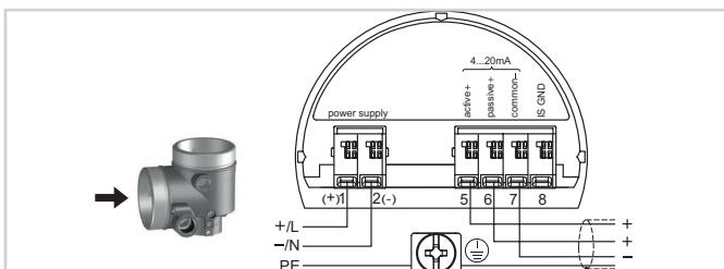
双腔式外壳的接线腔 - 电网供电
