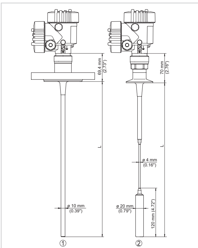
VEGAFLEX 83
