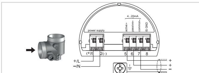
双腔式外壳的接线腔 - 小电压供电
