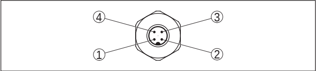
插图. 14: 察看 M12 x 1-接插器
