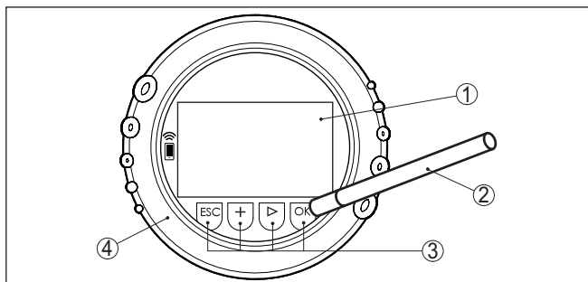
插图 17: 显示和调整元件 - 拥有磁笔操作功能
