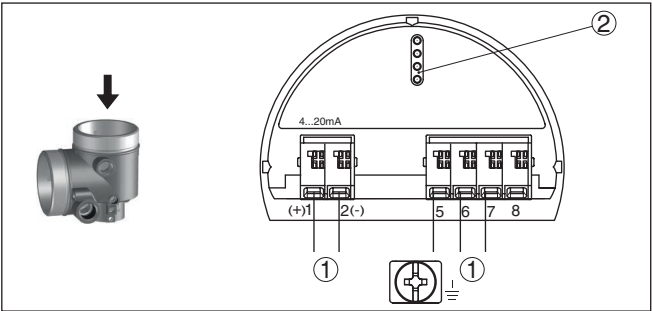
插图. 10: 双腔式外壳的电子部件腔 1 与接线腔的内部连接 2 用于显示和调整模块或接口适配器
