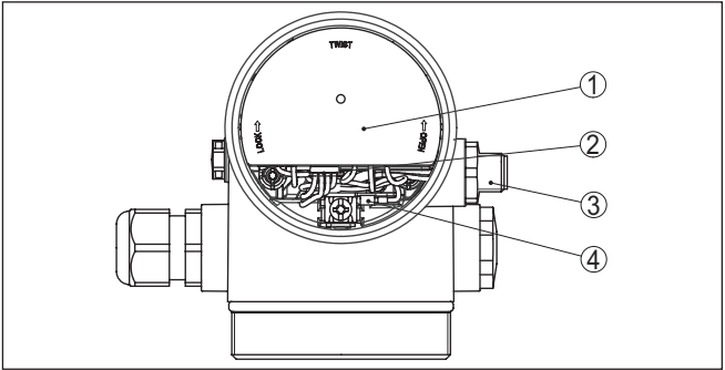
插图. 13: 目检带有与外部显示和调整单元相连接的 VEGADIS-Adapter 的电子部件腔
