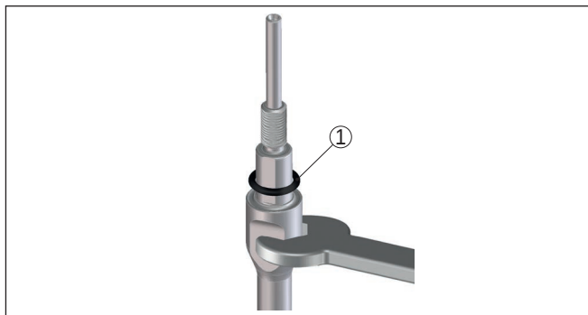
插图. 28: 拆下测量棒
