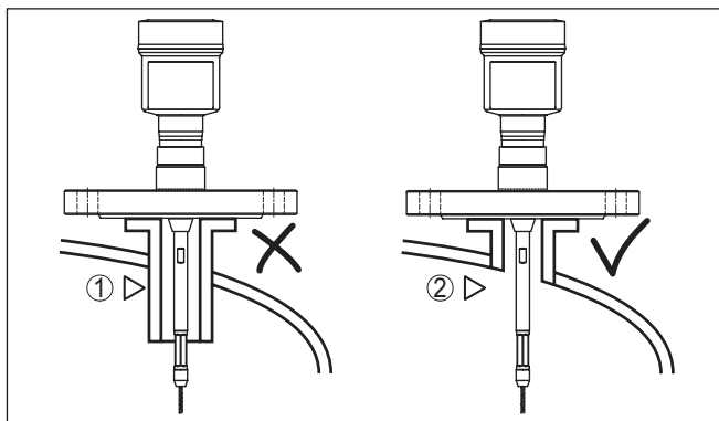
插图. 6: 齐平地安装管接头
