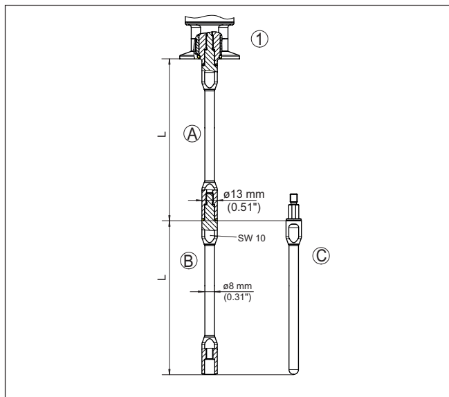
插图. 37: 直径为 \varnothing 8 \text{ mm} (0.315 in) 的加长型棒
