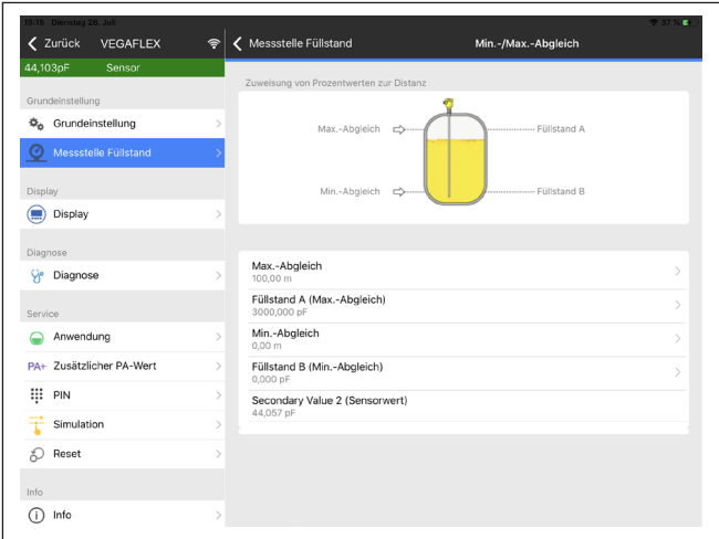
插图. 20: 应用程序视图举例 - 调试 传感器调整
