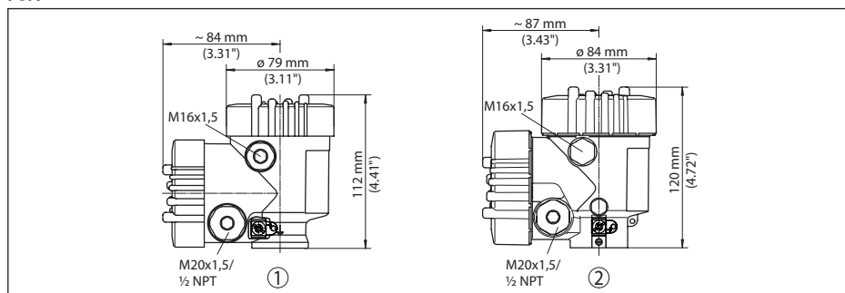
插图 34: VEGAFLEX 83 带内装的显示和调整模块, 能将壳体高度增加 9 mm (0.35 in)
