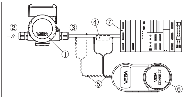
插图. 22: 通过 HART 将电脑与信号线路相连
