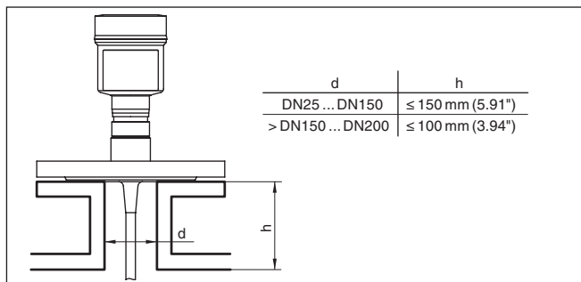
插图. 5: 安装用管接头
