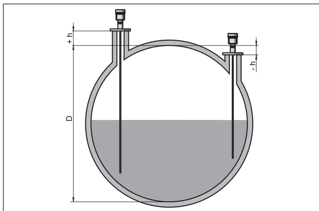
插图. 18: 容器高度和管接头修正值
