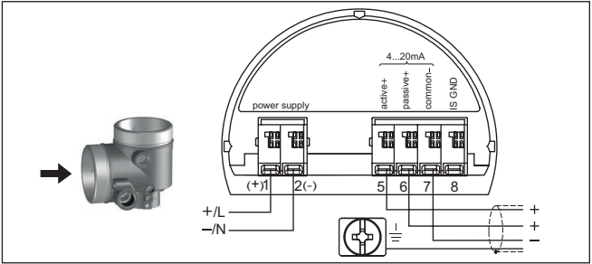
插图. 12: 小电压供电时双腔式外壳的接线腔
