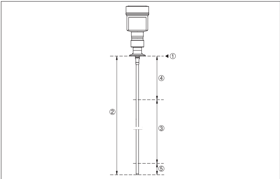
插图. 30: VEGAFLEX 83 的量程
