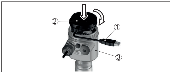
插图. 21: 通过接口适配器将电脑直接与仪表相连
