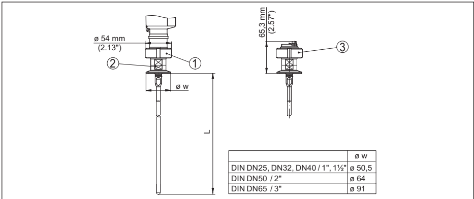
插图. 36: VEGAFLEX 83, 棒型 \varnothing 8 mm (0.315 in), 经抛光 - 自封闭式
