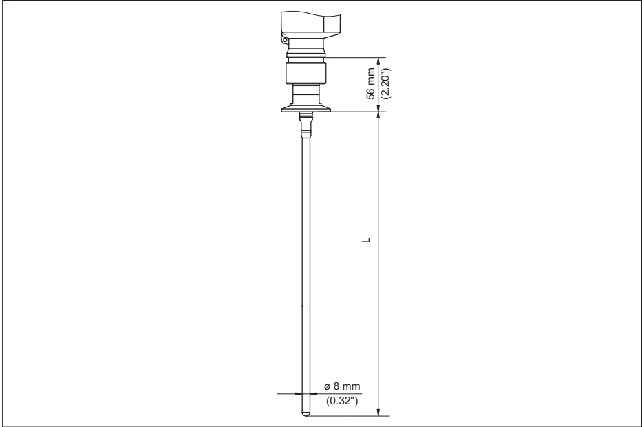
插图. 35: VEGAFLEX 83, 棒型 \varnothing 8 mm (0.315 in), 经抛光
