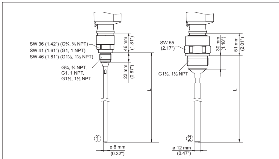
插图. 47: VEGAFLEX 81, 螺纹型
