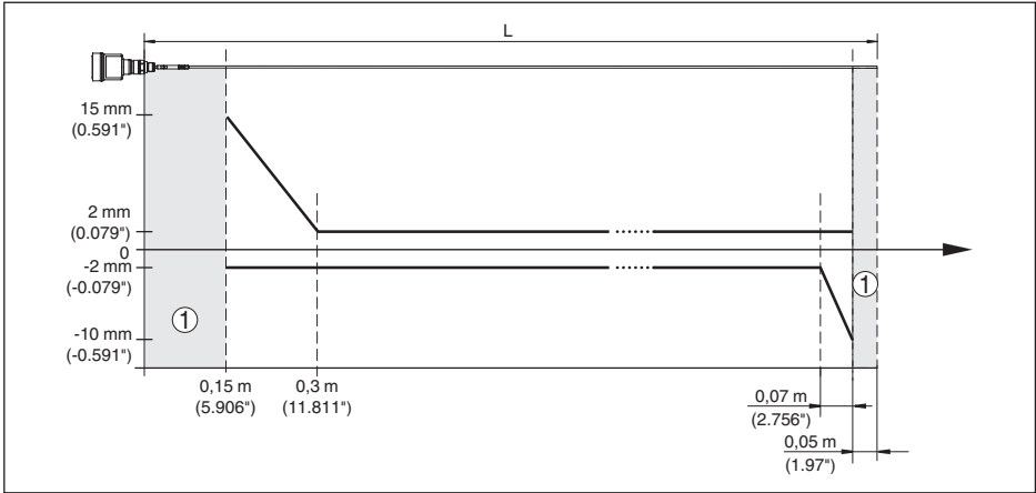
插图. 32: 棒型 VEGAFLEX 81 在介质“油”中的测量偏差
