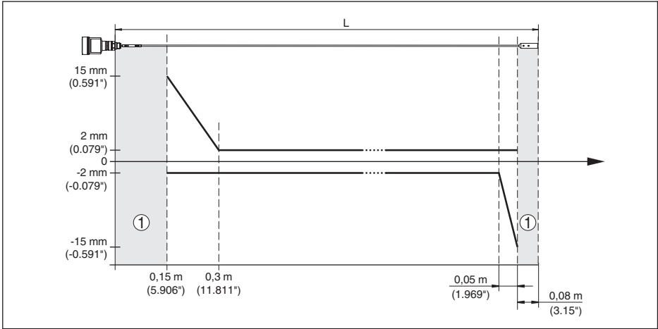
插图. 34: 绳型 (ø 2 mm/0.079 in) VEGAFLEX 81 在介质“油”中的测量偏差
