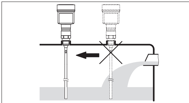
插图. 7: 流入介质时安装传感器
