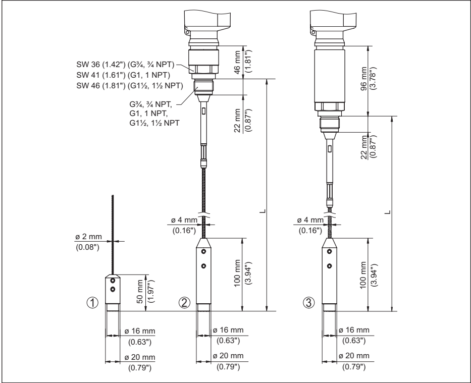
插图. 45: VEGAFLEX 81, 带重锤的绳型 (所有重锤都带有用于环首螺钉的螺纹孔, M8)
