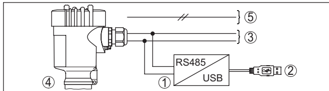
插图. 23: 电脑通过接口适配器与 RS 485 电线相连接
