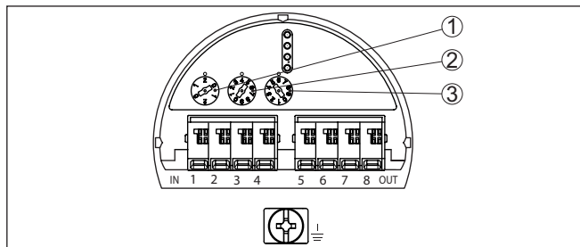
插图. 15: 地址选择开关
