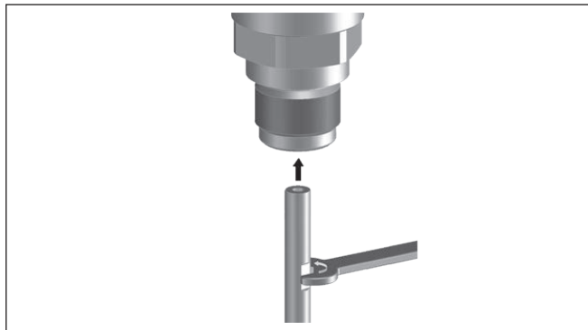
插图. 28: 更换测量绳或测量棒
