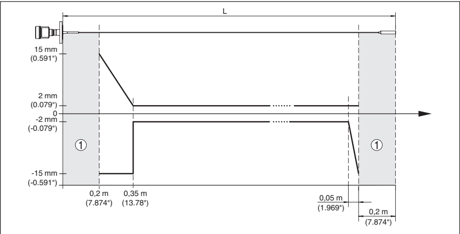
插图. 37: 在介质油中, 绳型 VEGAFLEX 81 (ø 4 mm/0.157 in, 经 PFA 涂层) 的测量偏差
