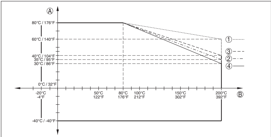
插图. 39: 环境温度 - 过程温度、带有温度连接元件的选型
