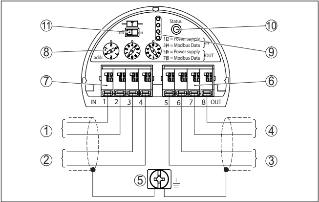
插图. 13: 电子部件腔 - 菊花链接口
