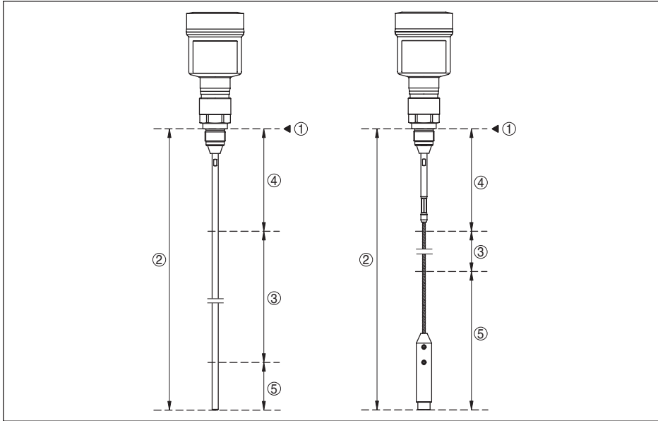
插图. 30: VEGAFLEX 81 的量程
