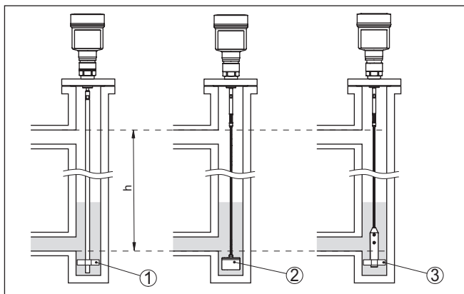
插图. 8: 安装在一根旁路管中 - 星形对中垫片或定心锤的位置
