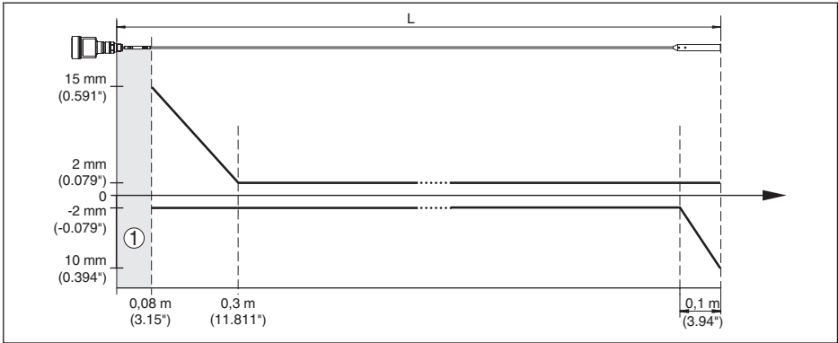
插图. 33: 绳型 VEGAFLEX 81 在介质“水”中的测量偏差
