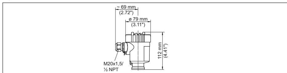
插图. 40: 采用防护等级为 IP66/IP67 的外壳版本 (内装显示和调整模块后, 外壳高度增加了 9 mm/0.35 in)
