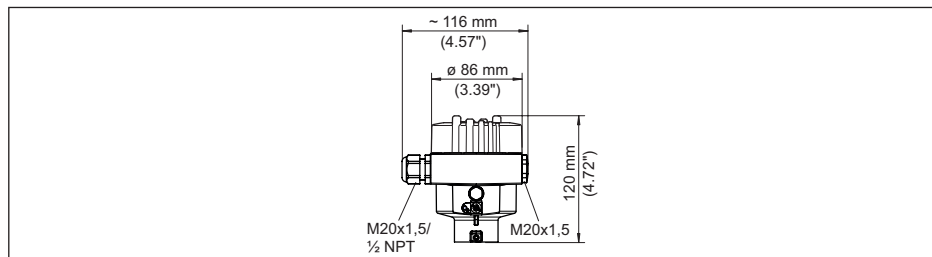
插图. 41: 防护等级达 IP66/IP68 (0.2 bar) 的壳体版本, (内装显示和调整模块后, 壳体高度增加了18 mm/0.71 in)
