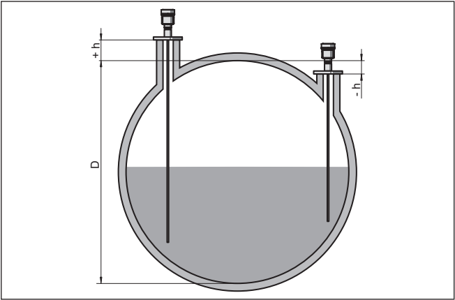
插图. 19: 容器高度和管接头修正值
