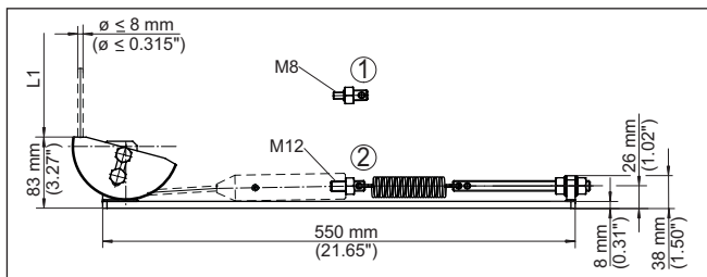
插图. 11: 绳型仪表的系紧装置
