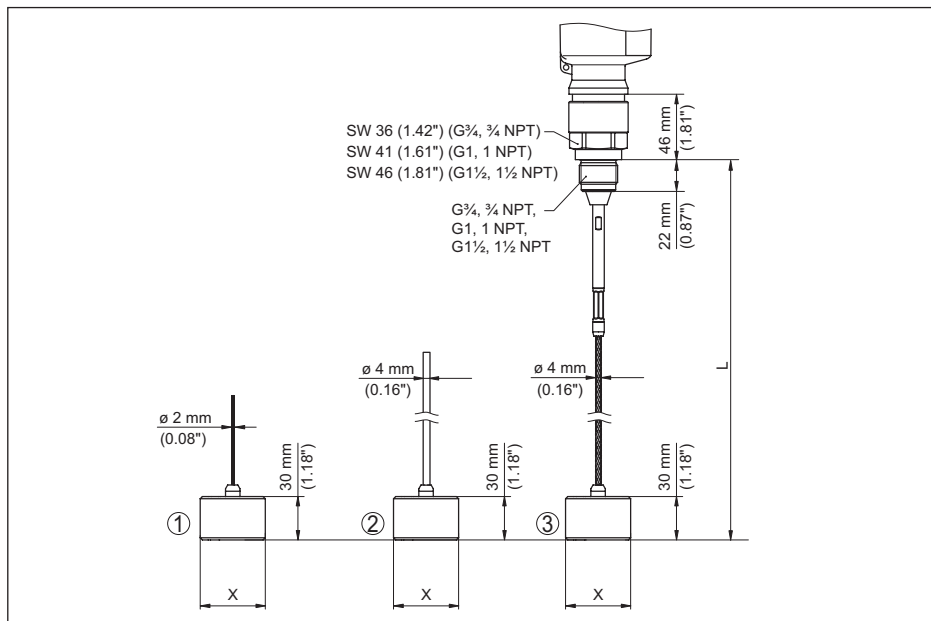
插图. 46: VEGAFLEX 81, 螺纹型
