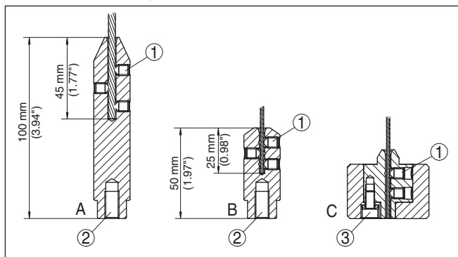
插图. 29: 裁短绳型测量探头
