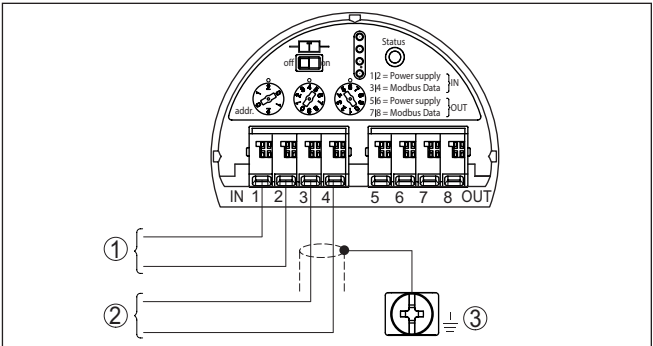
插图. 14: 电子部件腔 - 与短线相连接
