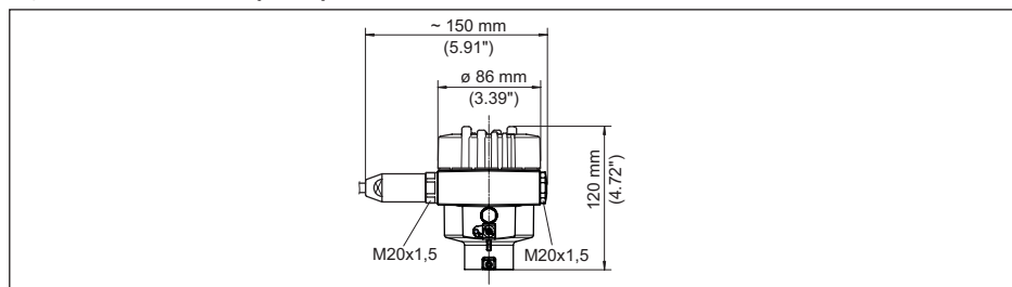
插图. 42: 防护等级达 IP66/IP68 (1 bar) 的壳体版本, (内装显示和调整模块后, 壳体高度增加了18 mm/0.71 in)
