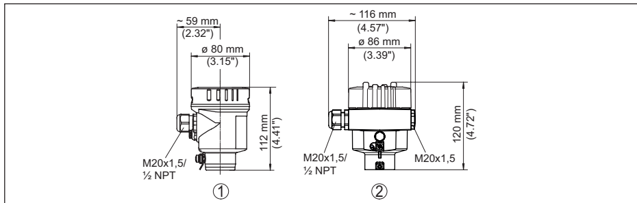
插图. 43: 采用防护等级达 IP66/IP68 (0.2 bar) 的壳体版本, (内装显示和调整模块后, 壳体高度增加了18 mm/0.71 in)
