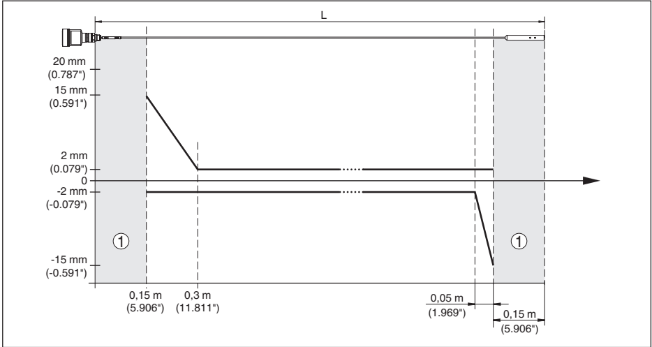
插图. 35: 绳型 ( \varnothing 4 \text{ mm}/0.157 \text{ in} ) VEGAFLEX 81 在介质"油"中的测量偏差
