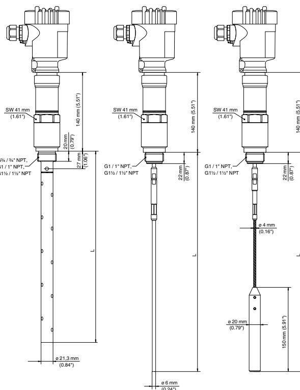
VEGAFLEX 66 - 螺纹型
