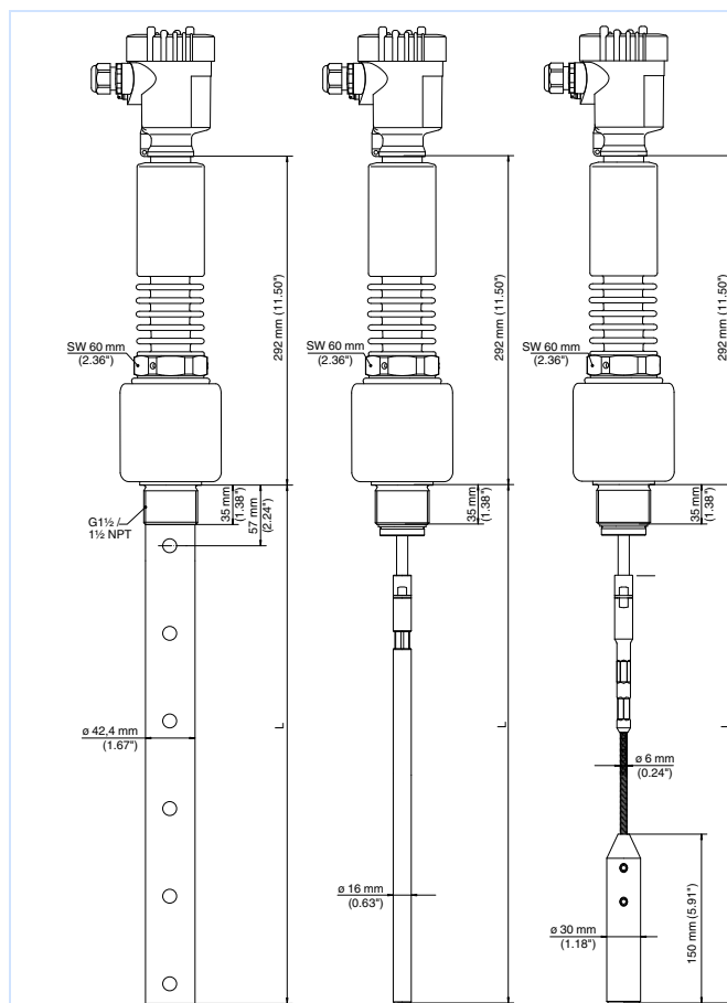
VEGAFLEX 66 – 螺纹型
