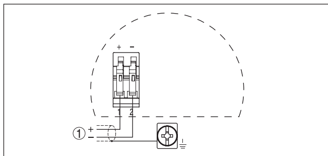
插图. 9: 接线图
