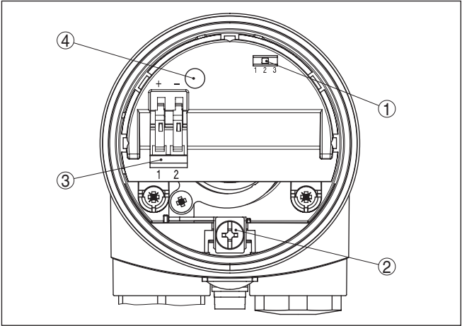
插图. 12: 电子部件 - 两线制输出口
