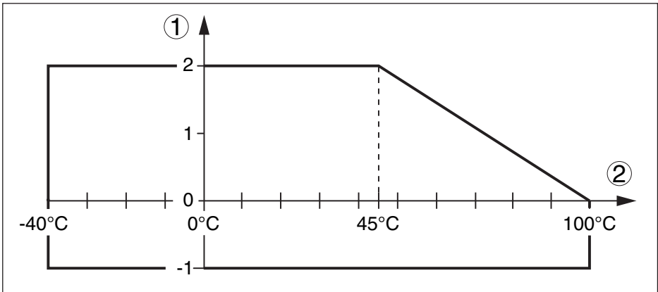
插图. 18: 过程压力 - 过程温度 (用 PTFE 制成的法兰)
