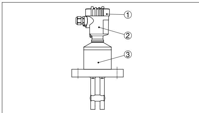
插图. 1: VEGACAP 69 - 带有塑料壳体的双棒式测量探针
