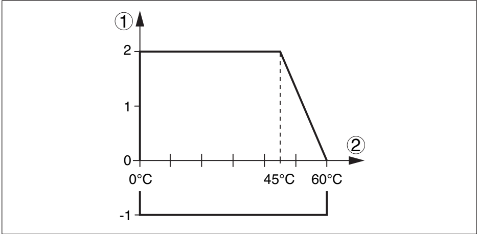
插图. 19: 过程压力 - 过程温度 (用 PP 制成的法兰)
