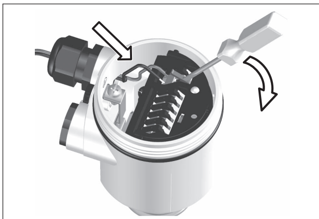
插图. 6: 接线步骤5和6
