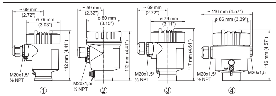
插图. 18: 外壳选型
