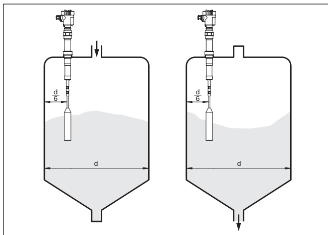
插图. 6: 在中央进行充填和排空
