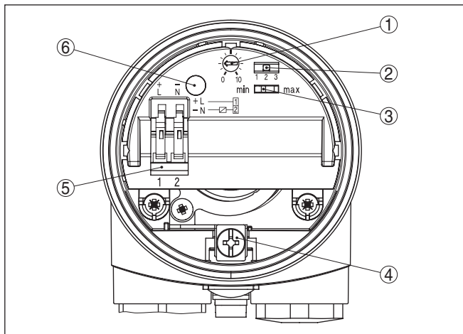
插图. 10: 电子部件腔和接线腔
