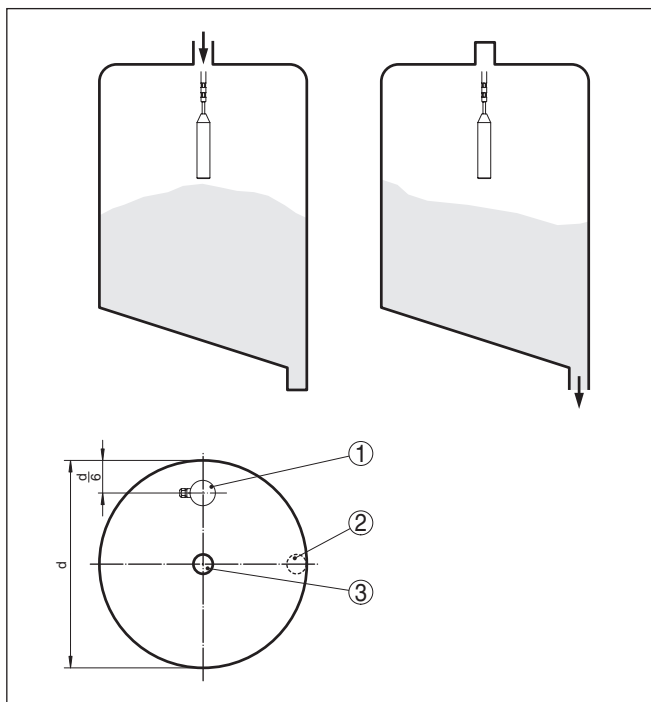
插图. 7: 在中央充填，在侧面排空
