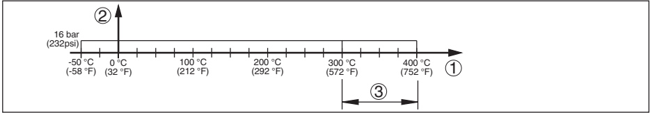
插图. 17: 过程温度 - 过程压力
