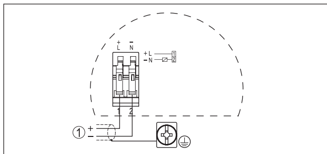
插图. 11: 接线图
