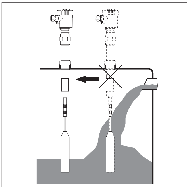
插图. 5: 流入的介质
