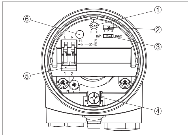
插图. 12: 电子插件 - 无接触式开关
