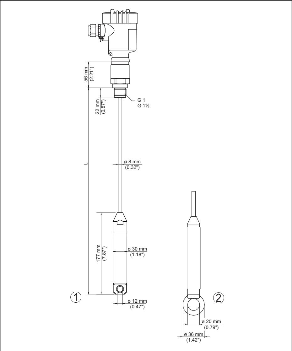
插图. 22: VEGACAP 66, 螺纹型 G1 (ISO 228 T1)
