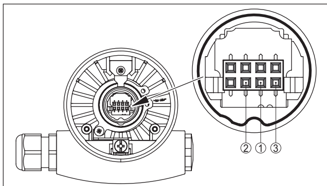
插图. 16: 检查测量探头内的电阻
