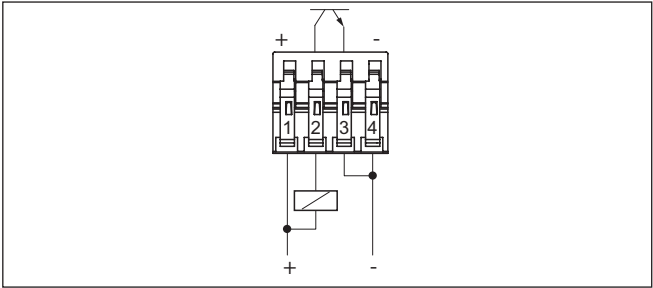
插图. 12: NPN 工作方式
