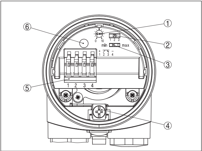
插图. 15: 电子部件 - 晶体管输出口
