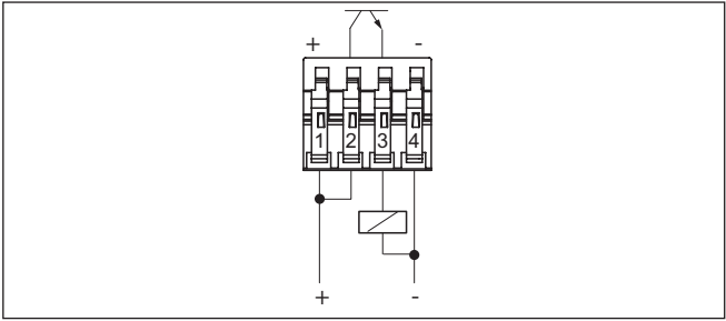
插图. 13: PNP 工作方式
