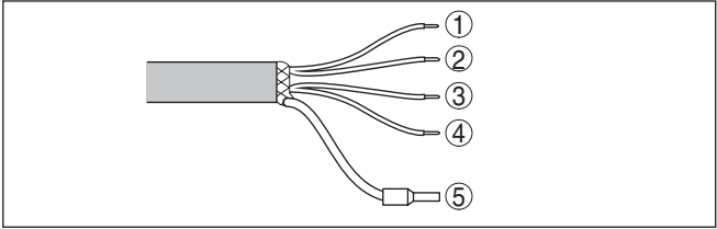
插图. 14: 连接电缆的芯线分布情况。芯线的编号对应于仪表的接线端子。
