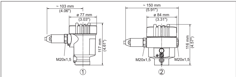
插图. 21: 外壳型式所采用的保护等级为 IP66/IP68 (1 bar)
