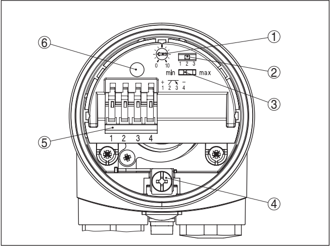
插图. 10: 电子部件腔和接线腔
