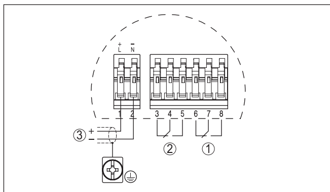
插图. 11: 接线图
