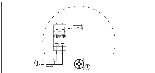
插图. 12: 接线图
