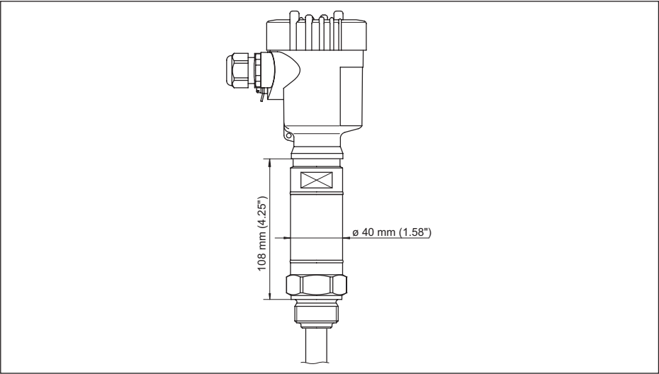
插图. 21: 温度连接元件
