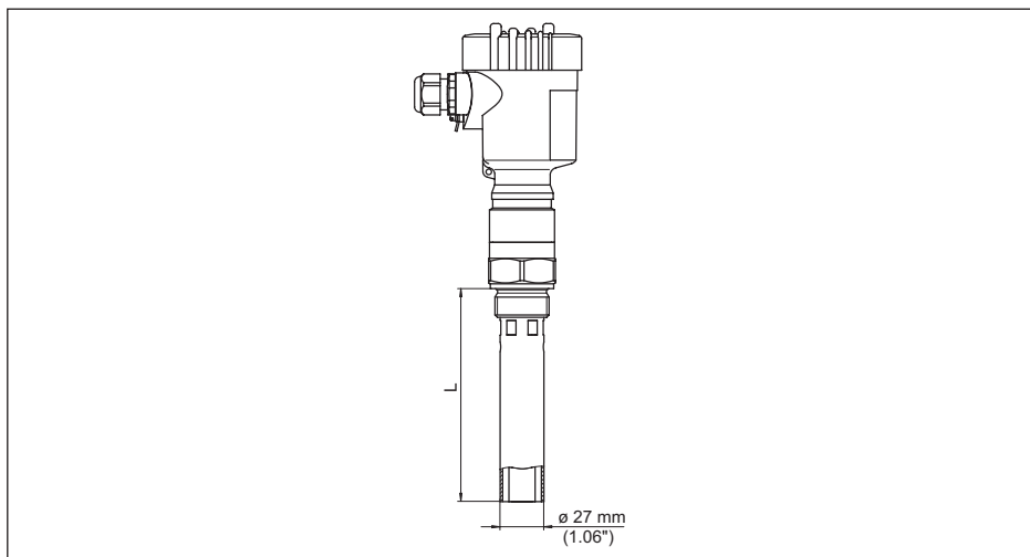
插图. 23: VEGACAP 62, 封管, 比如在介电常数较小时或进行线性化时
