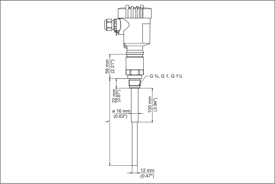
插图. 20: VEGACAP 62, 螺纹型 G1 (ISO 228 T1)
