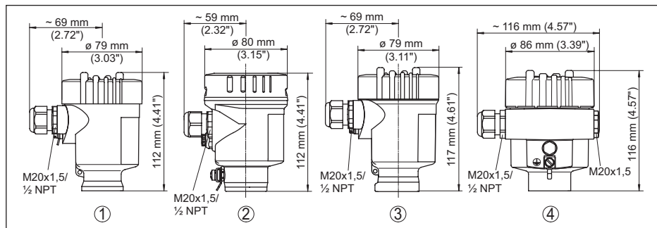
插图. 19: 外壳选型
