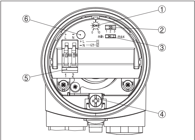
插图. 13: 电子插件 - 无接触式开关
