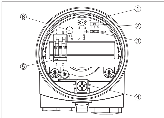
插图. 11: 电子部件腔和接线腔
