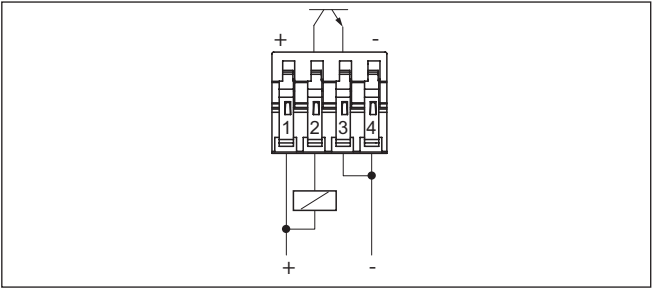
插图. 13: NPN 工作方式
