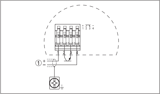
插图. 12: 接线图
