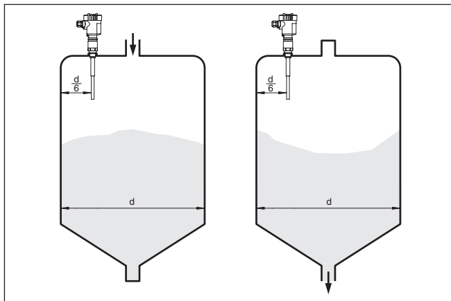
插图. 7: 在中央进行充填和排空
