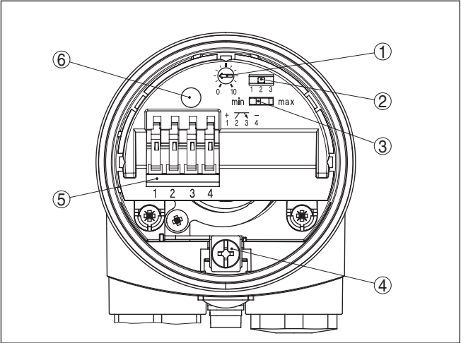
插图. 16: 电子部件 - 晶体管输出口
