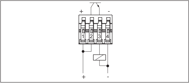
插图. 14: PNP 工作方式
