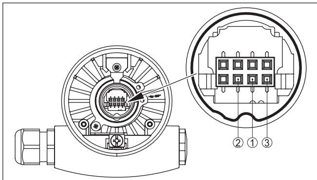
插图. 17: 检查测量探头内的电阻
