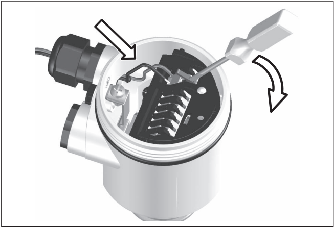
插图. 9: 接线步骤5和6
