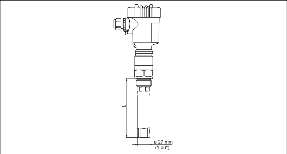
插图. 27: VEGACAP 62, 封管, 比如在介电常数较小时或进行线性化时
