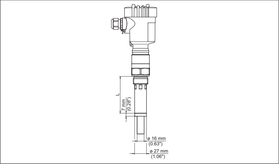
插图. 26: VEGACAP 62, 屏蔽管, 如用于防止冷凝水大量积聚
