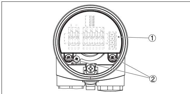
插图. 18: 拧松支撑螺钉
