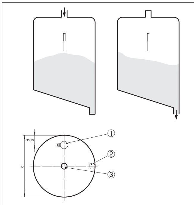
插图. 8: 在中央充填，在侧面排空
