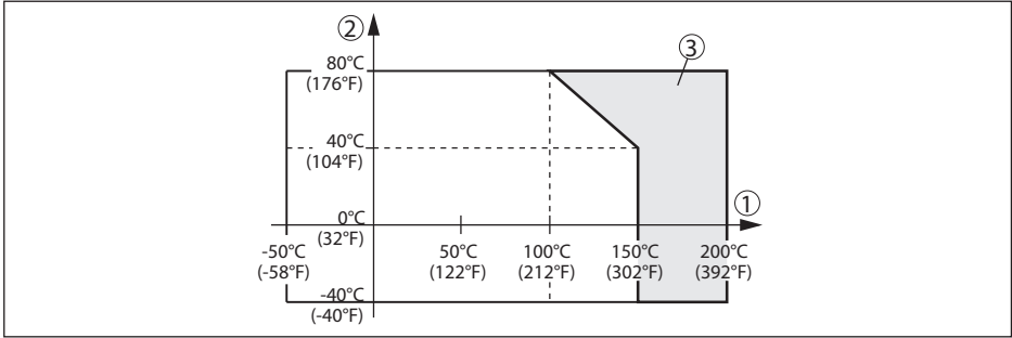
插图. 21: 环境温度 - 过程温度
