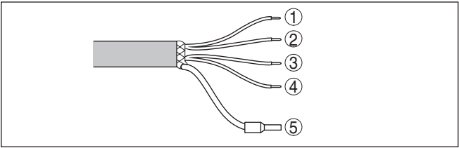
插图. 15: 连接电缆的芯线分布情况。芯线的编号对应于仪表的接线端子。
