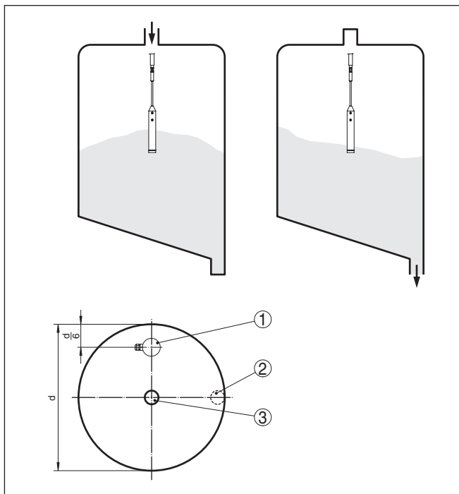
插图. 6: 在中央充填, 在侧面排空
