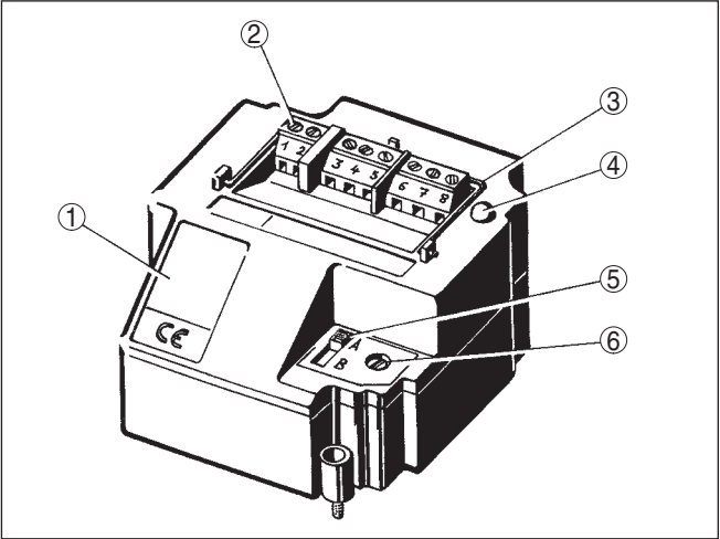
插图. 8: 带继电器输出电子的插件
