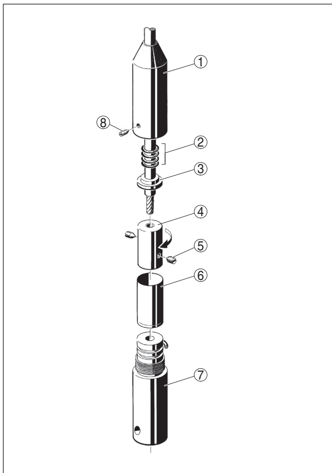
插图. 10: 缩短绳型测量探头
