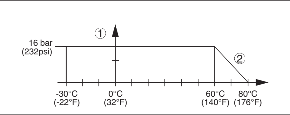
插图. 11: 过程压力 - 过程温度 - VEGACAP 35 带用铝制成的过程接头
