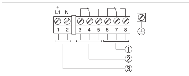
插图 7: 接线图
