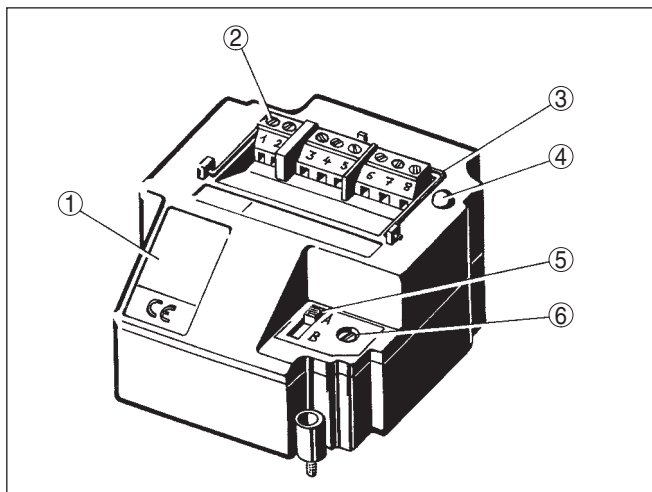
插图. 6: 带继电器输出电子插件
