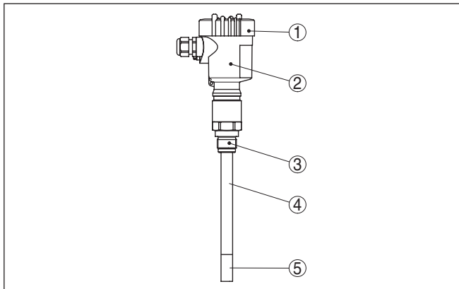
插图 1: VEGACAP 27，带塑料外壳
