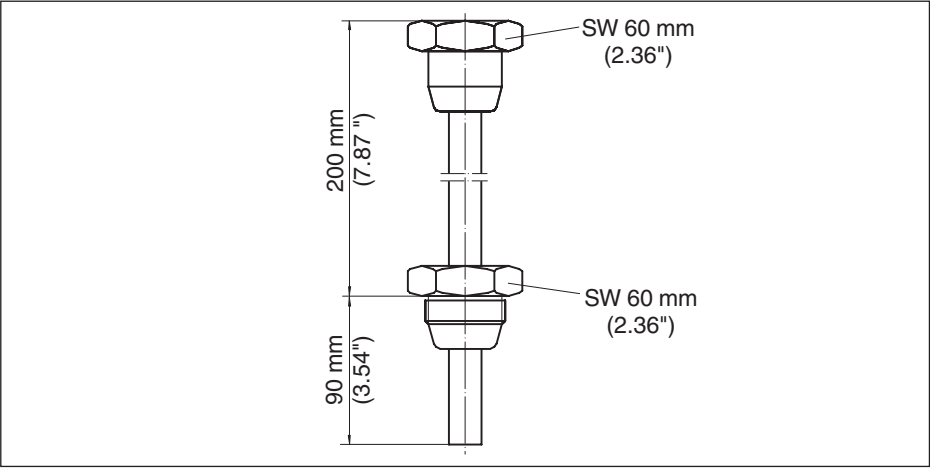
插图. 11: 温度连接件 (可选) 316L, 316Ti
