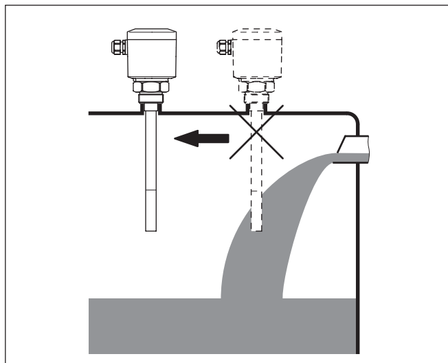
插图. 4: 流入的介质
