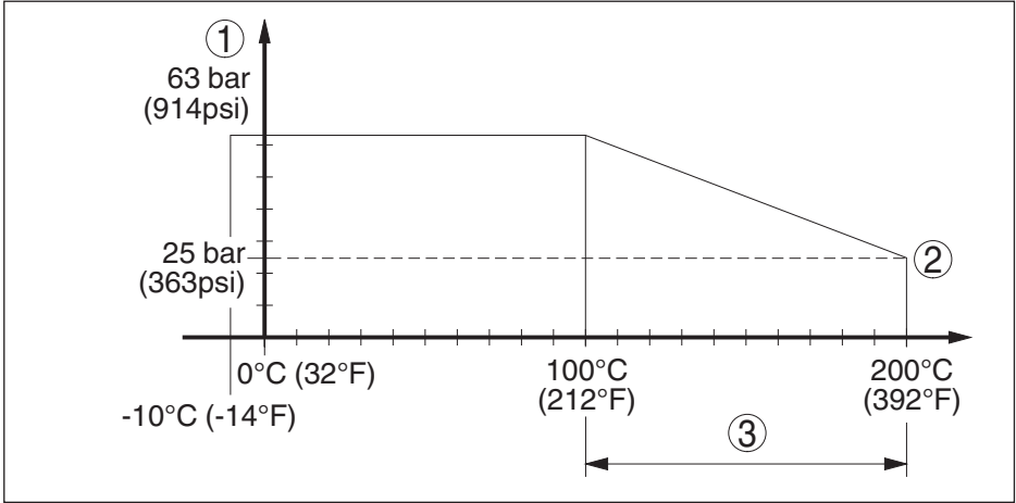
插图 8: 过程压力 - 过程温度 - VEGACAP 27 带有 316L 制成的过程接头
