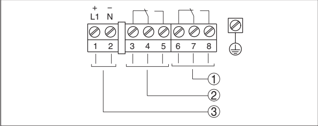
插图 5: 接线图
