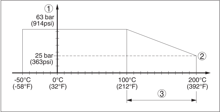
插图 9: 过程压力 - 过程温度 - VEGACAP 27 带有 316Ti 制成的过程接头
