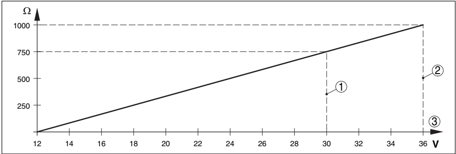
插图. 17: 供电电压图
