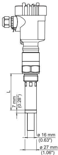
插图. 24: VEGACAL 65, 屏蔽管, 如用于防止冷凝水大量积聚
