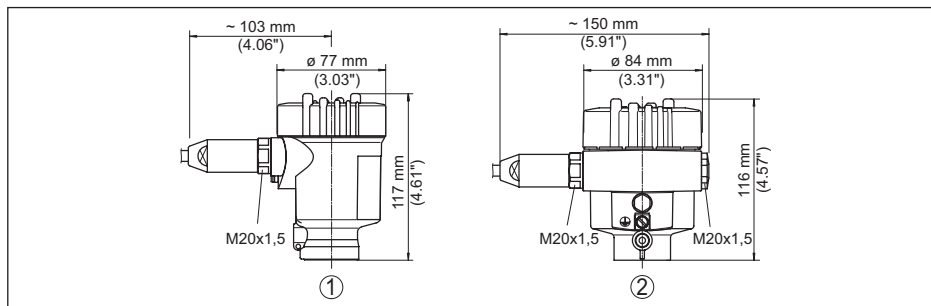
插图. 19: 外壳型式所采用的保护等级为 IP66/IP68 (1 bar)
