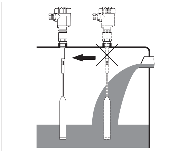
插图. 7: 流入的介质
