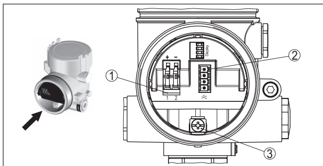
插图. 14: 双腔式外壳的接线腔
