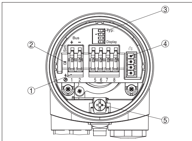
插图. 10: 单腔式外壳的电子部件和接线腔
