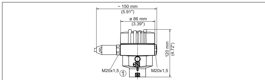
插图. 32: 采用防护等级达 IP66/IP68 (1 bar) 的壳体版本 (内装显示和调整模块后, 壳体高度增加了18 mm/0.71 in)
