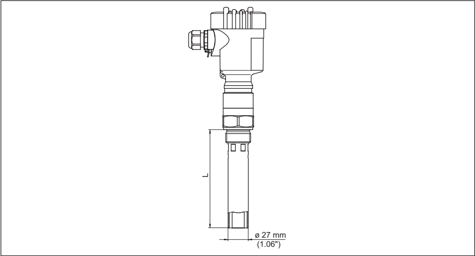
插图. 35: VEGACAL 63, 封管，比如在介电常数较小时或进行线性化时
