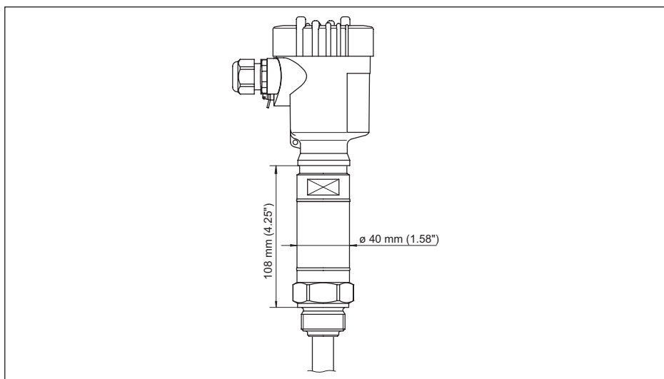
插图. 34: 温度连接元件
