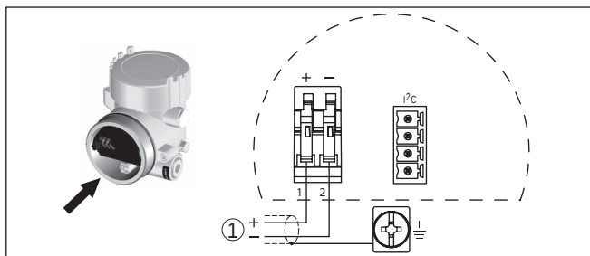
插图. 15: 双腔式外壳的接线图
