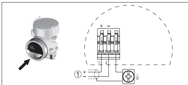
插图. 19: 防爆 (d ia) 型双腔式外壳的接线图
