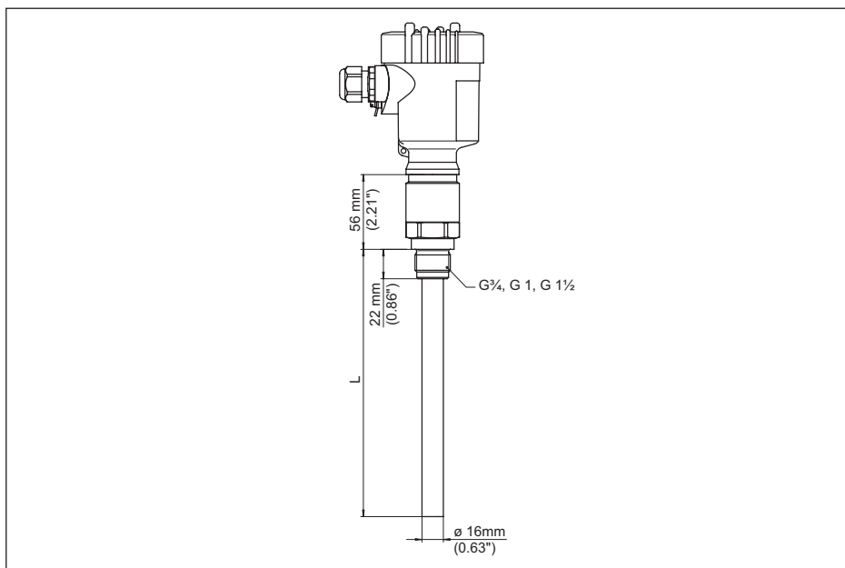
插图. 33: VEGACAL 63, 螺纹型 G1 (ISO 228 T1)
