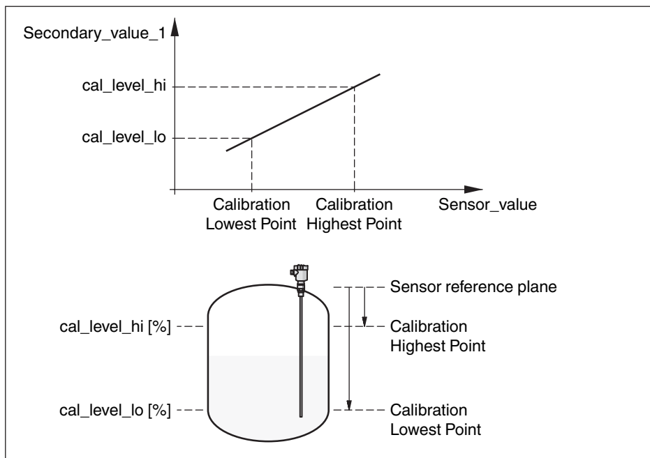
插图. 30: VEGACAL 63 的调整
