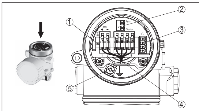
插图. 13: 双腔式外壳的电子部件腔
