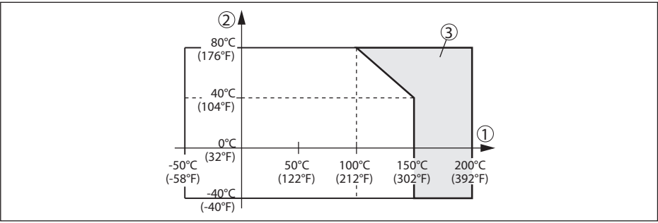
插图. 28: 环境温度 - 过程温度
