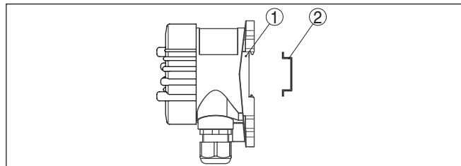
插图. 4: VEGABOX 03 带有塑料壳体，适合于安装在支撑轨道上
