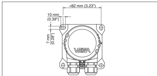
插图. 3: 安装在墙体上时 VEGABOX 03 的钻孔尺寸
