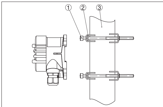
插图. 6: VEGABOX 03 用于安装在管件上
