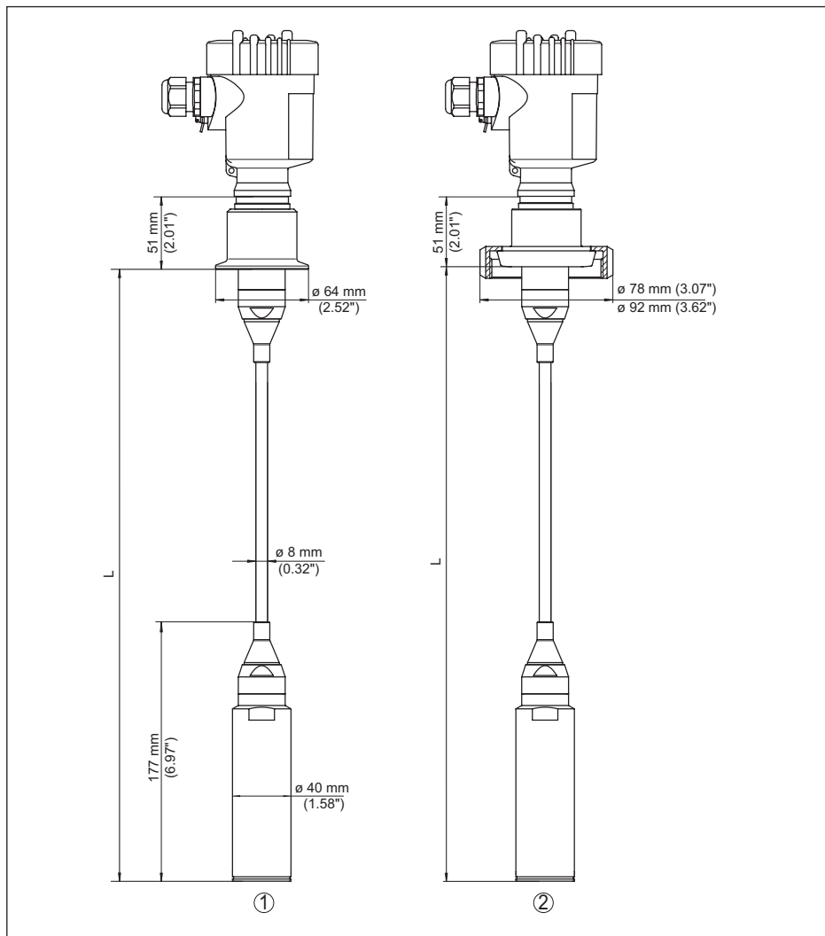
插图. 31: VEGABAR 87, 无菌接口
