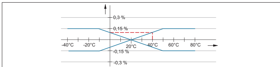
插图. 26: F_a 通过电流输出的热变化量, 在此例中 = 0.1 %
