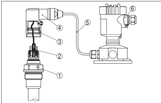
插图. 22: IP68 型 VEGABAR 87, 25 bar 及侧面电缆出口, 外部壳体
