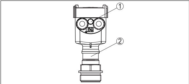
插图. 7: 过滤元件的位置 - 气密孔
