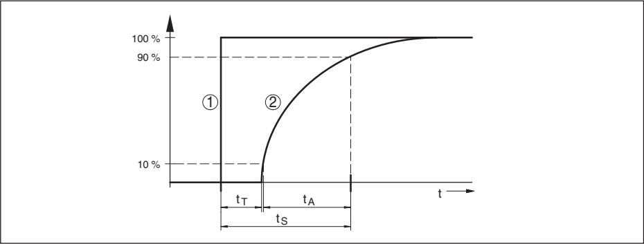
插图. 23: 在出现过程值跳跃式变化时的表现。t T : 死亡时间; t A : 上升时间; t S : 跳跃式回应时间
