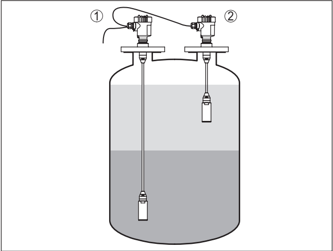
插图. 1: 用于测量分离层的电子差压举例
