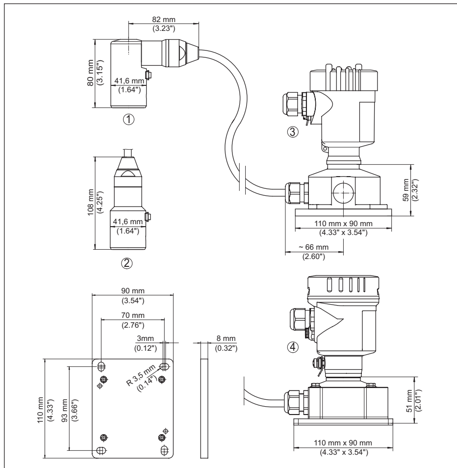
插图. 28: VEGABAR 87, IP68 型, 带外部壳体
