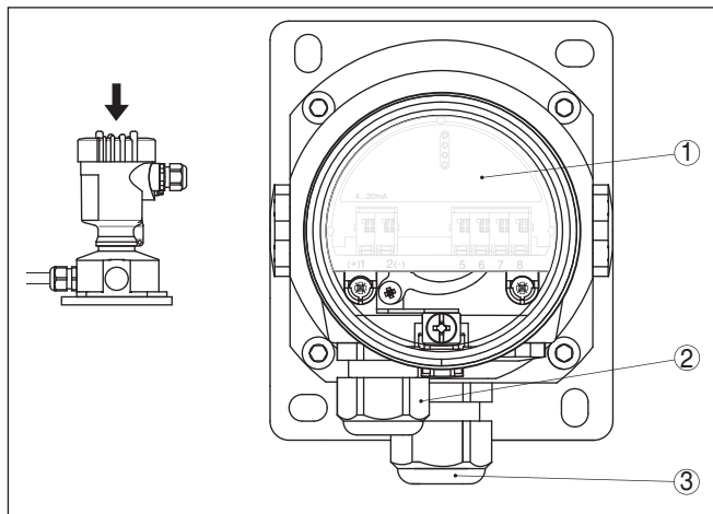
插图. 17: 电子部件腔和接线腔
