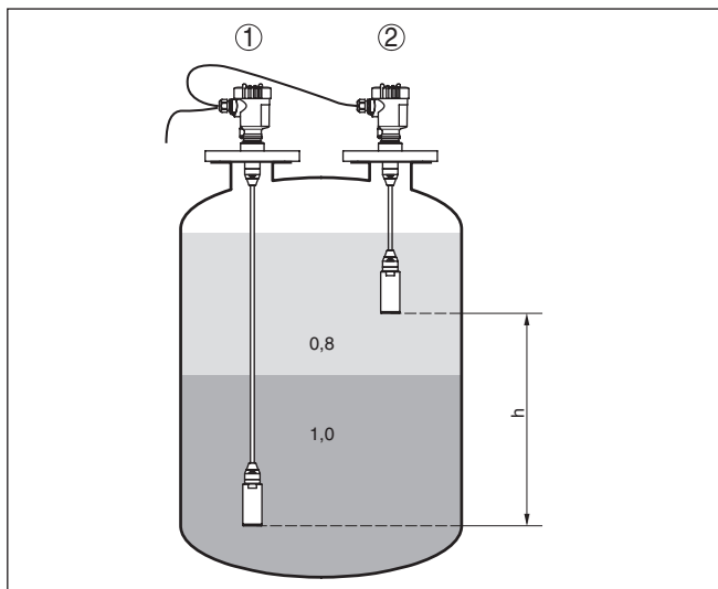
插图. 10: 测量分离层时的测量分布, h = 在两个测量点之间的距离
