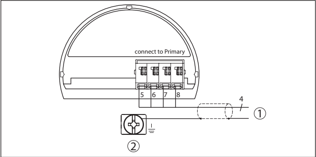
插图. 15: 从机接线图 VEGABAR 87
