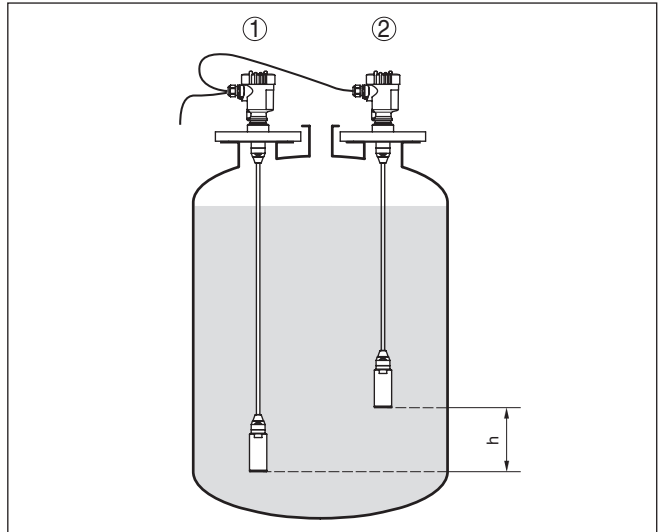
插图. 12: 在密度补偿式物位测量时的测量布局, h = 在两个测量点之间的距离
