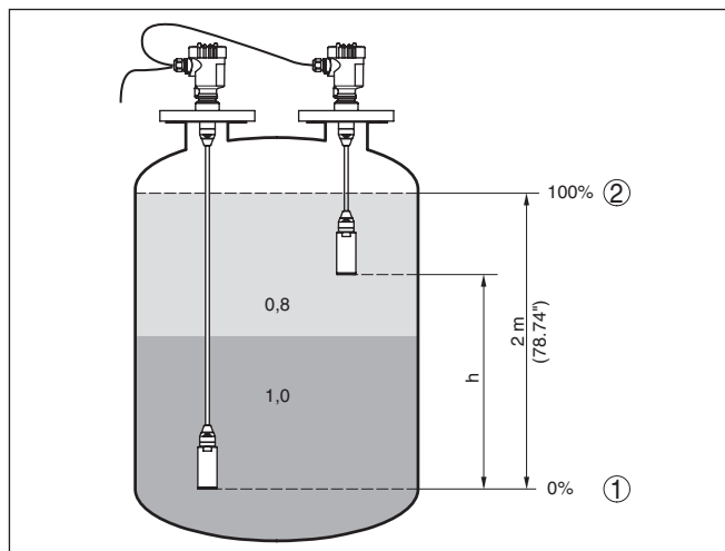
插图. 21: 界面测量时最小/最大调整的参数设置举例
