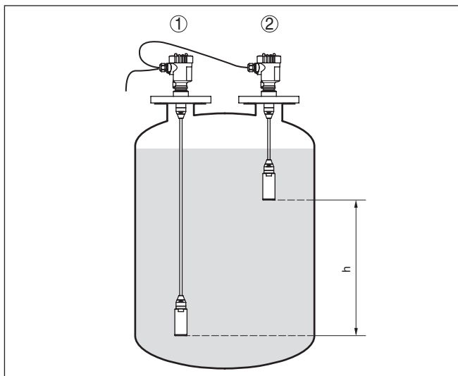
插图. 11: 测量密度层时的测量分布, h = 在两个测量点之间的距离
