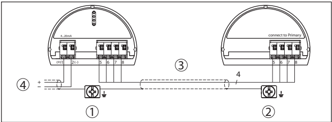
插图. 20: 电子差压的连接举例
