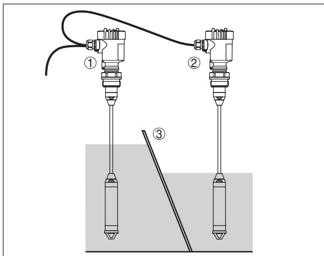
插图. 9: 进行水位差测量时的测量排布
