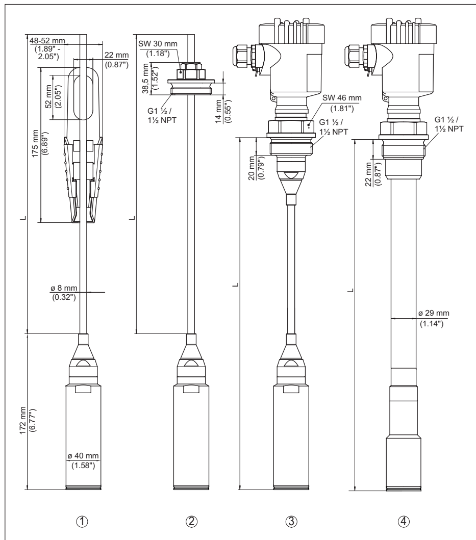
插图. 29: VEGABAR 87, 标准接头
