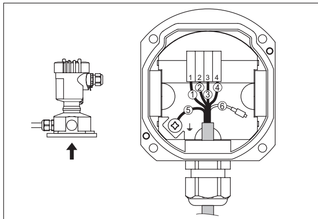
插图. 18: 壳体底座中过程组件的接口
