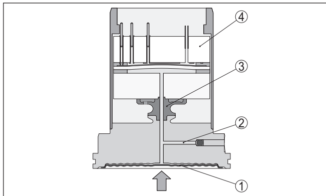
插图. 2: 在 VEGABAR 87 中 METEC® 测量元件的结构
