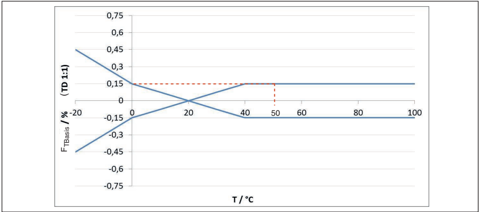
插图. 25: 为上例计算基本温度误差: F_{TBasis} = 0.15 \%
