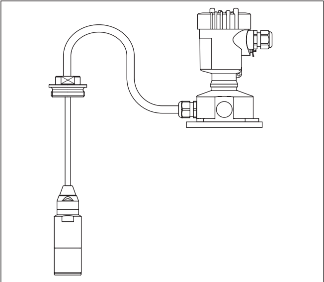
插图. 16: IP68 型 VEGABAR 87, 25 bar, 不能防爆, 轴向电缆出口, 外部壳体
