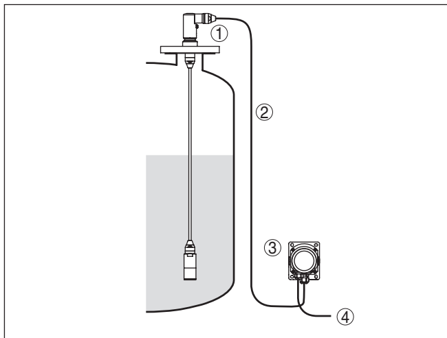
插图. 13: 测量点的分布, 外部壳体
