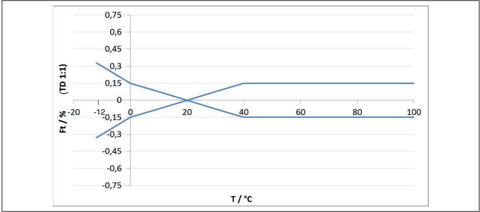
插图. 24: 基本温度错误 F_{T_{基本}} 当 TD 1 : 1 时
