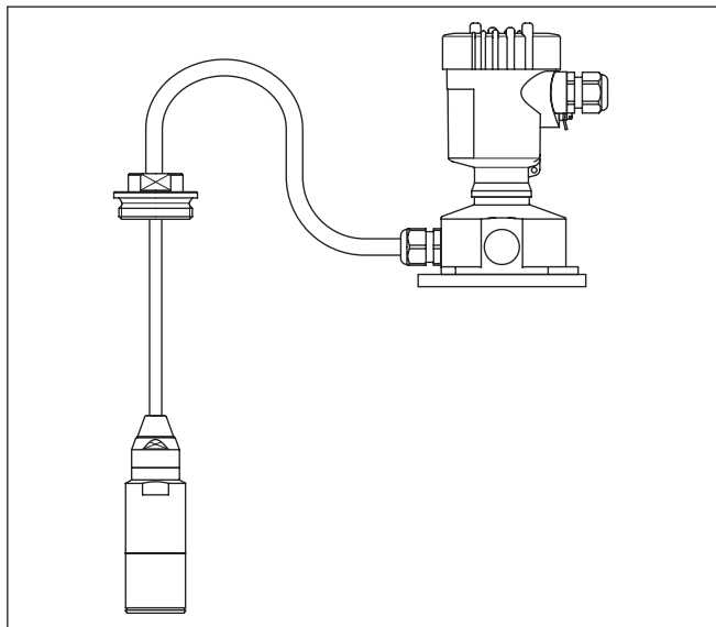
插图. 23: IP 68 型 VEGABAR 67 , 25 bar , 不能防爆 , 轴向电缆出口 , 外部壳体
