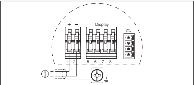
插图. 26: 外部电子部件的接线图
