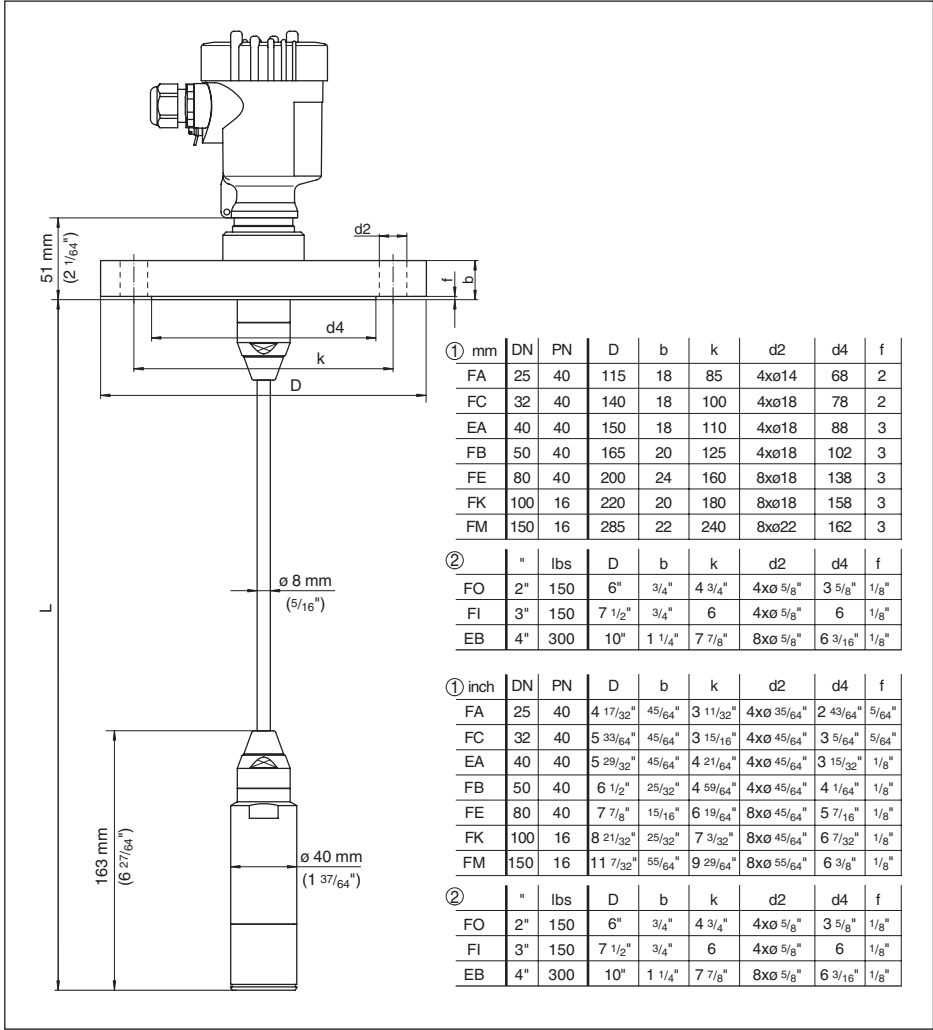
插图. 48: VEGABAR 67，法兰连接
