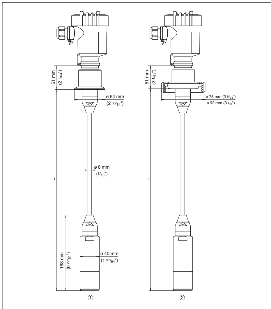
插图. 49: VEGABAR 67, 无菌连接
