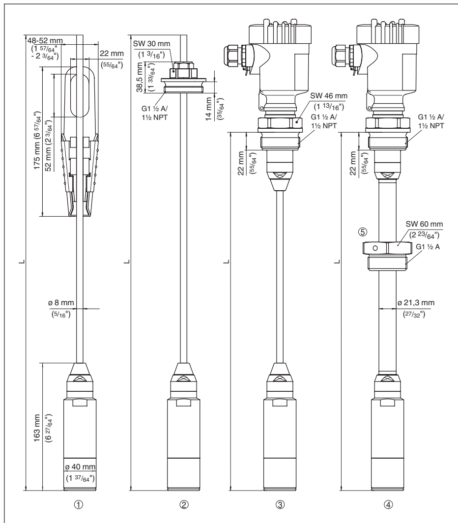
插图. 47: VEGABAR 67, 标准接头
