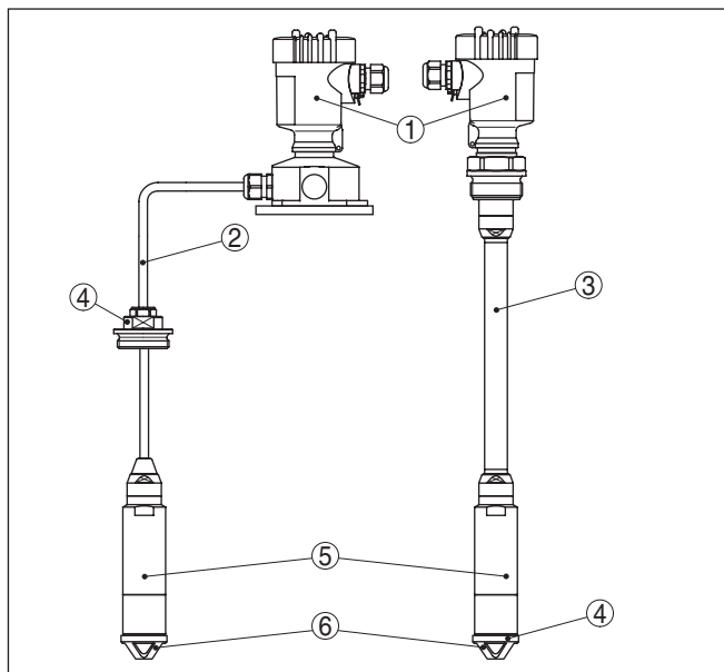
插图. 1: 举例说明一个VEGABAR 67, 带提携电缆 (左) 和连接管 (右)
