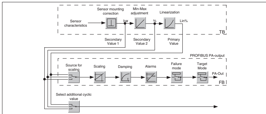
插图. 33: VEGABAR 67 : 带有 AI (PA-OUT) 值和附加循环值的框图
