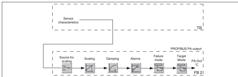
插图. 34: VEGABAR 67 : 带有温度值的框图
