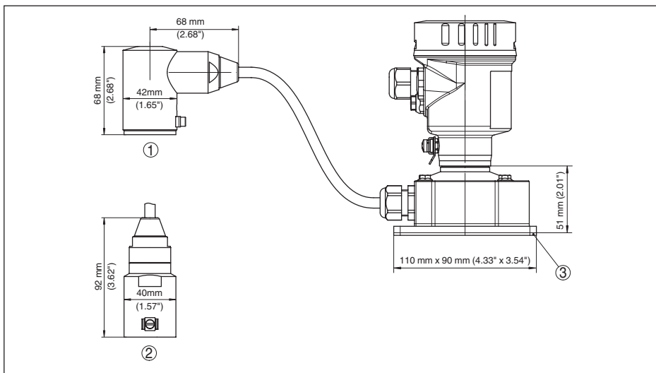
插图. 46: 外部壳体 - 不锈钢型
