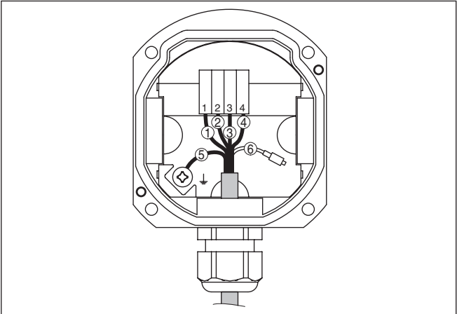
插图. 25: 传感器在壳体底座内的连接情况
