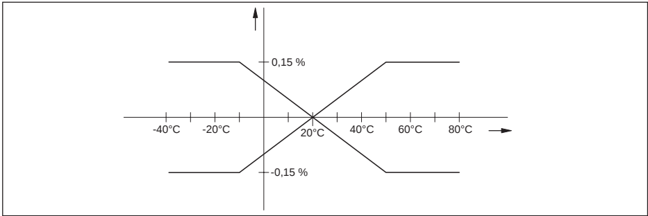
插图. 32: 电流输出的热变化
