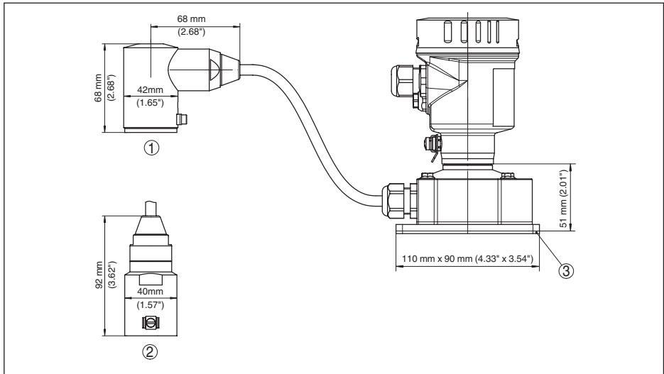
插图. 28: 外部壳体 - 不锈钢型
