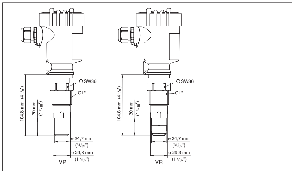
插图. 35: VEGABAR 54, 用于造纸的连接 : VP = G1" 用于 PASVE, VR = G1" 用于带 O 型密封圈的 PASVE
