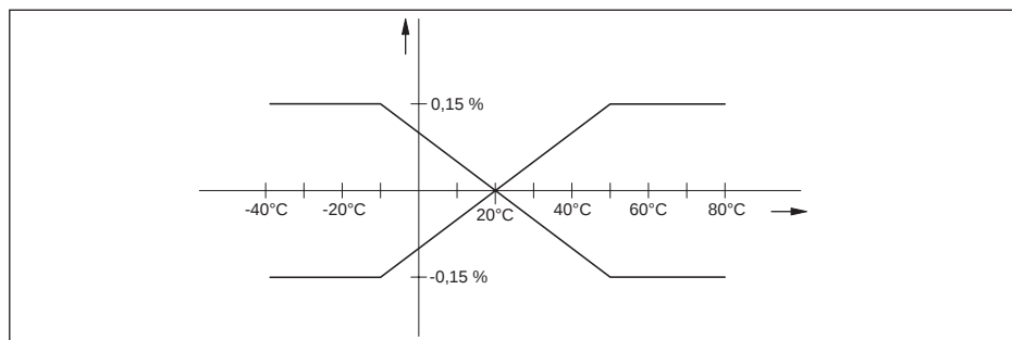
插图. 20: 电流输出的热变化
