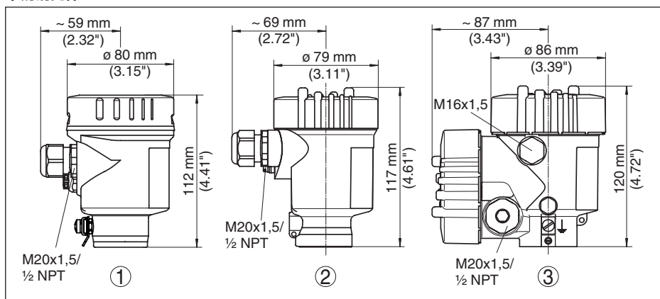
插图. 25: 采用保护方式为 IP 66/IP 68 (0.2 bar) 的外壳型式 - 内装显示和调整模块后，外壳高度增加了 9 mm/0.35 in
