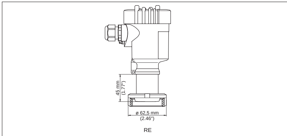
插图. 31: VEGABAR 54, 无菌连接 : RE = 管螺纹接头 DN 25 PN 40 符合 DIN 11851
