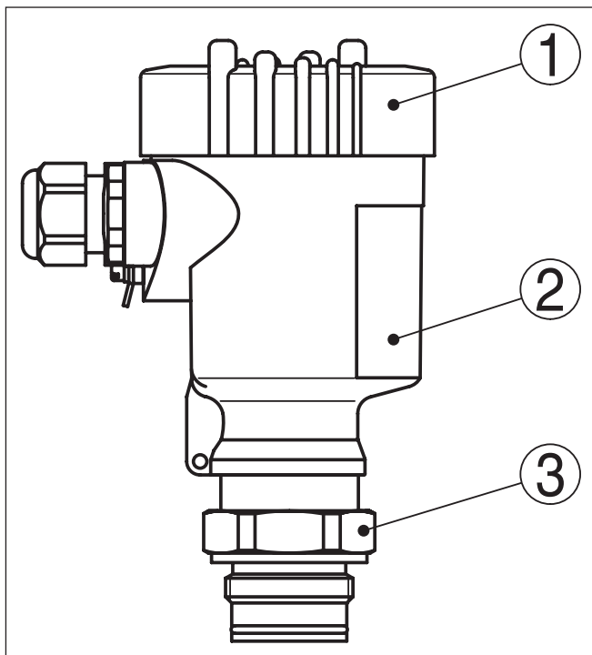
插图. 1: 举例说明一个带有过程接头 G1 A 和塑料壳体的 VEGABAR 54
