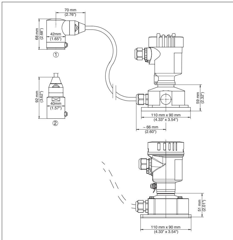
插图. 27: 带有外部壳体的 IP 68 型 - 塑料型
