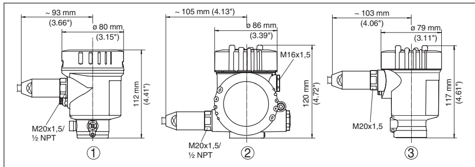
插图. 26: 采用保护方式为 IP 66/IP 68 (1 bar) 的外壳型式 - 内装显示和调整模块后，外壳高度增加了 9 mm/0.35 in
