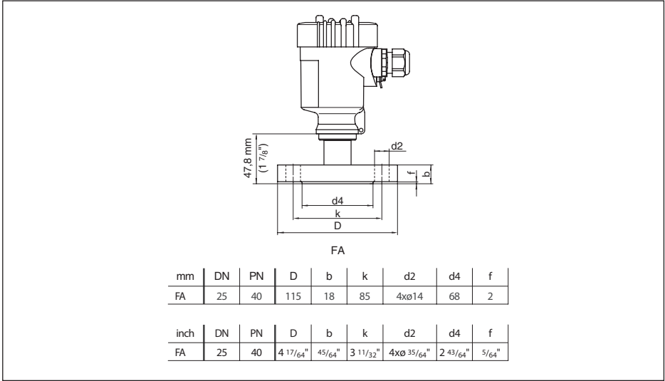
插图. 33: VEGABAR 54, B1 法兰连接, EN 1092-1
