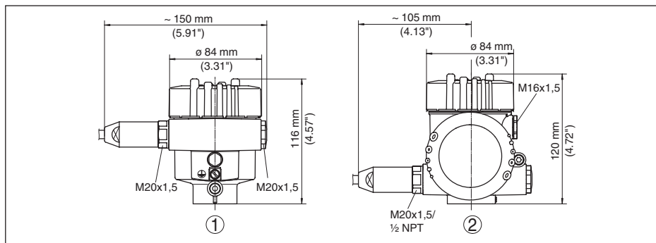
插图. 24: 采用保护方式为 IP 66/IP 68 (1 bar) 的外壳型式 - 内装显示和调整模块后，外壳高度增加了 9 mm/0.35 in
