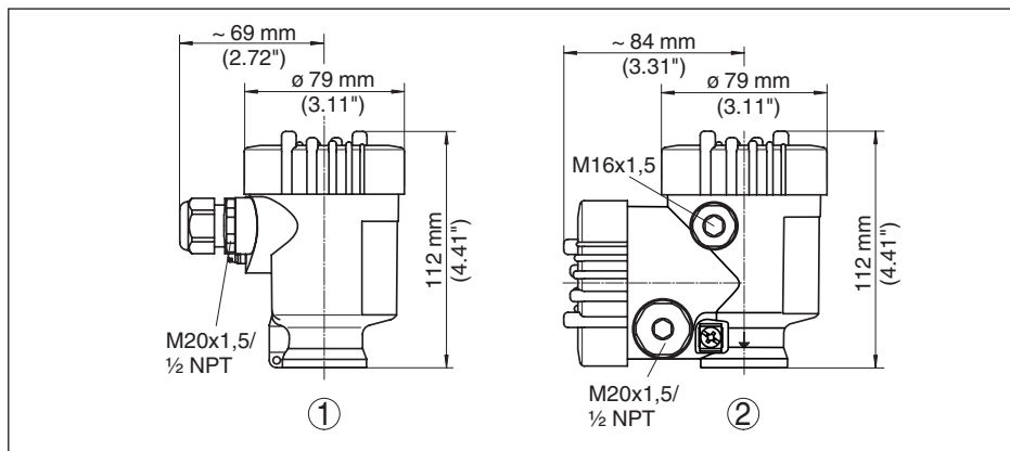
插图. 22: 采用保护方式为 IP 66/IP 68 (0.2 bar) 的外壳型式 - 内装显示和调整模块后，外壳高度增加了 9 mm/0.35 in
