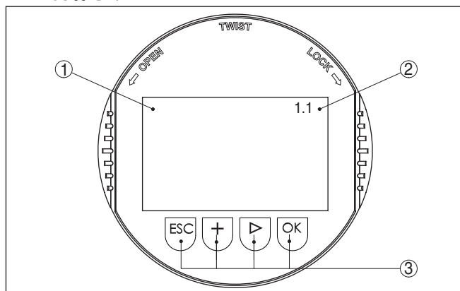
插图. 18: 显示和调整元件
