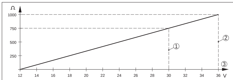
插图. 21: 供电电压图
