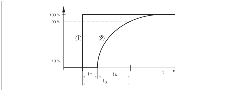
插图. 19: 过程值的跳跃式更改。t T : 死亡时间；t A : 上升时间；t S : 跳跃式回应时间
