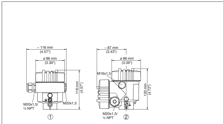
插图. 23: 采用保护方式为 IP 66/IP 68 (0.2 bar) 的外壳型式 - 内装显示和调整模块后，外壳高度增加了 9 mm/0.35 in
