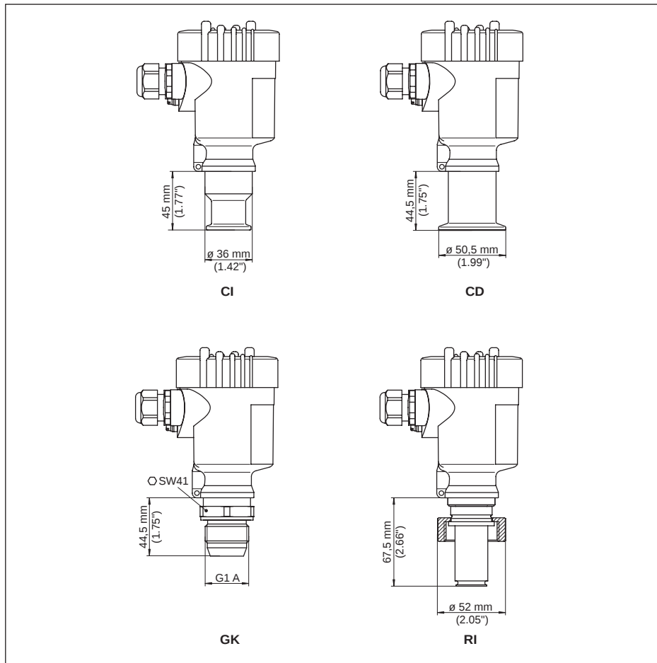
插图. 30: VEGABAR 54 , 无菌接头 : CI = 卡箍 DN15-20 符合 DIN 32676, CD = 卡箍 1" 符合 DIN 32676, ISO 2852, GK = G1 A 锥形 40° 与前壁齐平 , RI = Ingold 连接
