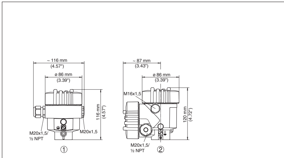
插图. 36: 采用保护方式为 IP 66/IP 68 (0.2 bar) 的外壳型式 - 内装显示和调整模块后, 外壳高度增加了 9 mm/0.35 in
