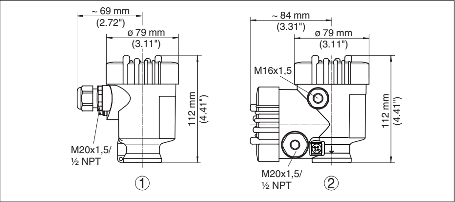
插图. 35: 采用保护方式为 IP 66/IP 68 (0.2 bar) 的外壳型式 - 内装显示和调整模块后，外壳高度增加了 9 mm/0.35 in 1 单腔型式 2 两腔型式
