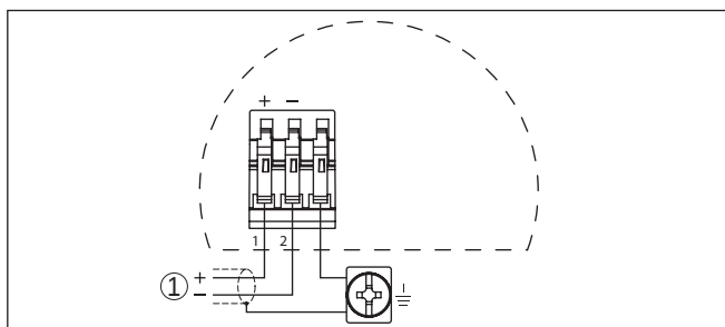
插图. 16: 防爆 (d) 型两腔式外壳的接线图
