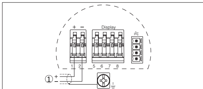
插图. 10: 单腔式外壳接线图
