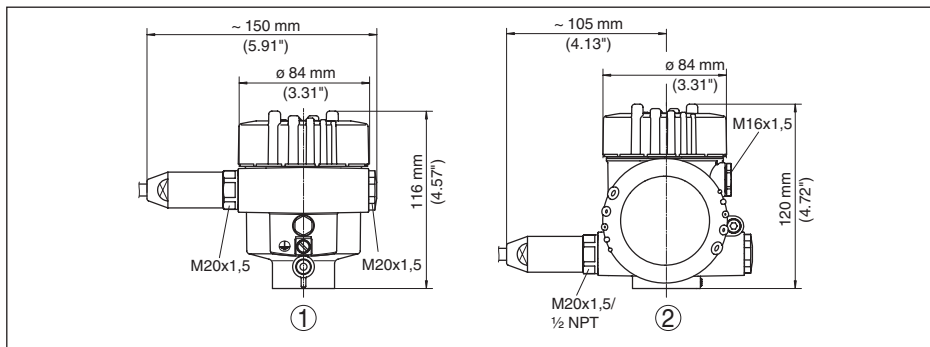
插图. 37: 采用保护方式为 IP 66/IP 68 (1 bar) 的外壳型式 - 内装显示和调整模块后, 外壳高度增加了 9 mm/0.35 in
