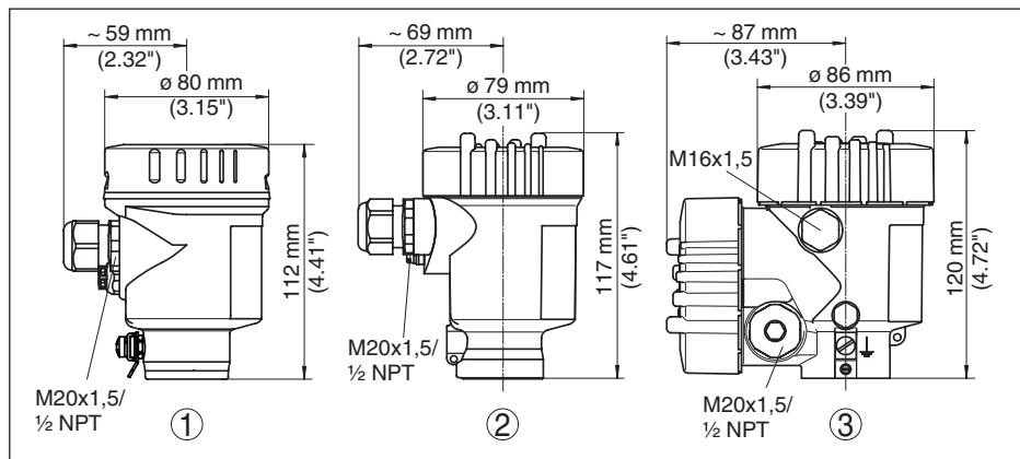
插图. 38: 采用保护方式为 IP 66/IP 68 (0.2 bar) 的外壳型式 - 内装显示和调整模块后, 外壳高度增加了 9 mm/0.35 in
