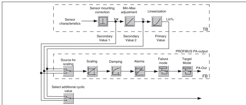
插图. 28: VEGABAR 52 : 带有 AI (PA-OUT) 值和附加循环值的框图
