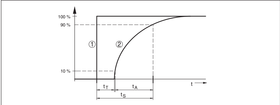
插图. 26: 过程值的跳跃式更改。 t_T : 死亡时间; t_A : 上升时间; t_S : 跳跃式回应时间
