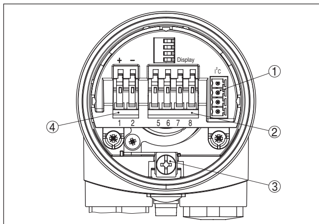
插图. 9: 采用单腔式外壳时的电子部件和接线腔
