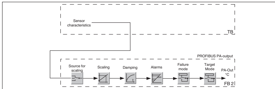
插图. 29: VEGABAR 52 : 带有温度值的框图
