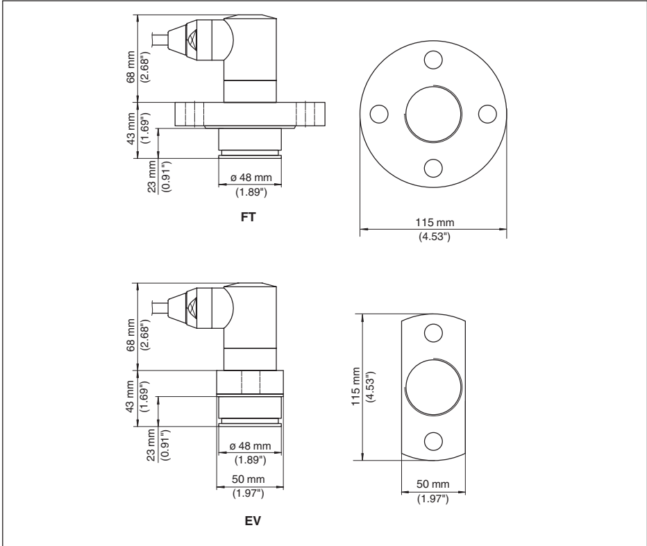
插图. 49: VEGABAR 52, 用于造纸工业的法兰连接 : FT = 绝对与前壁齐平, 用于造纸机, EV = 绝对与前壁齐平, 用于造纸机 (两侧铣平了的法兰)
