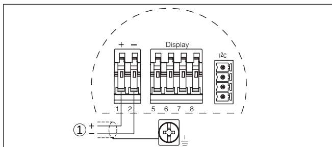
插图. 21: 外部电子部件的接线图
