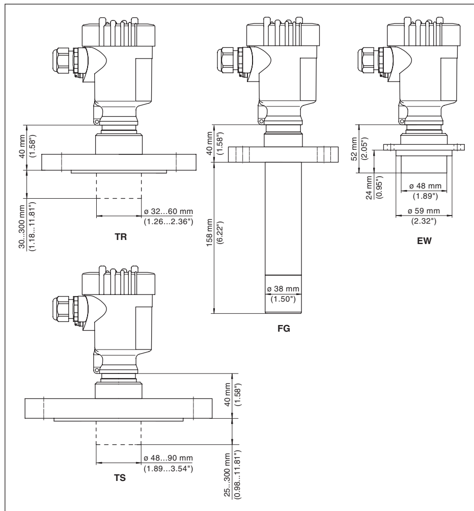
插图. 48: VEGABAR 52, 用于造纸工业的法兰连接 : TR = 法兰 DN 50 带可选的管, TS = 法兰 DN 80 带可选的管, FG = 用于球阀配件的法兰管, EW = 用于压力计视孔的法兰
