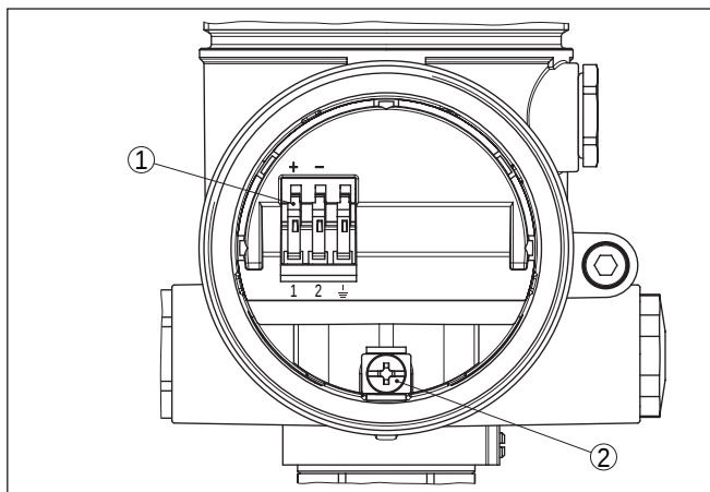
插图. 15: 防爆 (d) 型两腔式外壳的接线腔
