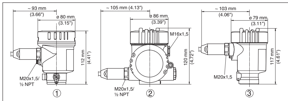
插图. 39: 采用保护方式为 IP 66/IP 68 (1 bar) 的外壳型式 - 内装显示和调整模块后, 外壳高度增加了 9 mm/0.35 in
