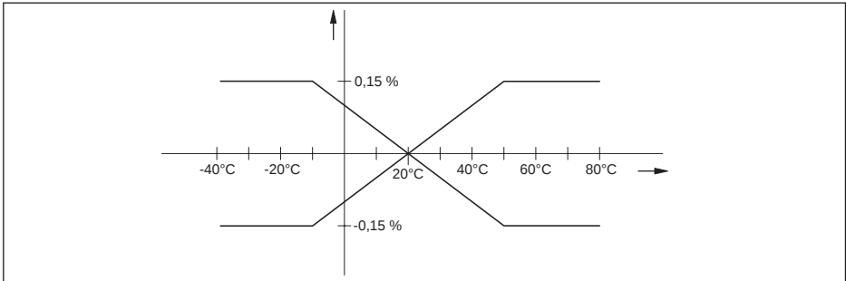
插图. 27: 电流输出的热变化
